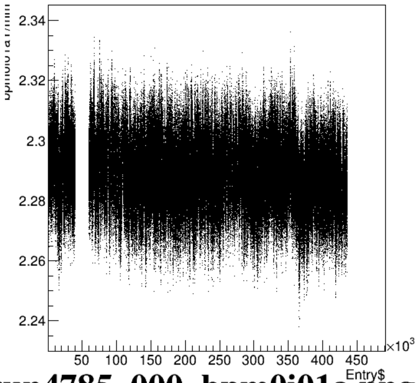
bpm0i01aY/mm:Entry$ {ErrorFlag==0}
