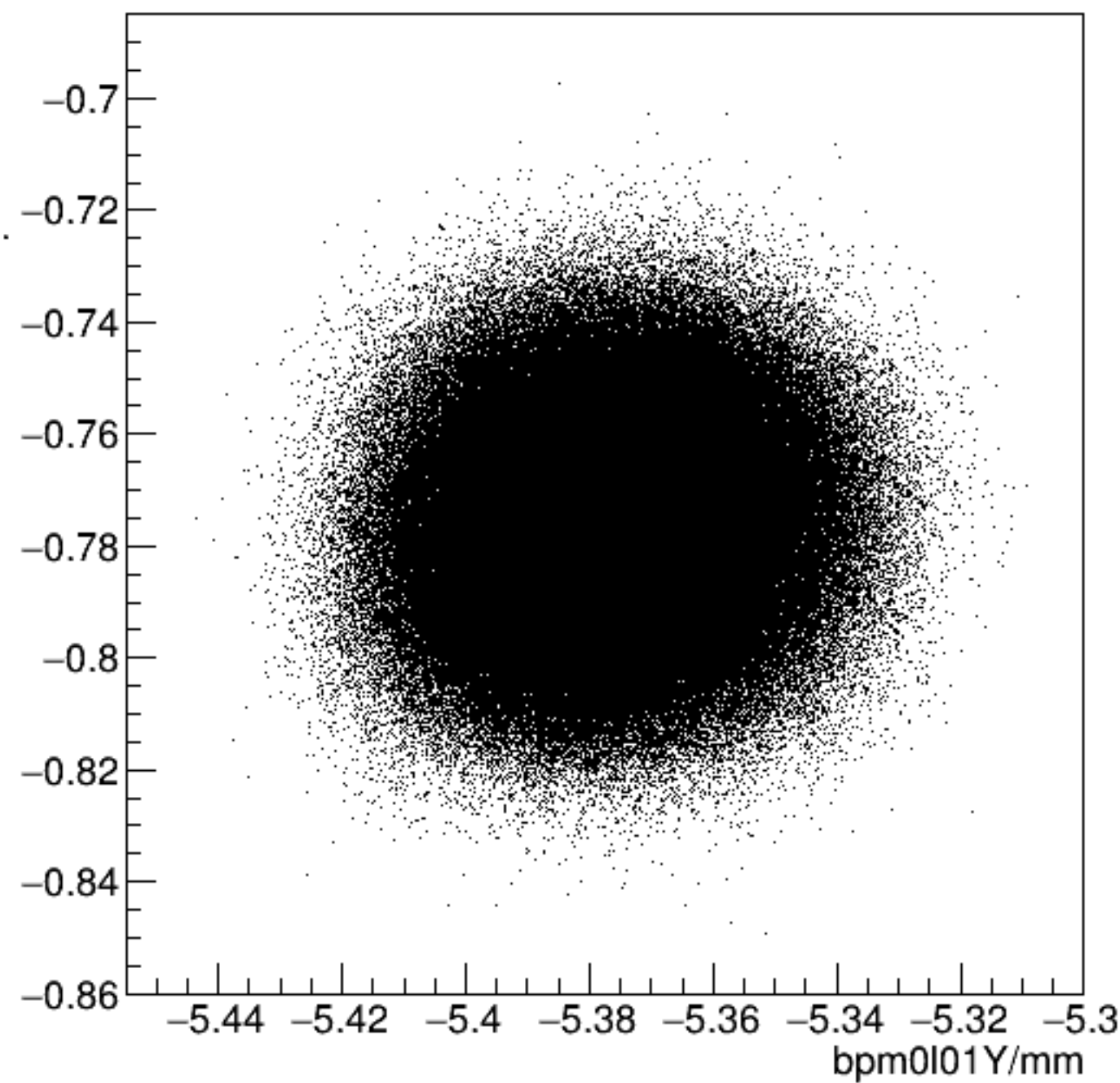
bpm0l01X/mm:bpm0l01Y/mm {ErrorFlag==0}
