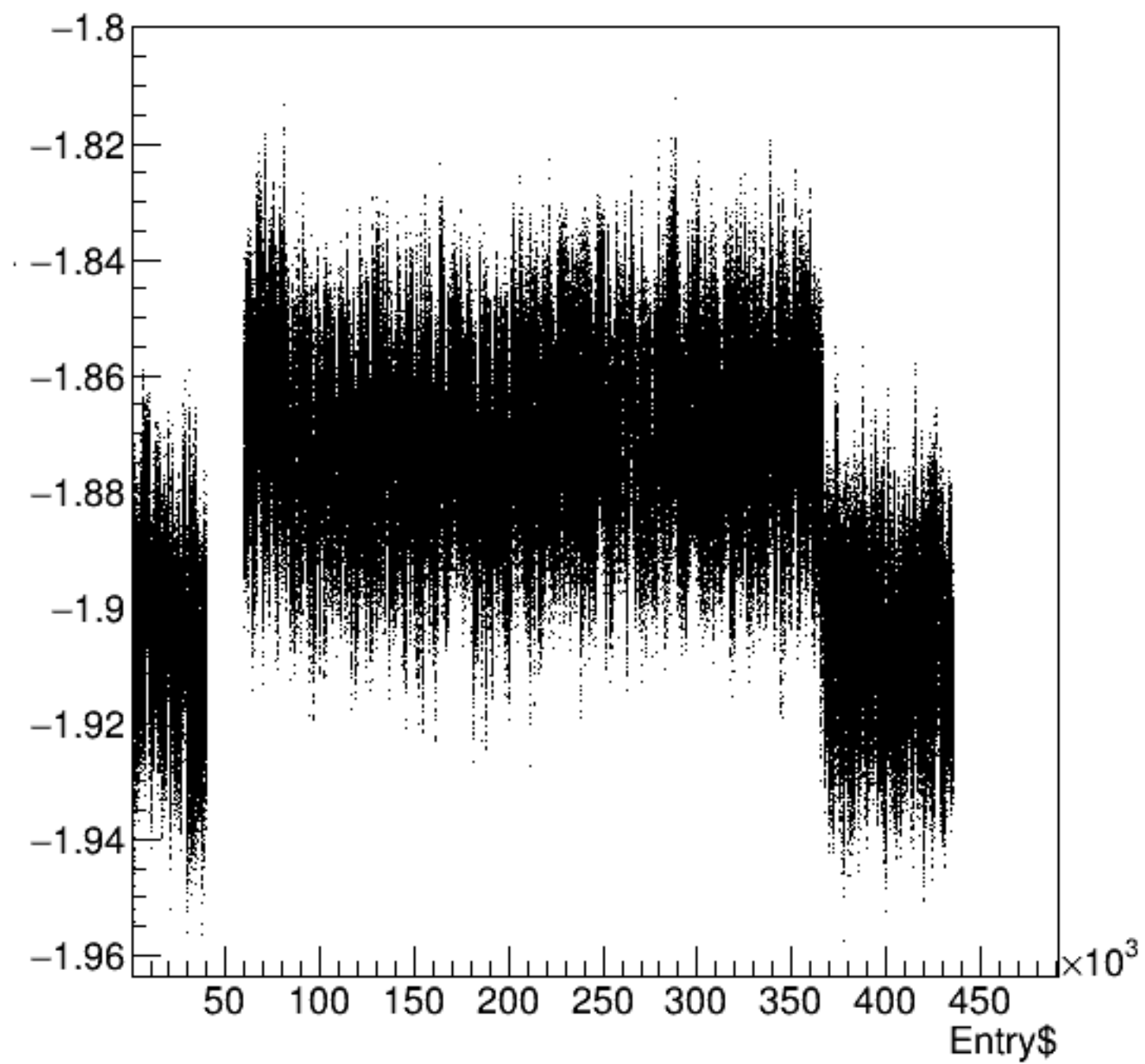
bpm0i01aX/mm:Entry$ {ErrorFlag==0}
