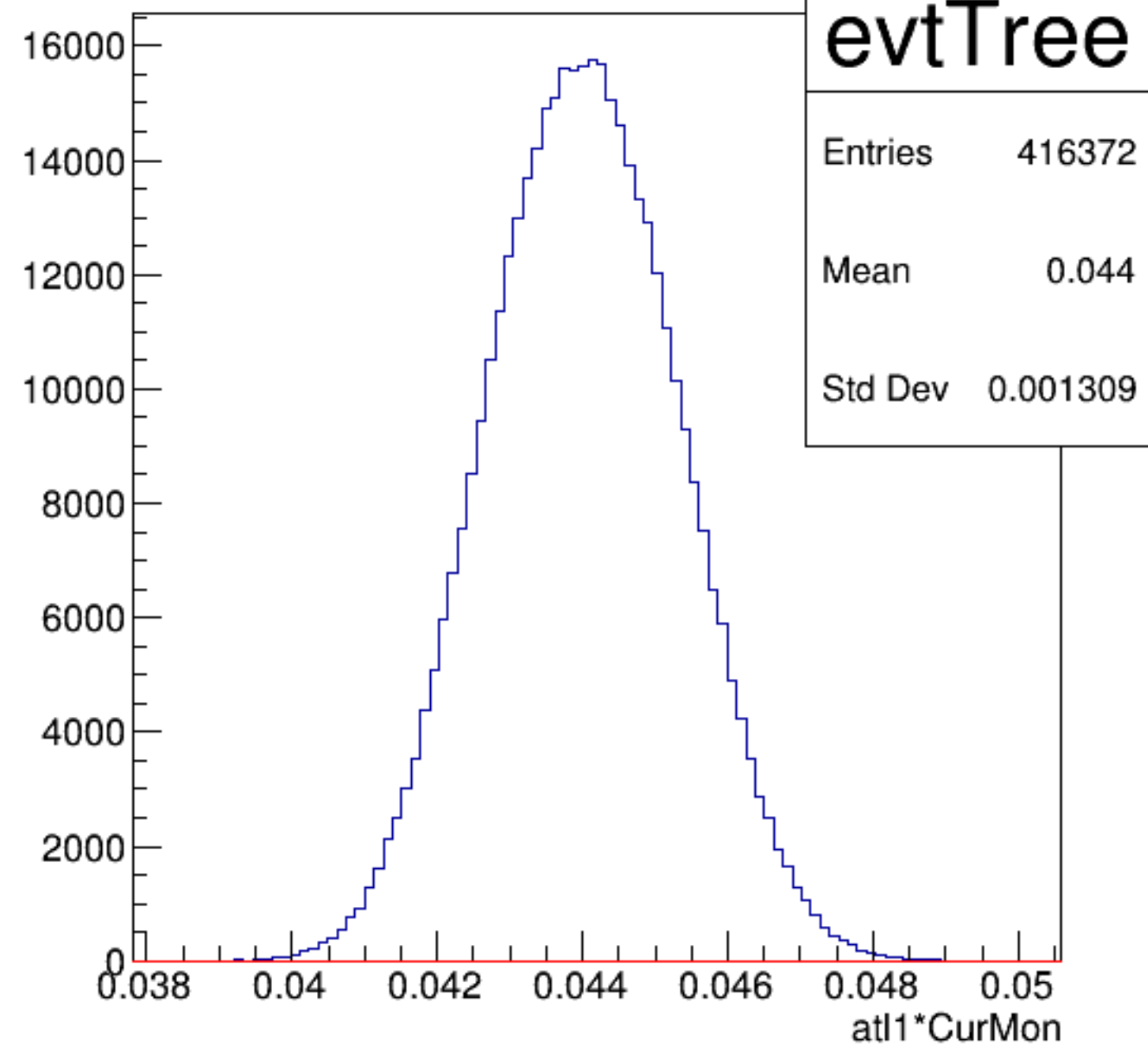
at1*CurMon {ErrorFlag==0}
