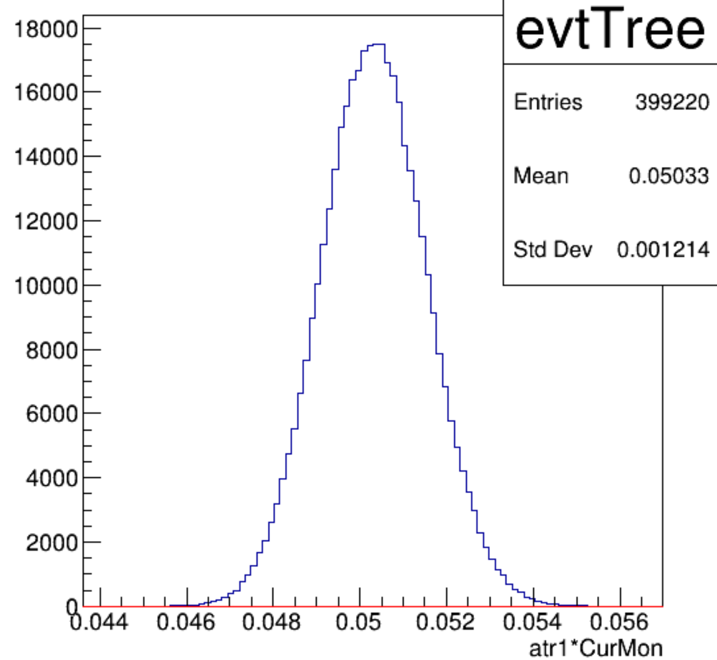
atr1*CurMon {ErrorFlag==0}
