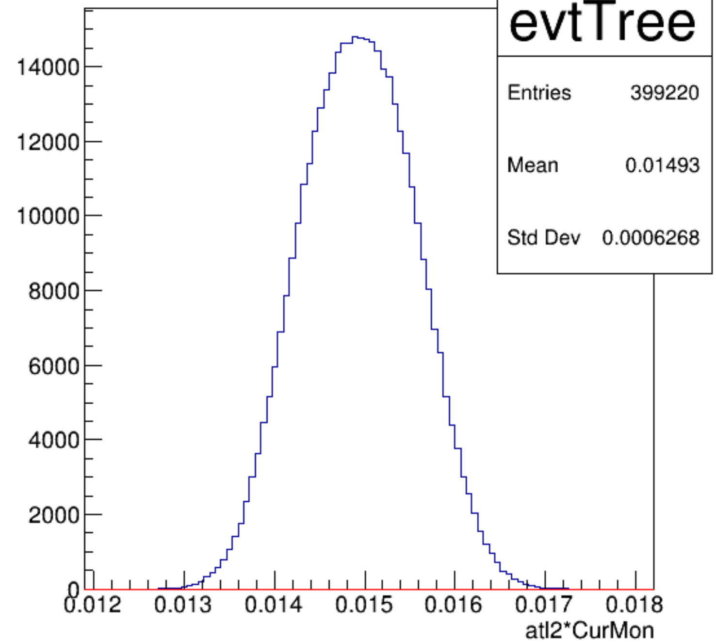
atl2*CurMon {ErrorFlag==0}
