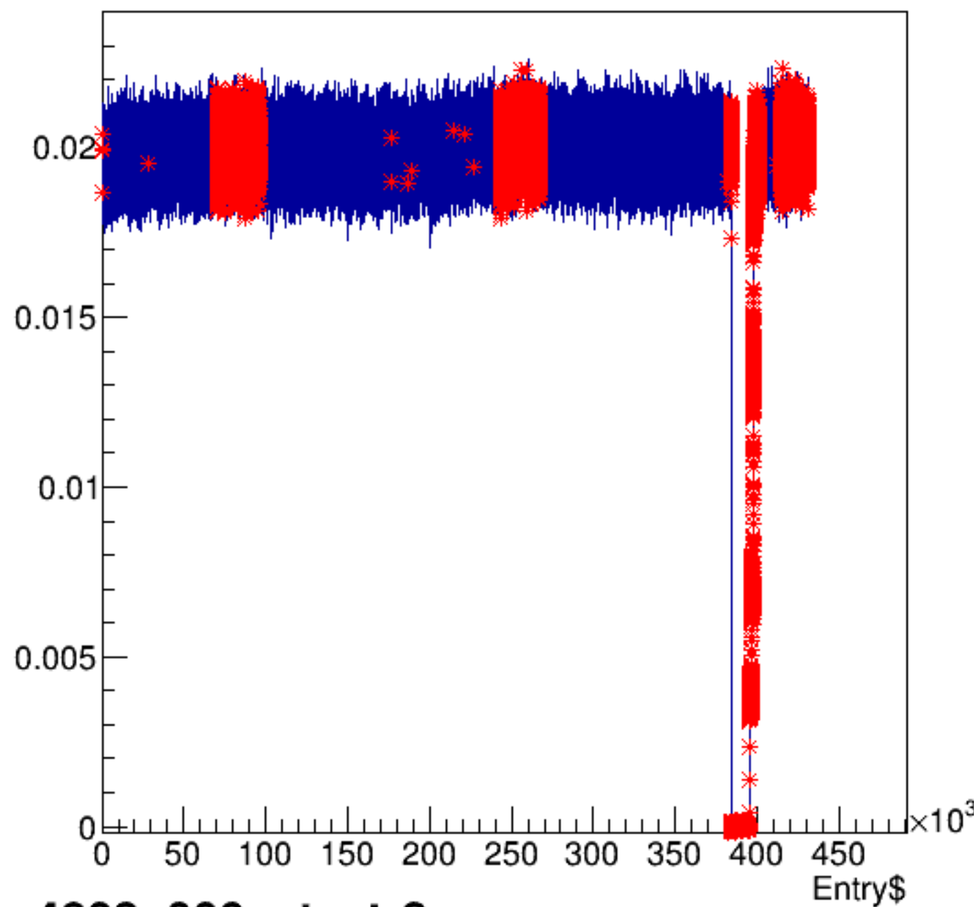
atr2*CurMon:Entry$
