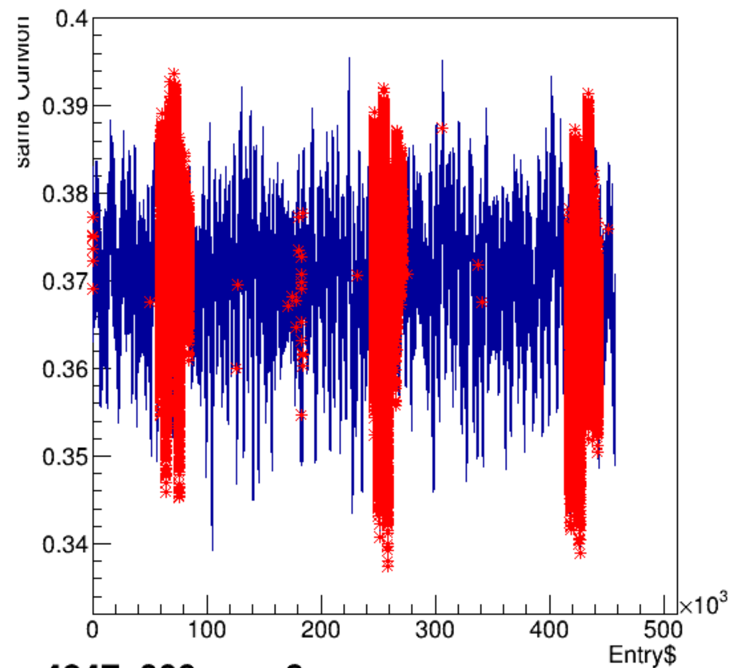
sam8*CurMon:Entry$
