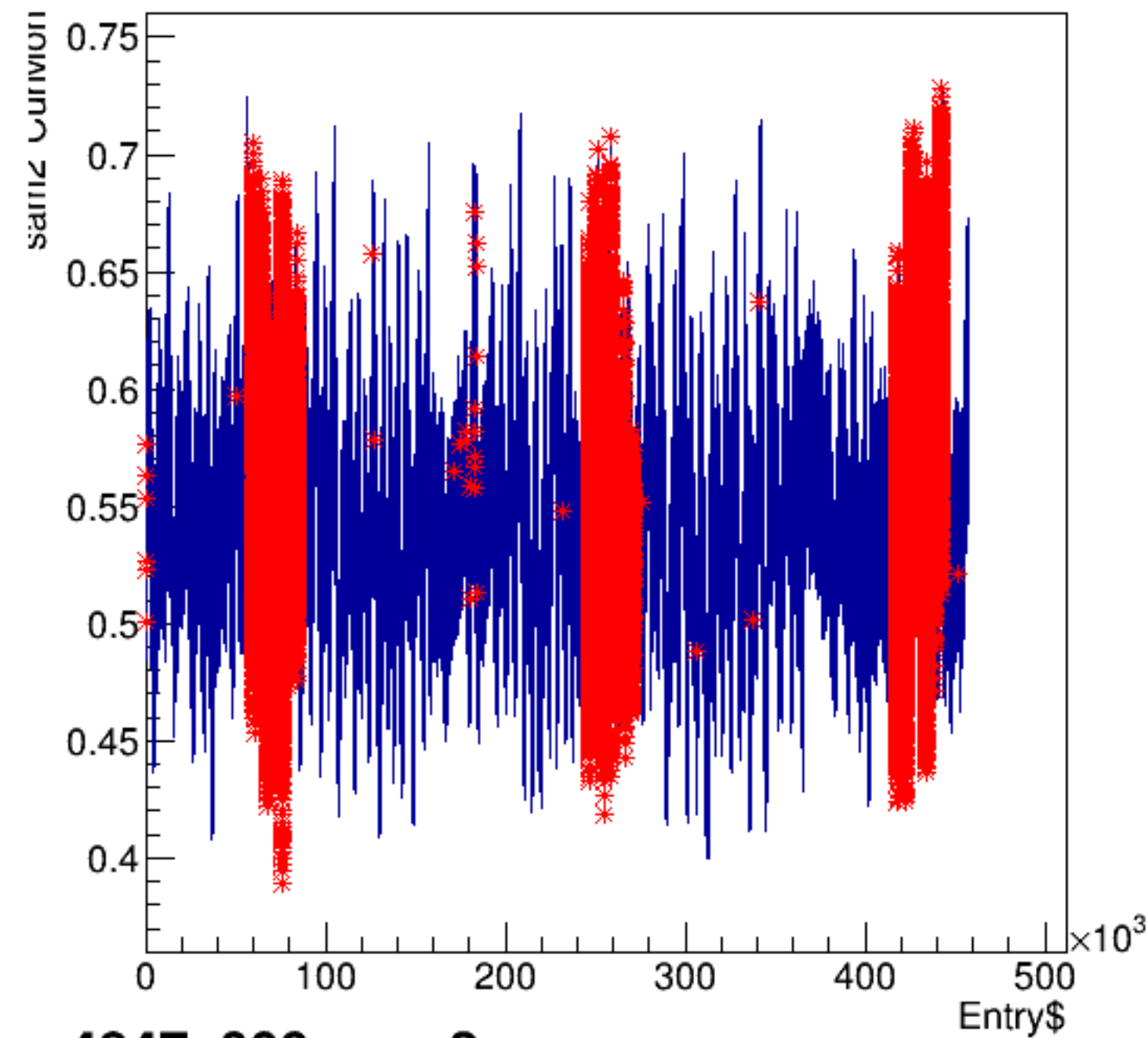
sam2*CurMon:Entry$
