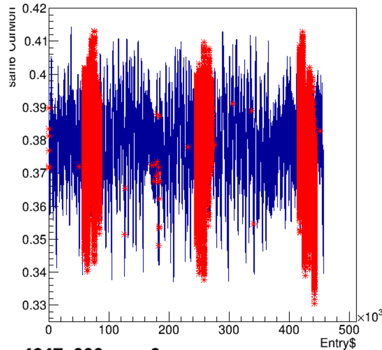
sam6*CurMon:Entry$
