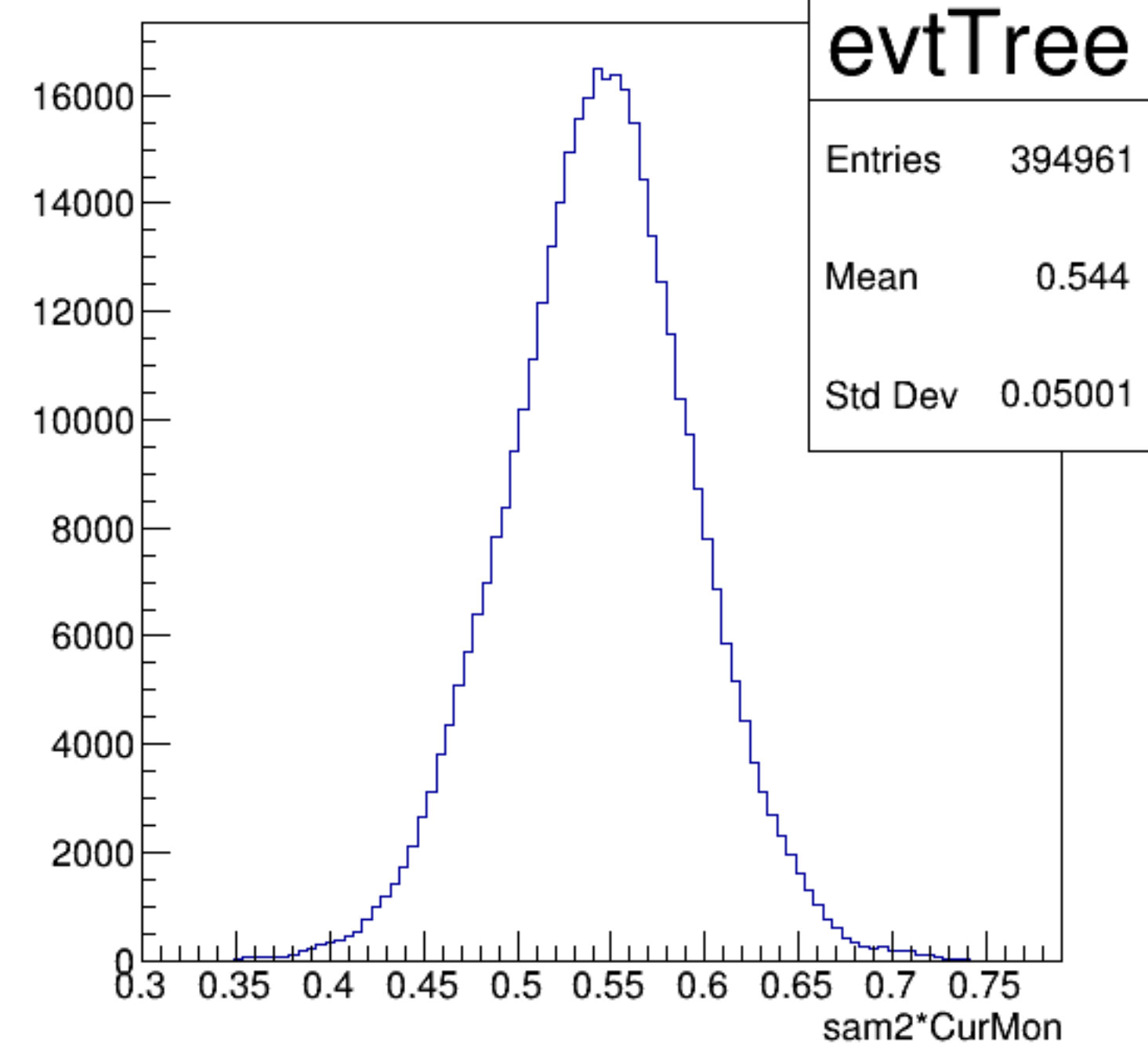
sam2*CurMon {ErrorFlag==0}
