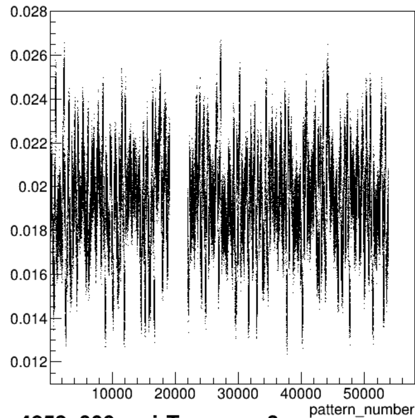
yield_sam3:pattern_number {ErrorFlag==0}
