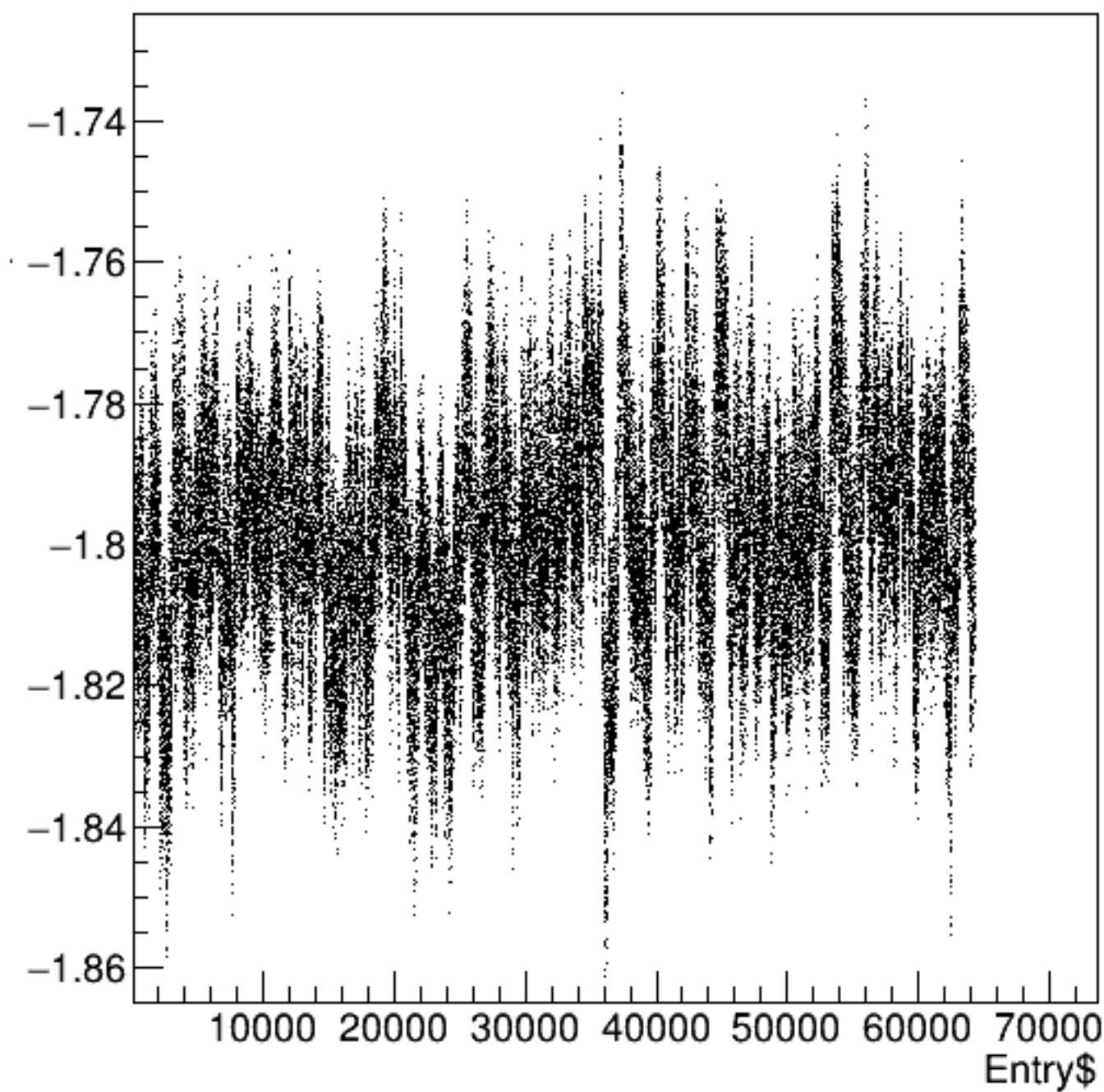
bpm0i01aX/mm:Entry$ {ErrorFlag==0}
