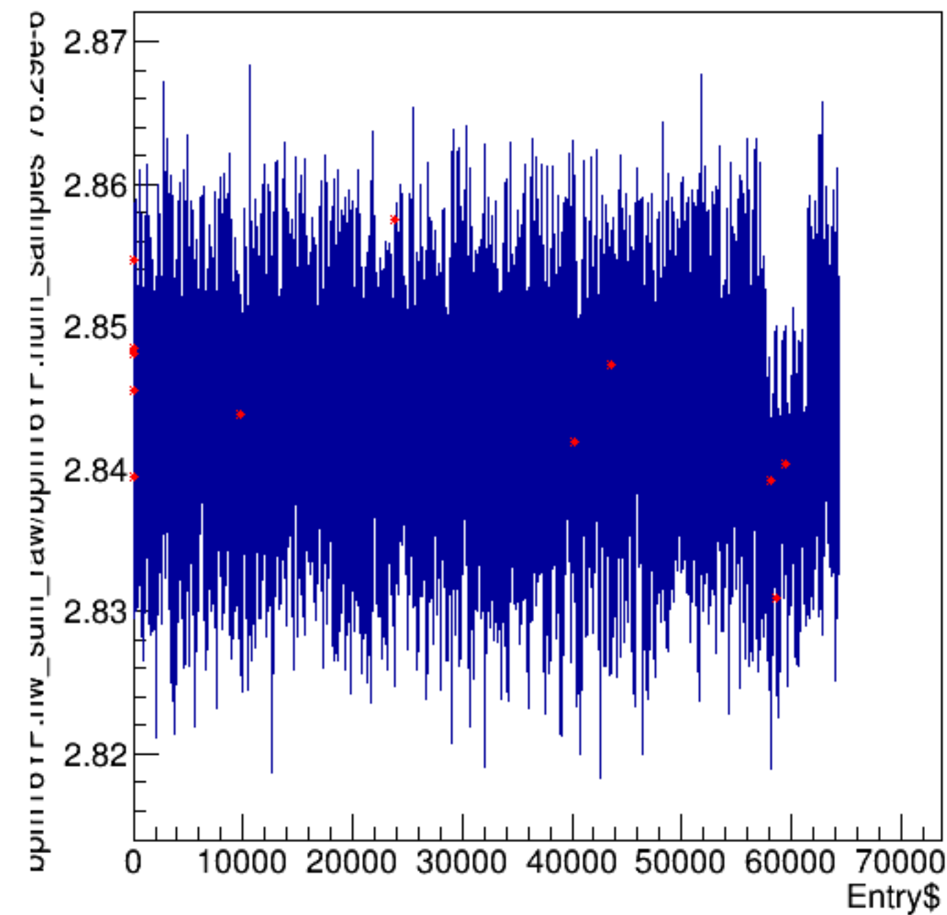
bpm16YP.hw_sum_raw/bpm16YP.num_samples*76.29e-6:Entry$
