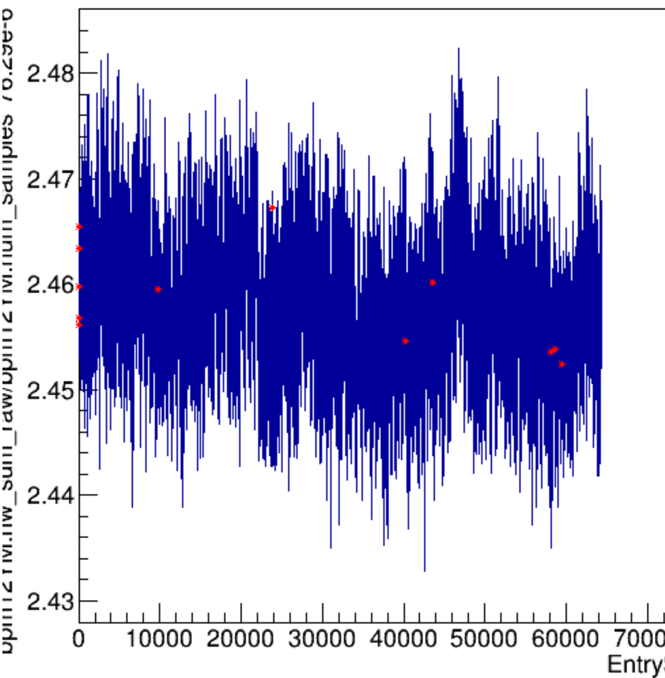
bpm12YM.hw_sum_raw/bpm12YM.num_samples*76.29e-6:Entry$
