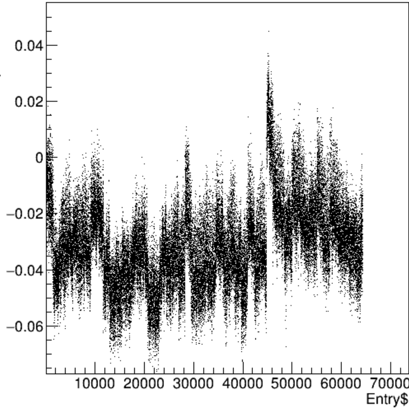
bpm4aX/mm:Entry$ {ErrorFlag==0}
