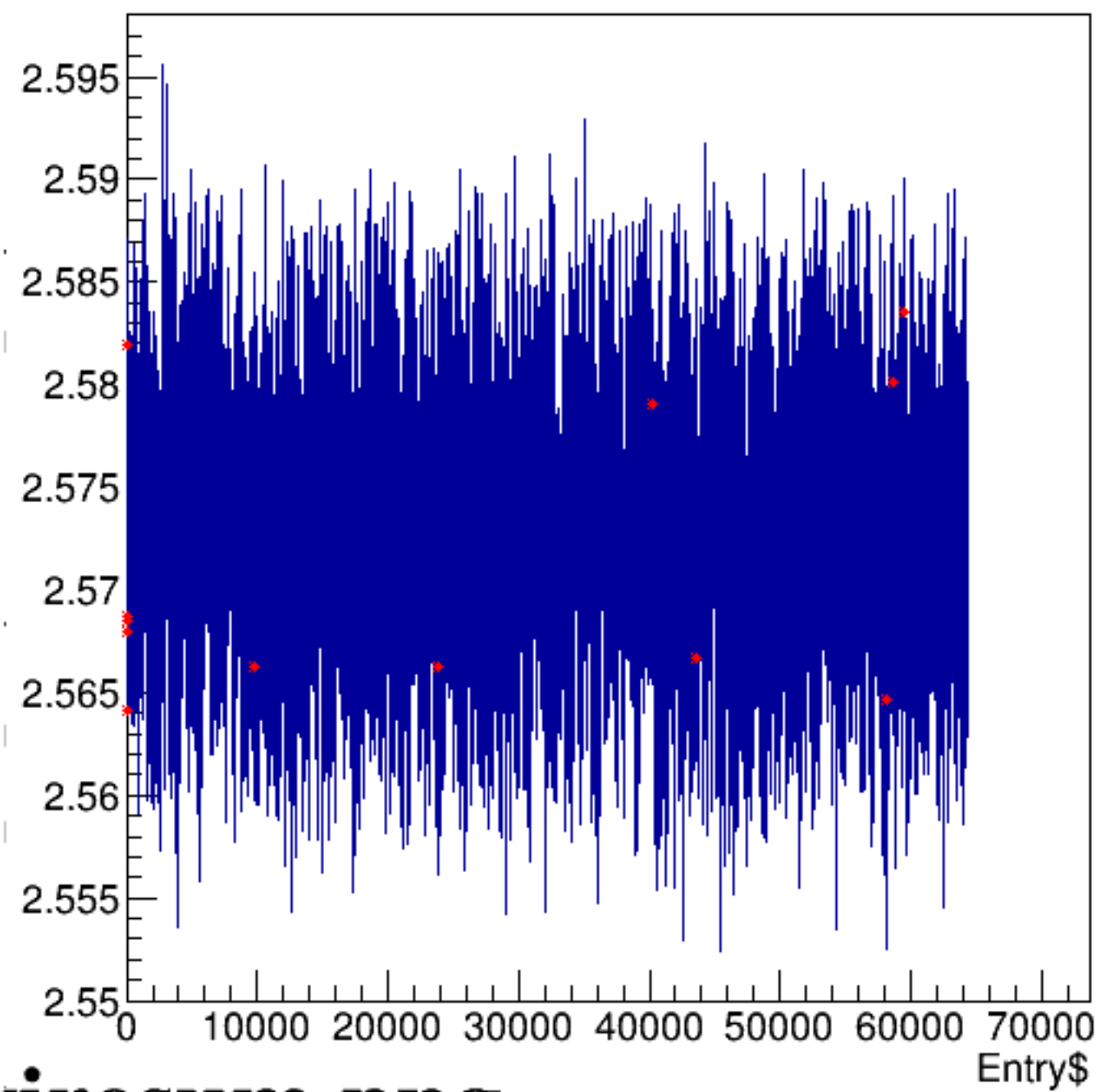
bpm2i01XM.hw_sum_raw/bpm2i01XM.num_samples*76.29e-6:Entry$
