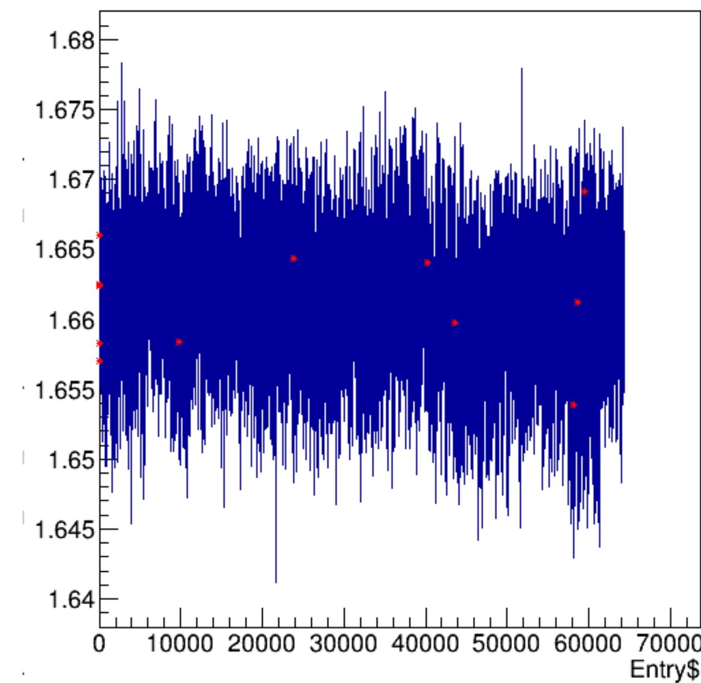
bpm0l01YP.hw_sum_raw/bpm0l01YP.num_samples*76.29e-6:Entry$
