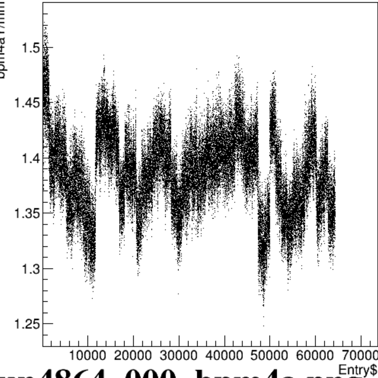
bpm4aY/mm:Entry$ {ErrorFlag==0}
