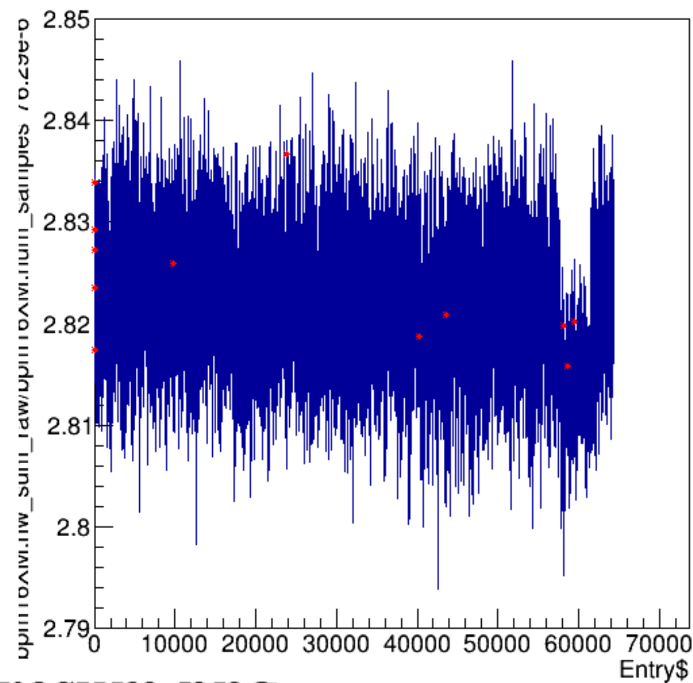
bpm16XM.hw_sum_raw/bpm16XM.num_samples*76.29e-6:Entry$
