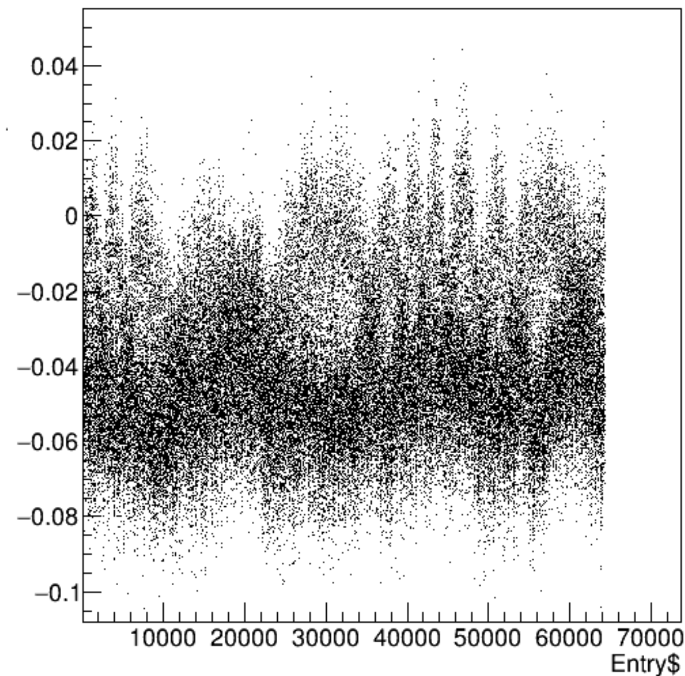
bpm16X/mm:Entry$ {ErrorFlag==0}
