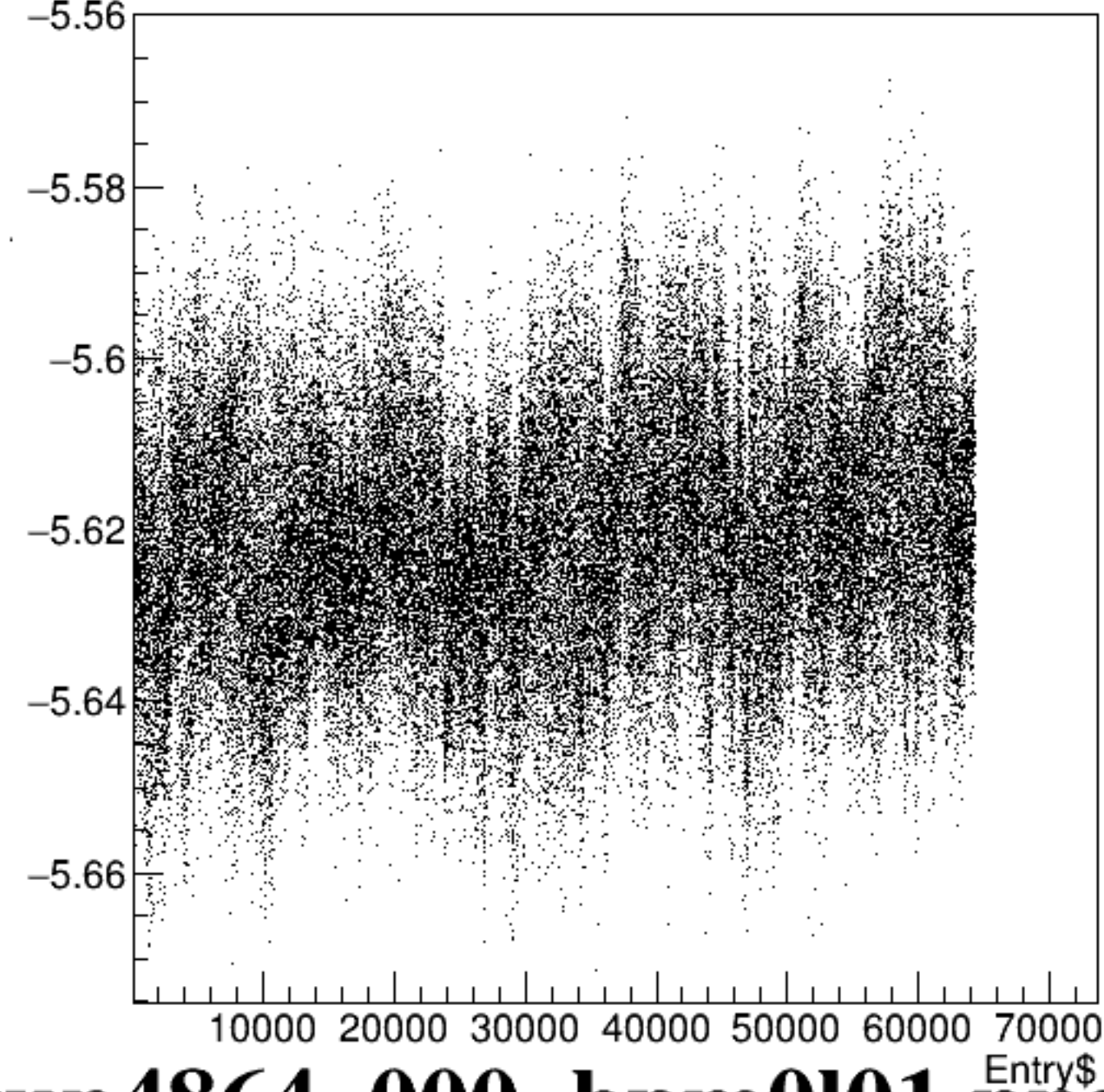
bpm0l01Y/mm:Entry$ {ErrorFlag==0}
