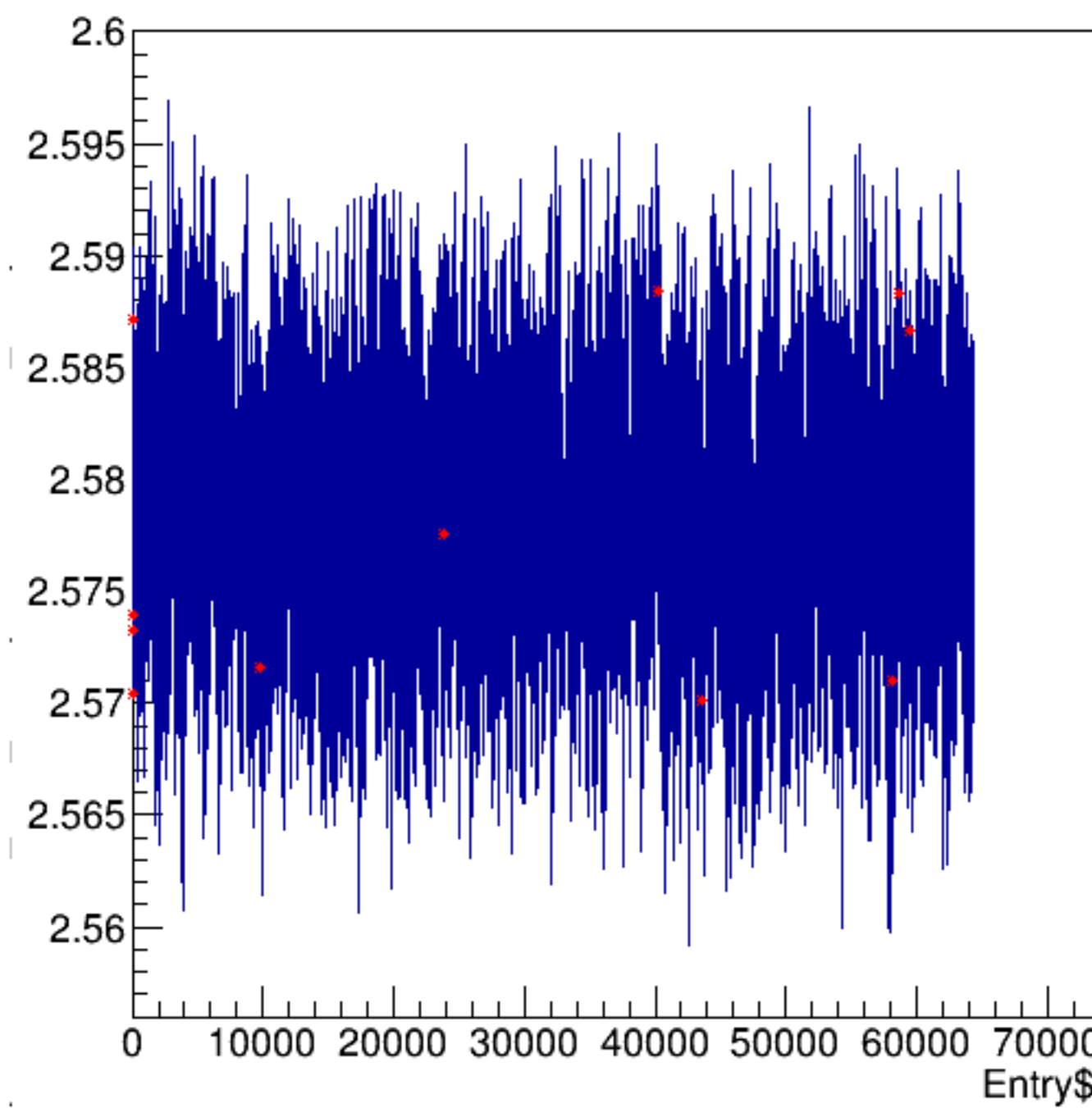
bpm2i01YM.hw_sum_raw/bpm2i01YM.num_samples*76.29e-6:Entry$
