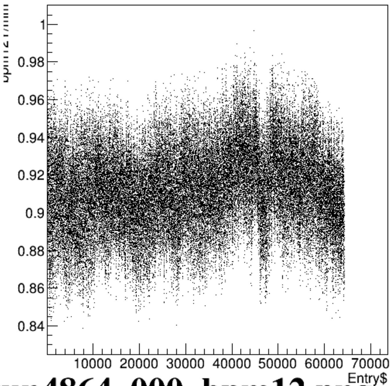
bpm12Y/mm:Entry$ {ErrorFlag==0}
