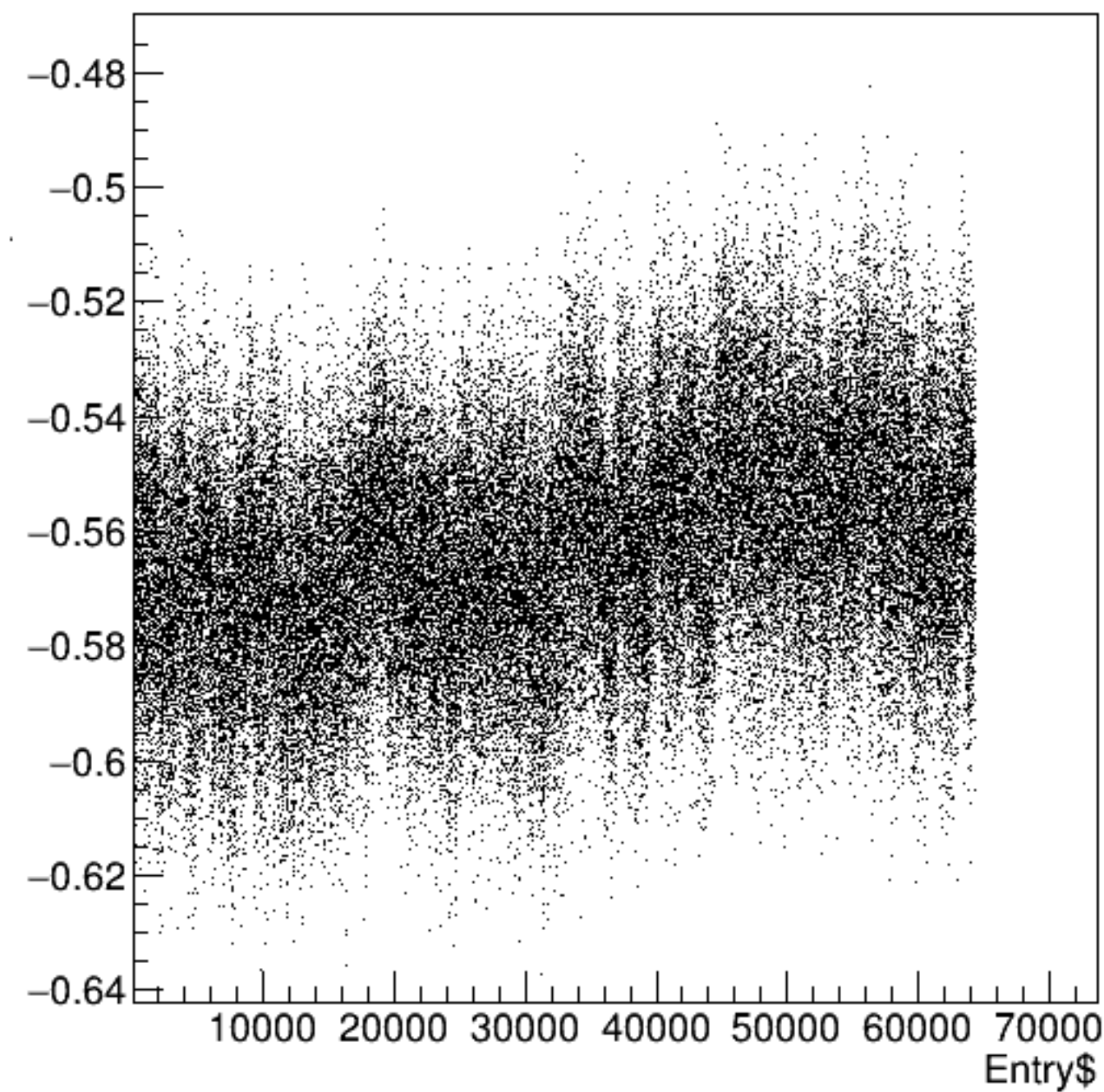
bpm0l01X/mm:Entry$ {ErrorFlag==0}
