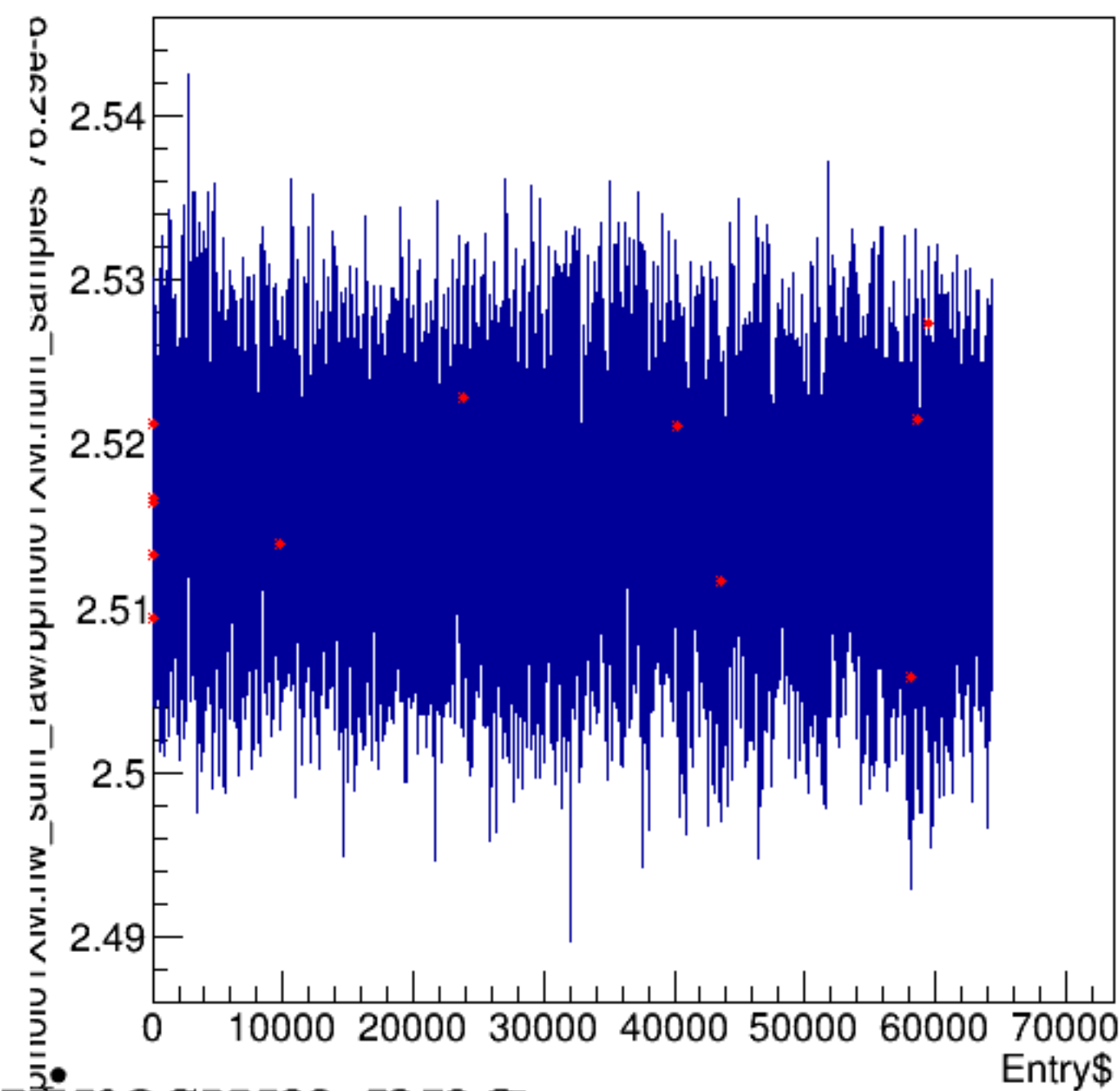
bpm0l01XM.hw_sum_raw/bpm0l01XM.num_samples*76.29e-6:Entry$
