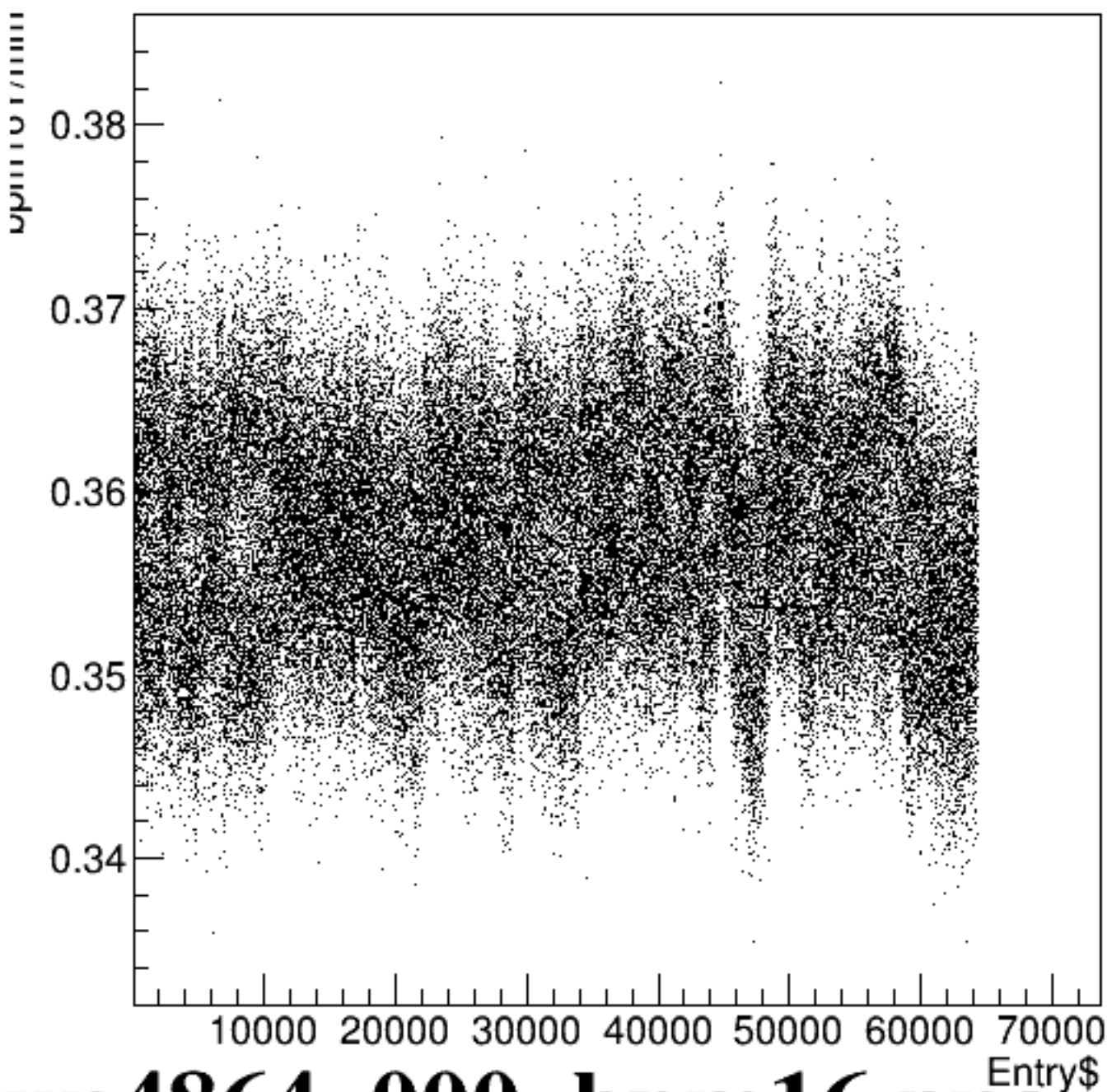
bpm16Y/mm:Entry$ {ErrorFlag==0}
