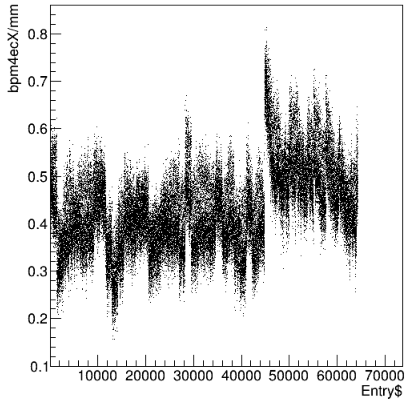
bpm4ecX/mm:Entry$ {ErrorFlag==0}
