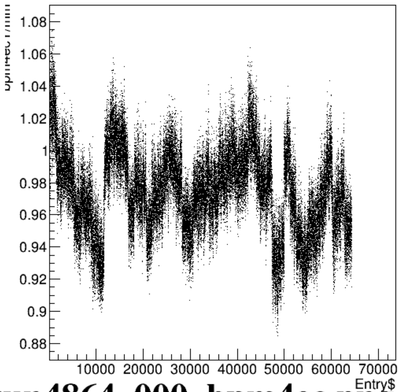
bpm4ecY/mm:Entry$ {ErrorFlag==0}
