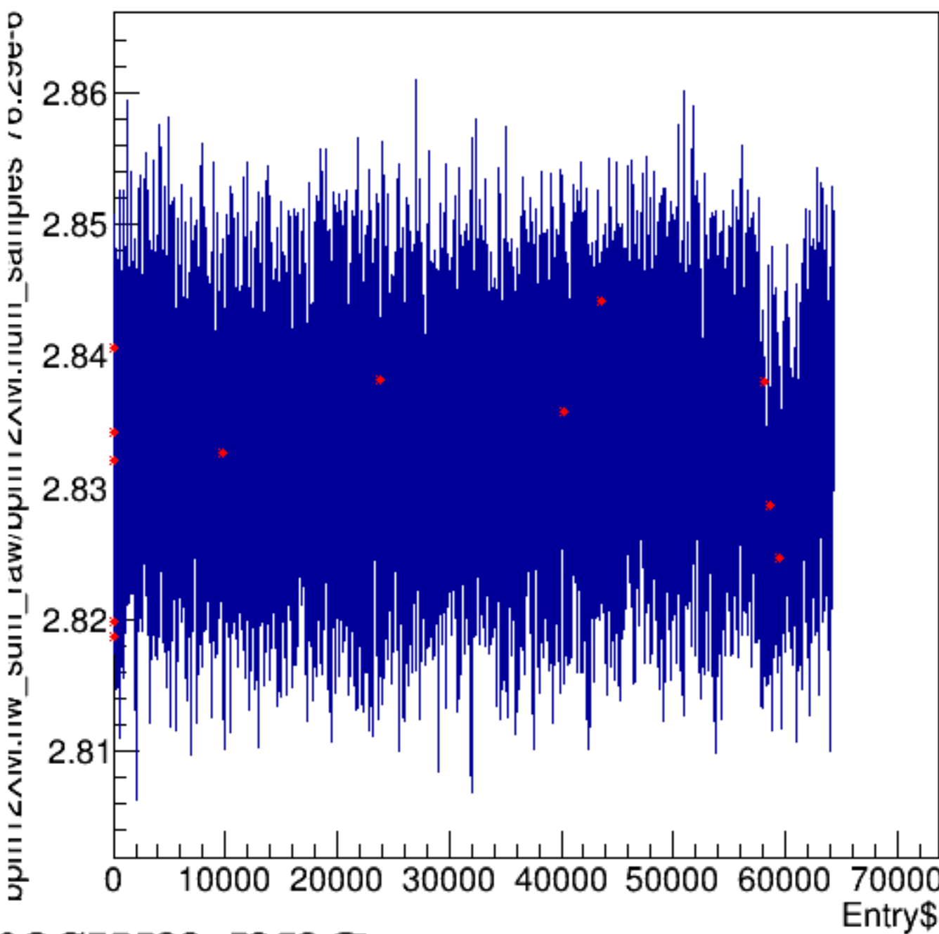
bpm12XM.hw_sum_raw/bpm12XM.num_samples*76.29e-6:Entry$
