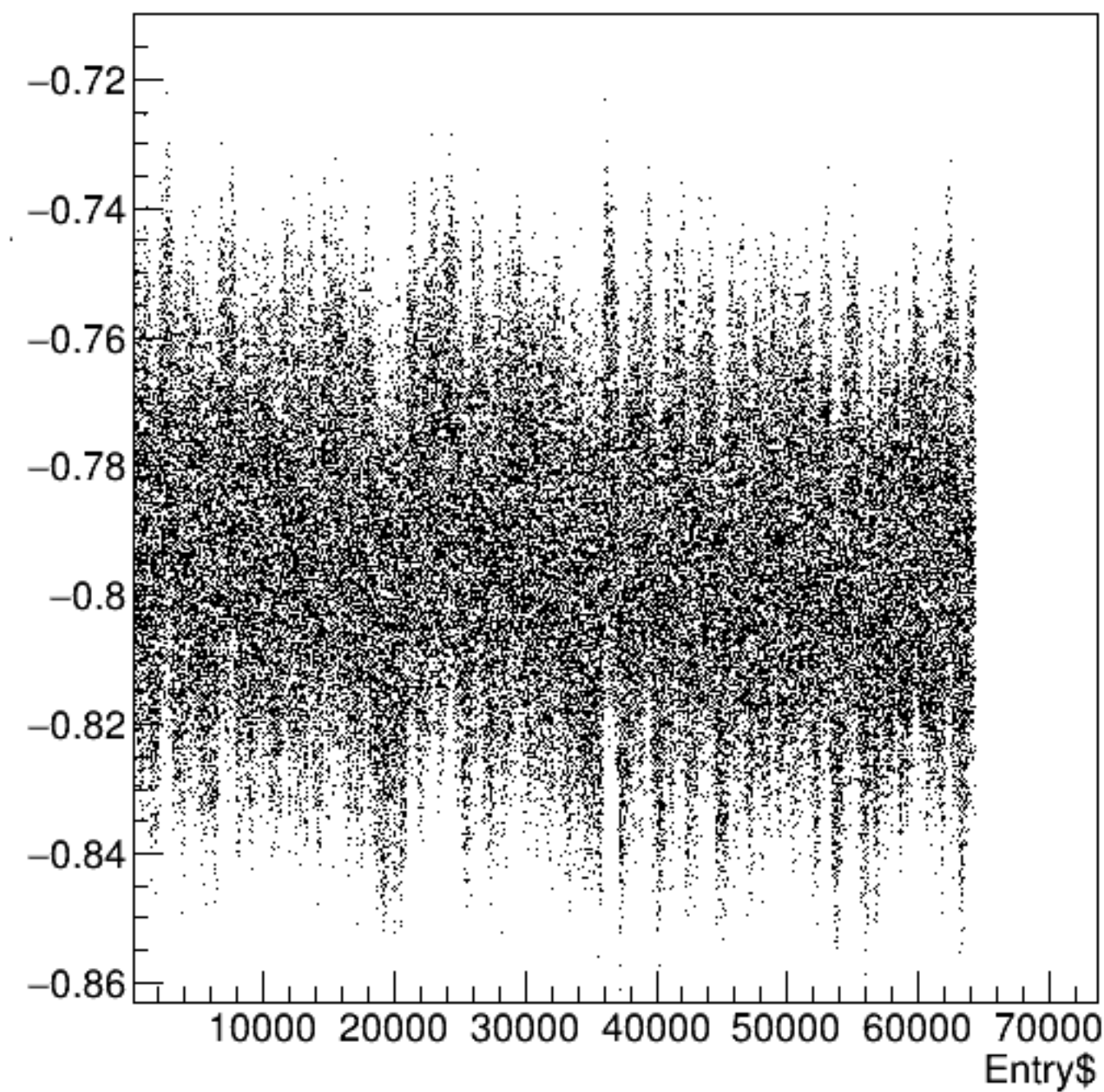
bpm0i02X/mm:Entry$ {ErrorFlag==0}
