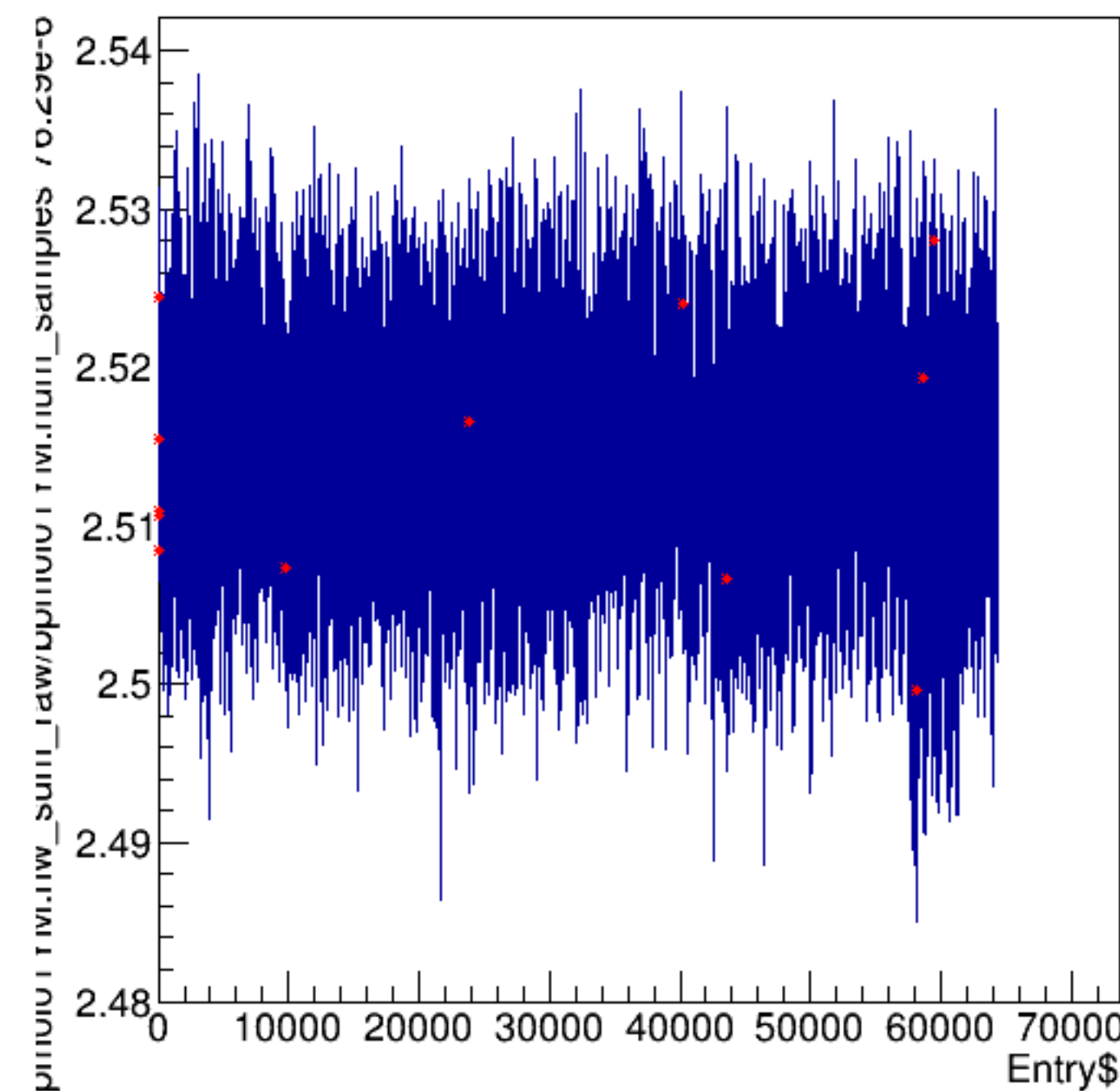
bpm0l01YM.hw_sum_raw/bpm0l01YM.num_samples*76.29e-6:Entry$
