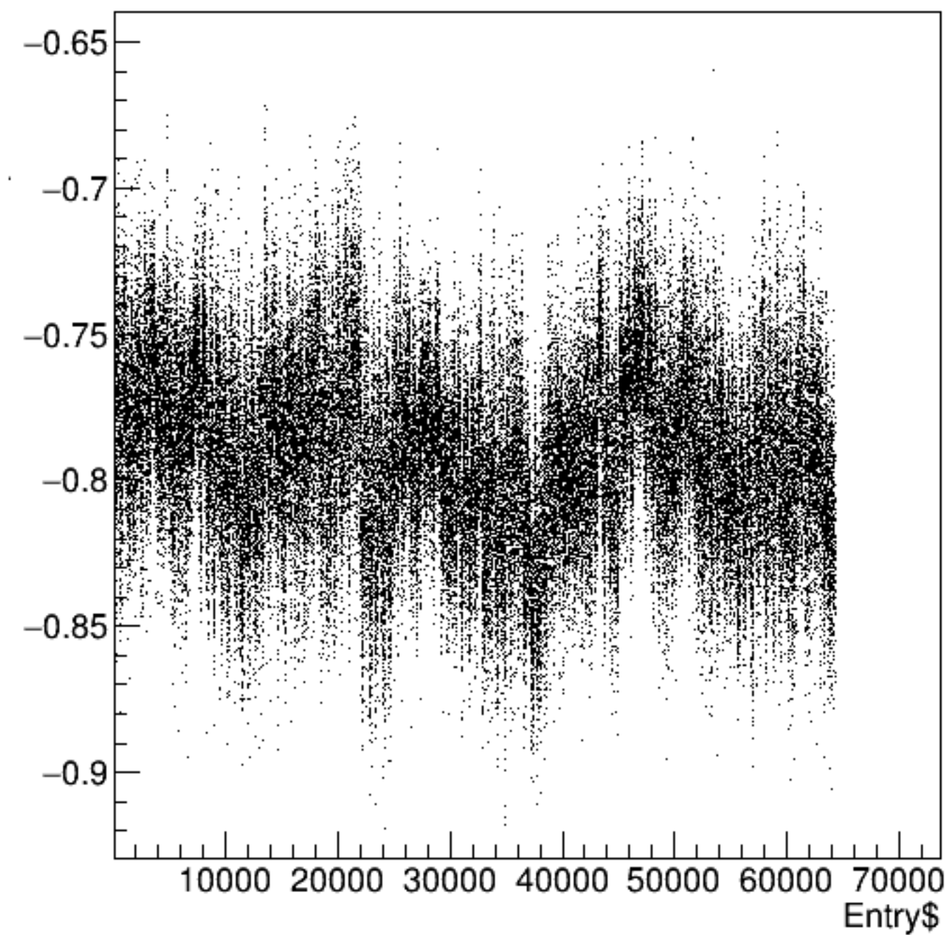
bpm12X/mm:Entry$ {ErrorFlag==0}
