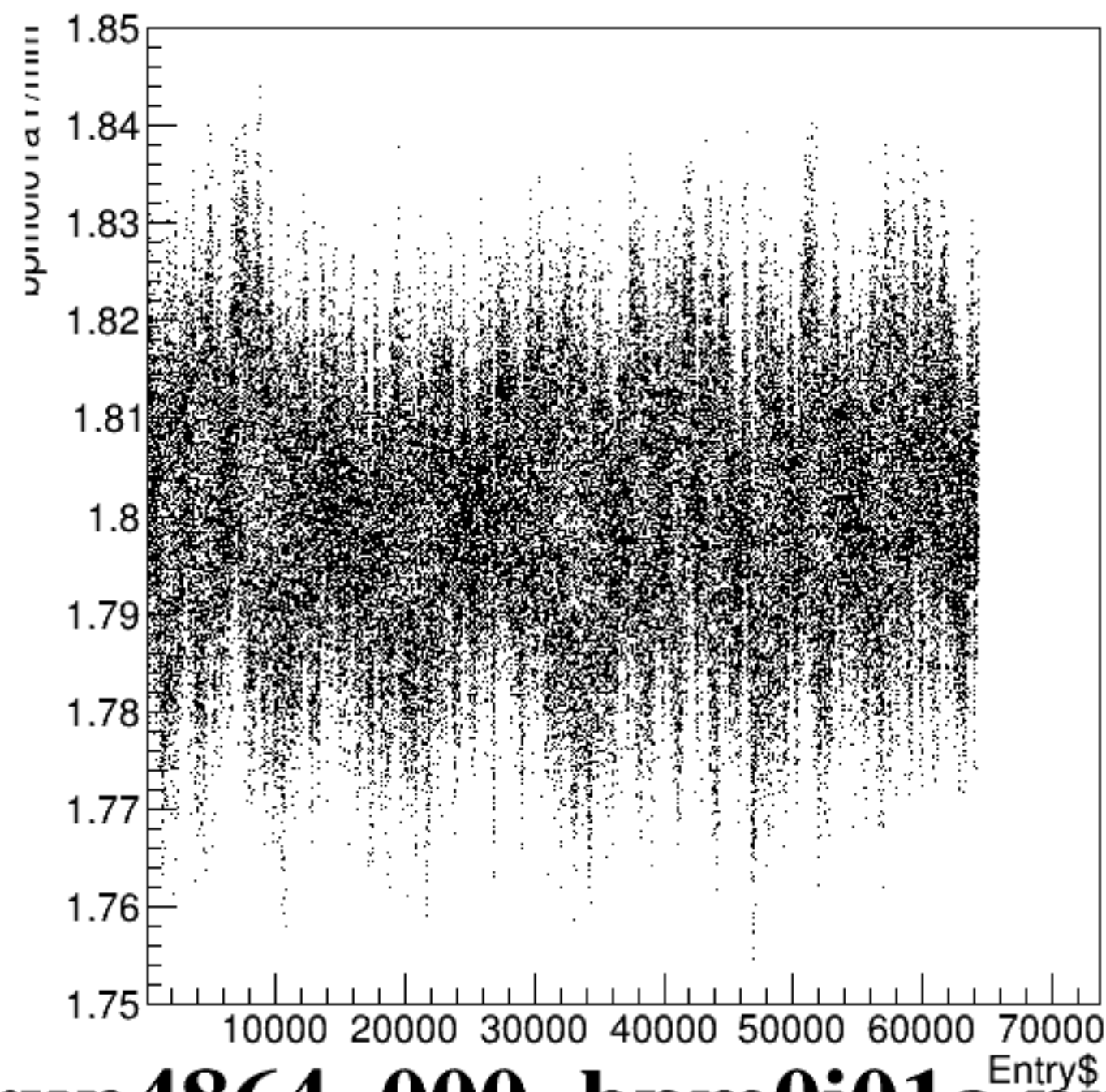
bpm0i01aY/mm:Entry$ {ErrorFlag==0}
