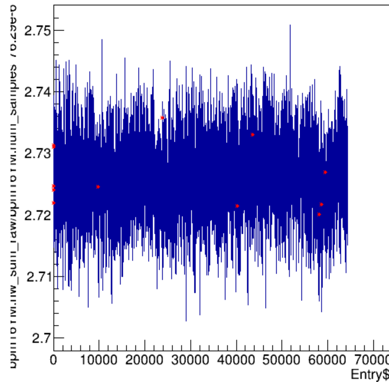
bpm16YM.hw_sum_raw/bpm16YM.num_samples*76.29e-6:Entry$
