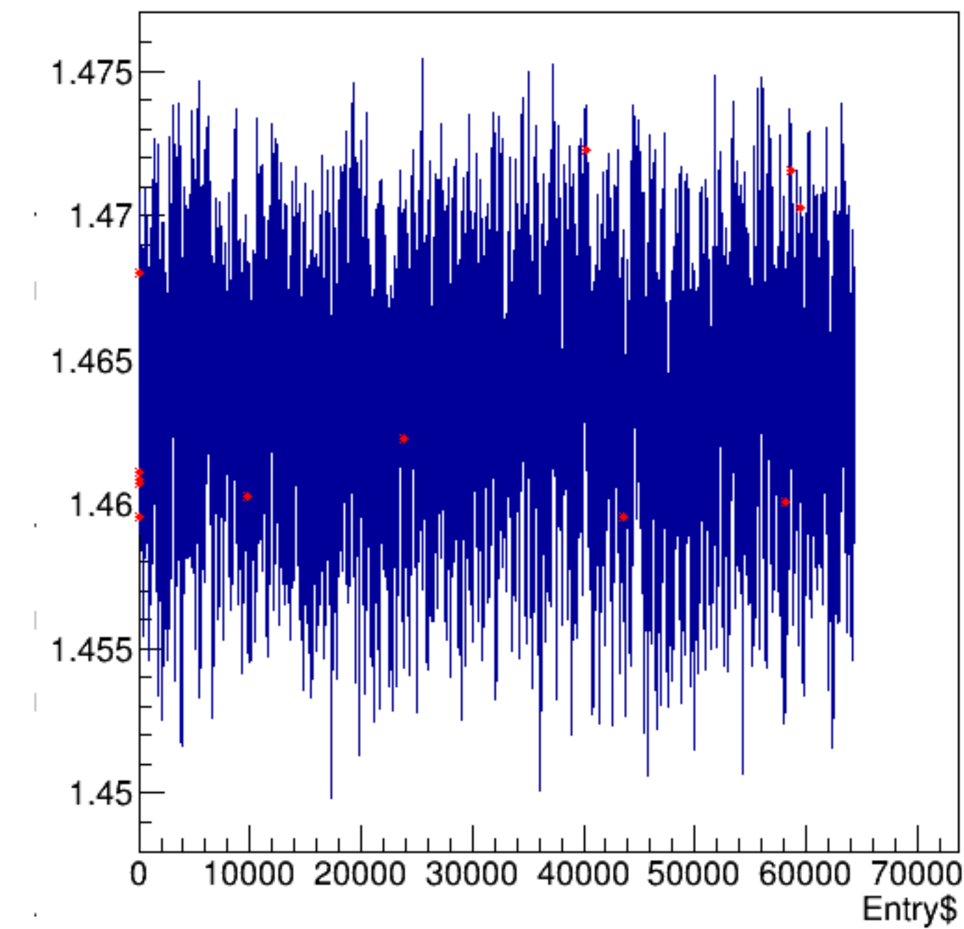
bpm2i01YP.hw_sum_raw/bpm2i01YP.num_samples*76.29e-6:Entry$
