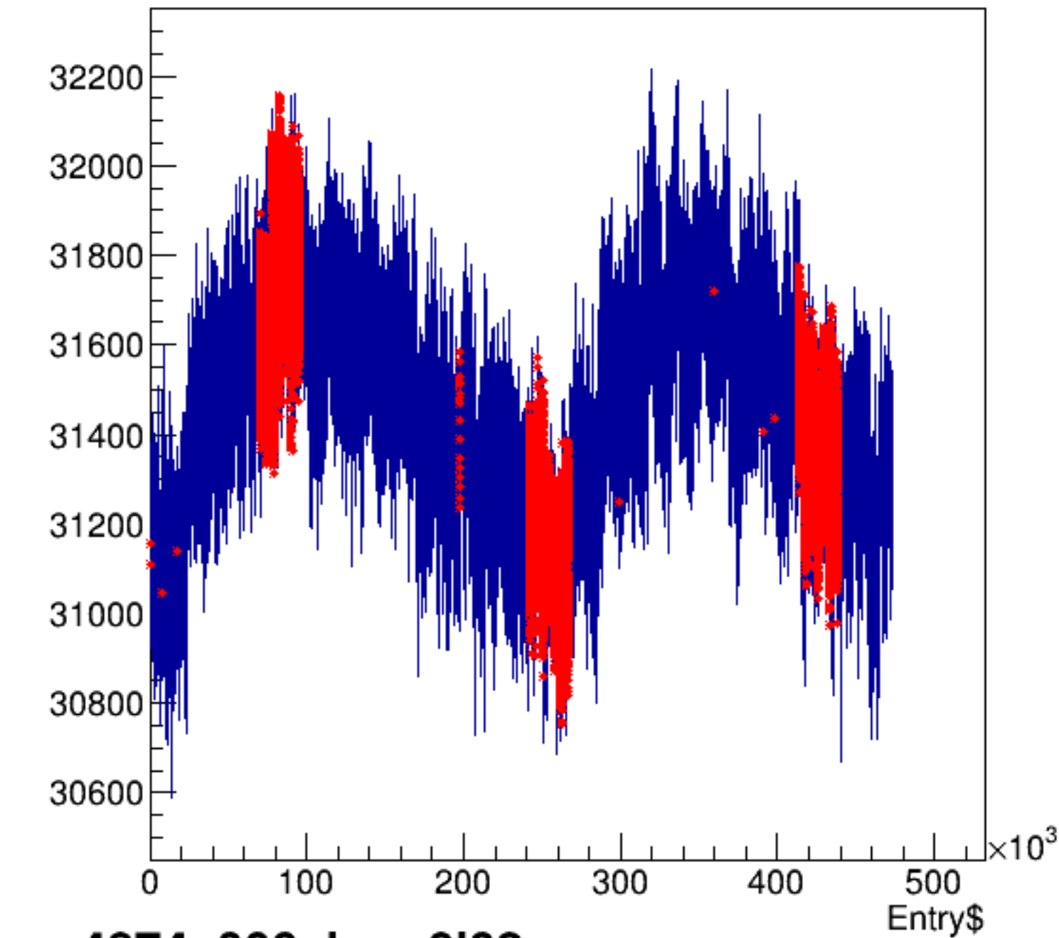
bcm0l02:Entry$
