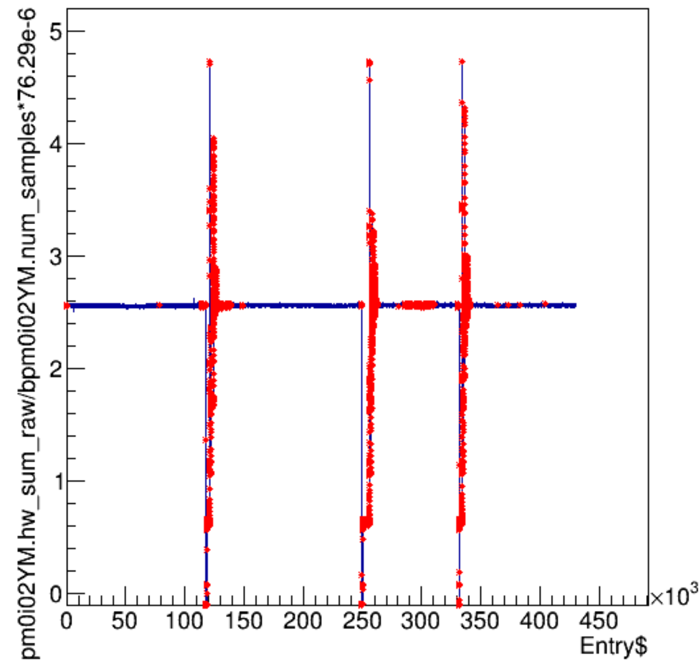
bpm0i02YM.hw_sum_raw/bpm0i02YM.num_samples*76.29e-6:Entry$
