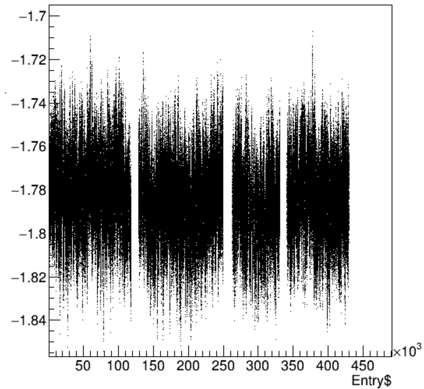
bpm0i01aX/mm:Entry$ {ErrorFlag==0}
