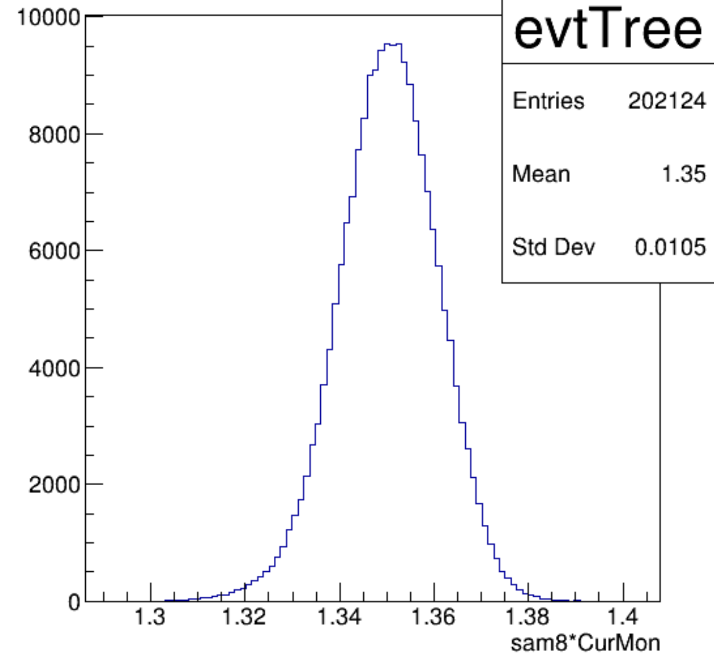
sam8*CurMon {ErrorFlag==0}
