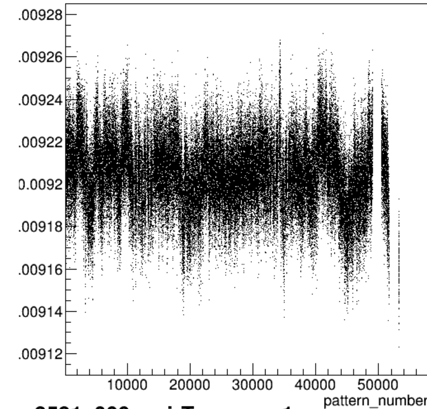
yield_sam1:pattern_number {ErrorFlag==0}
