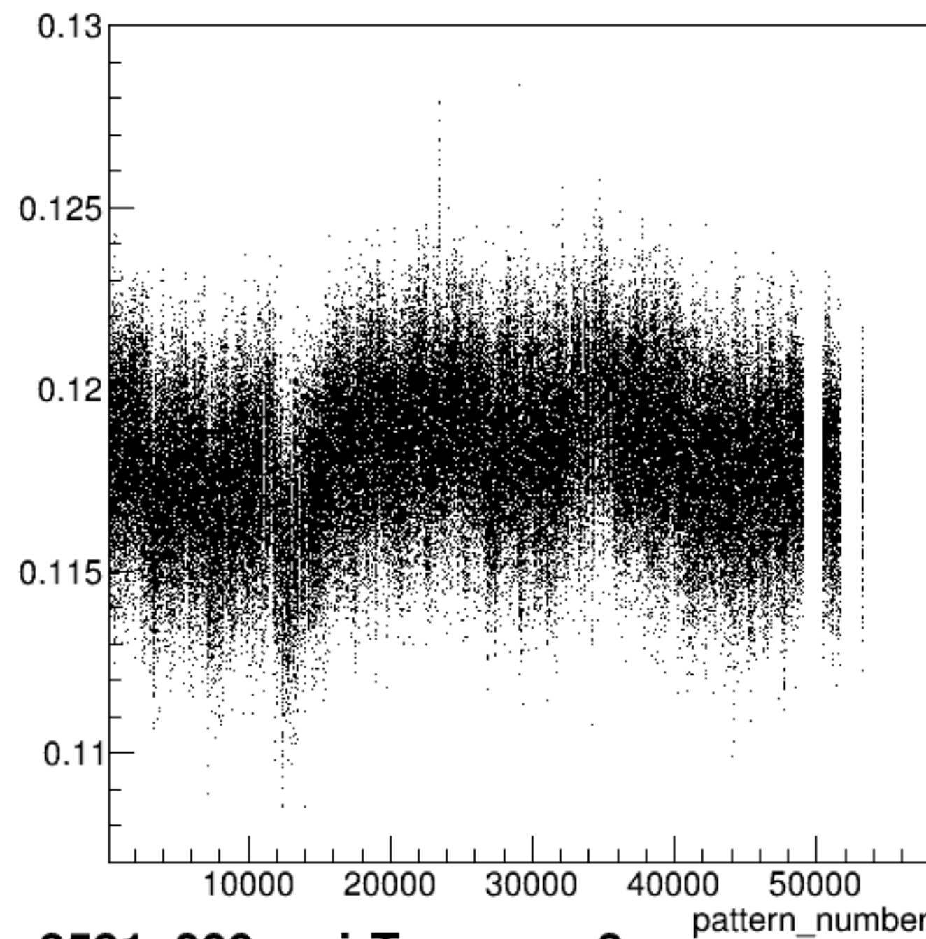
yield_sam3:pattern_number {ErrorFlag==0}
