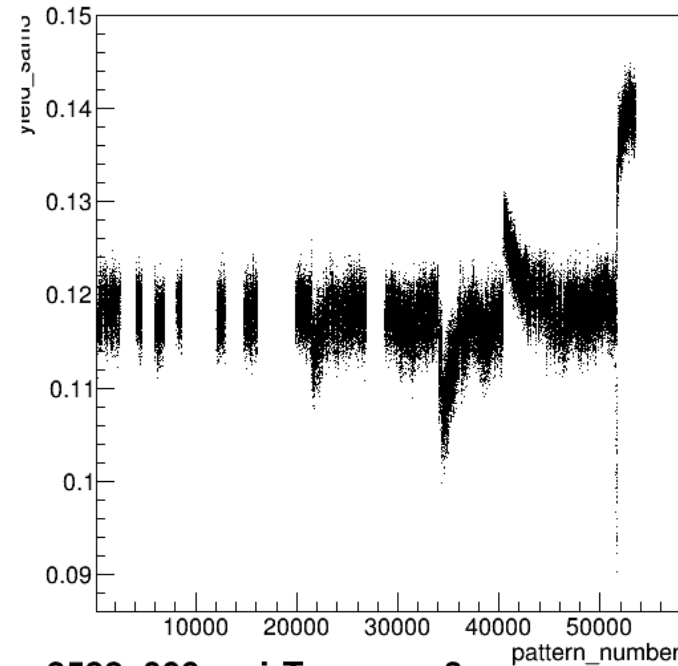
yield_sam3:pattern_number {ErrorFlag==0}
