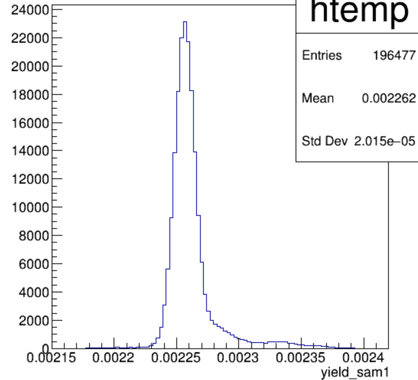
yield_sam1 {ErrorFlag==0}
