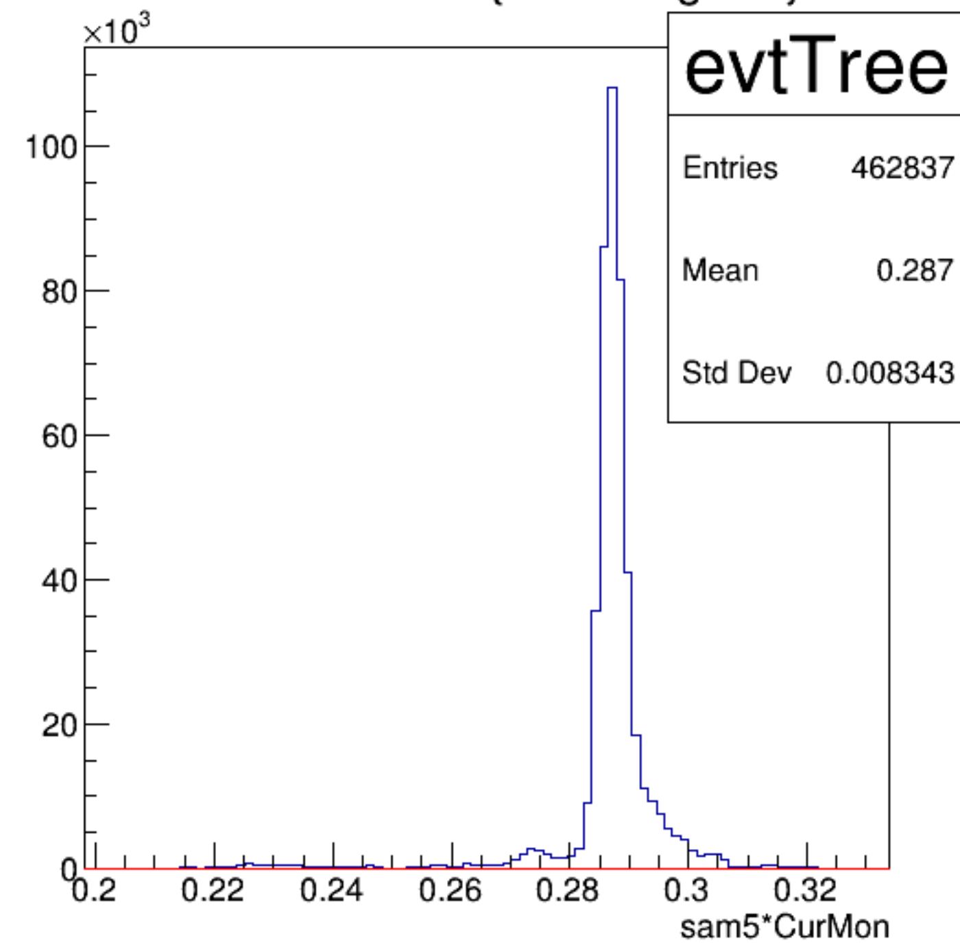
sam5*CurMon {ErrorFlag==0}
