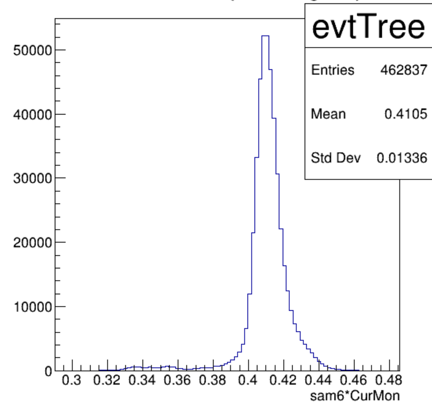
sam6*CurMon {ErrorFlag==0}
