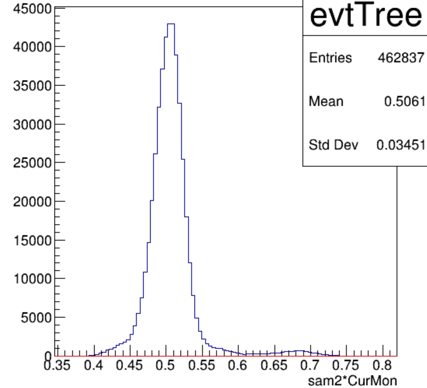
sam2*CurMon {ErrorFlag==0}
