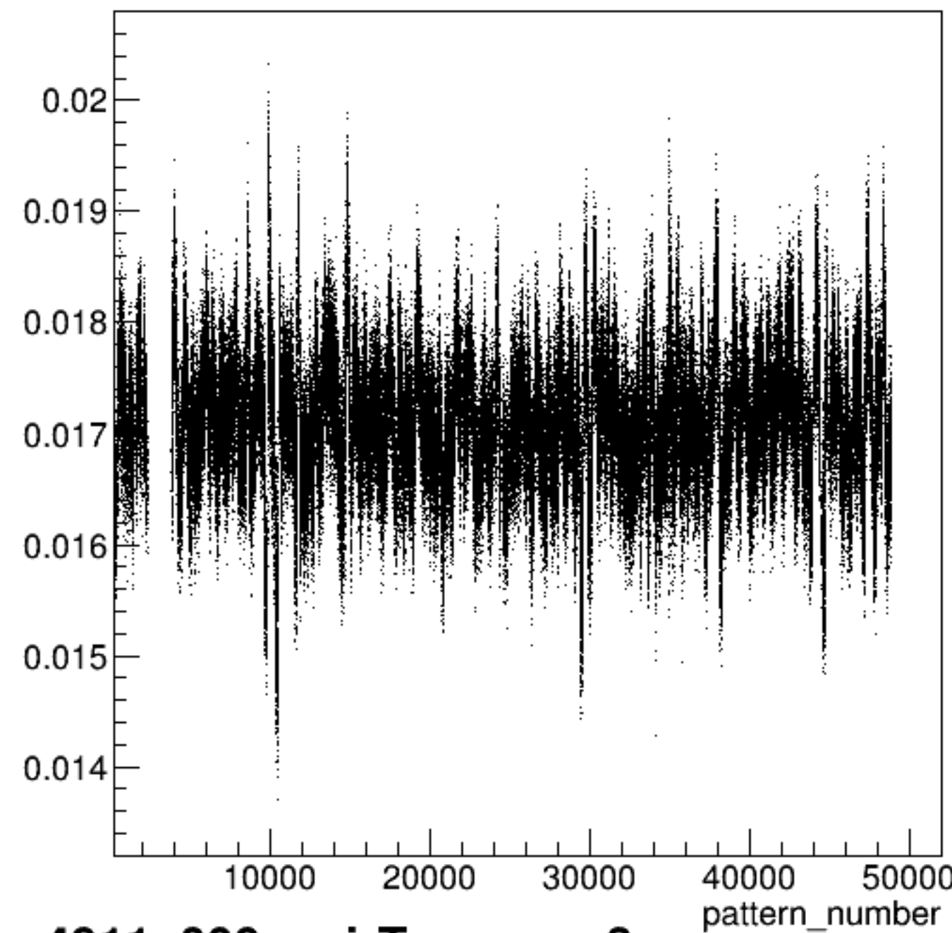
yield_sam3:pattern_number {ErrorFlag==0}
