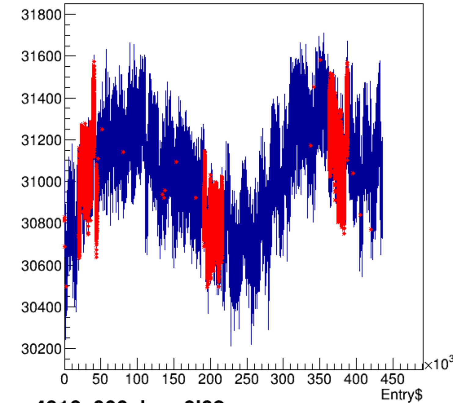
bcm0l02:Entry$
