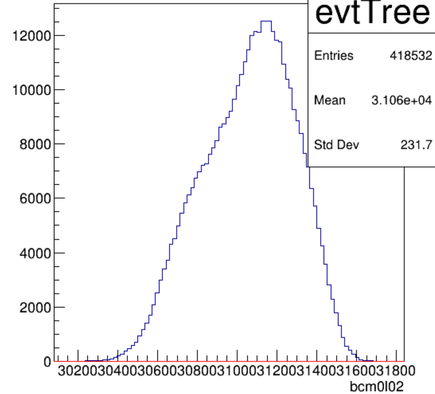
bcm0l02 {ErrorFlag==0}
