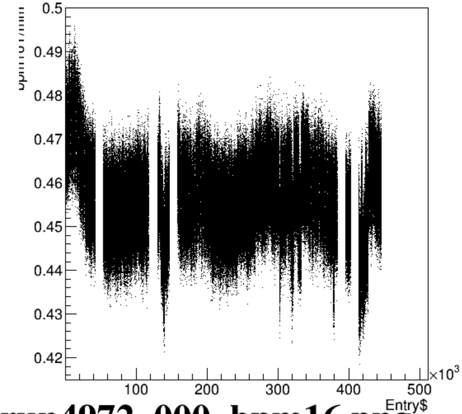
bpm16Y/mm:Entry$ {ErrorFlag==0}
