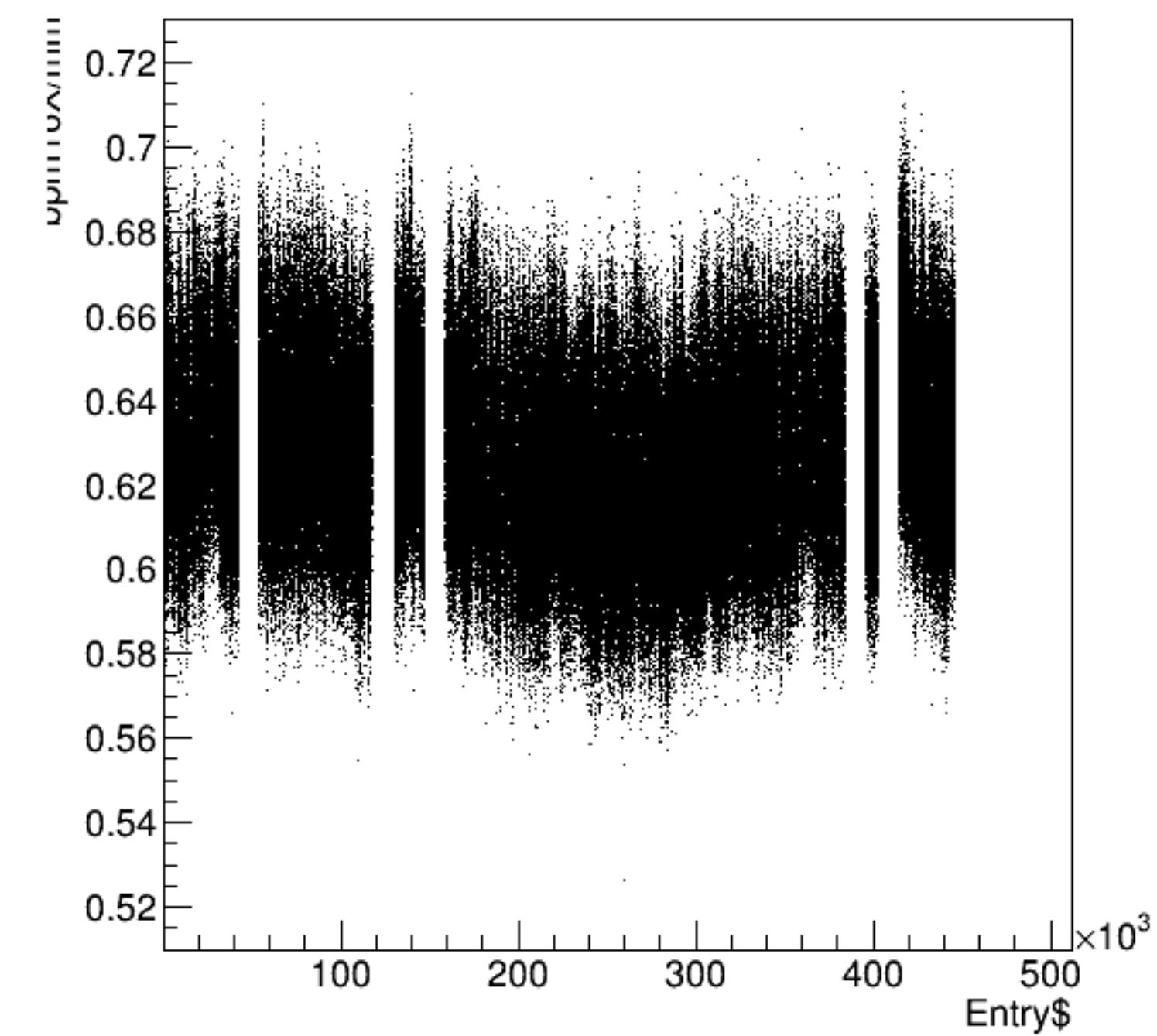
bpm16X/mm:Entry$ {ErrorFlag==0}
