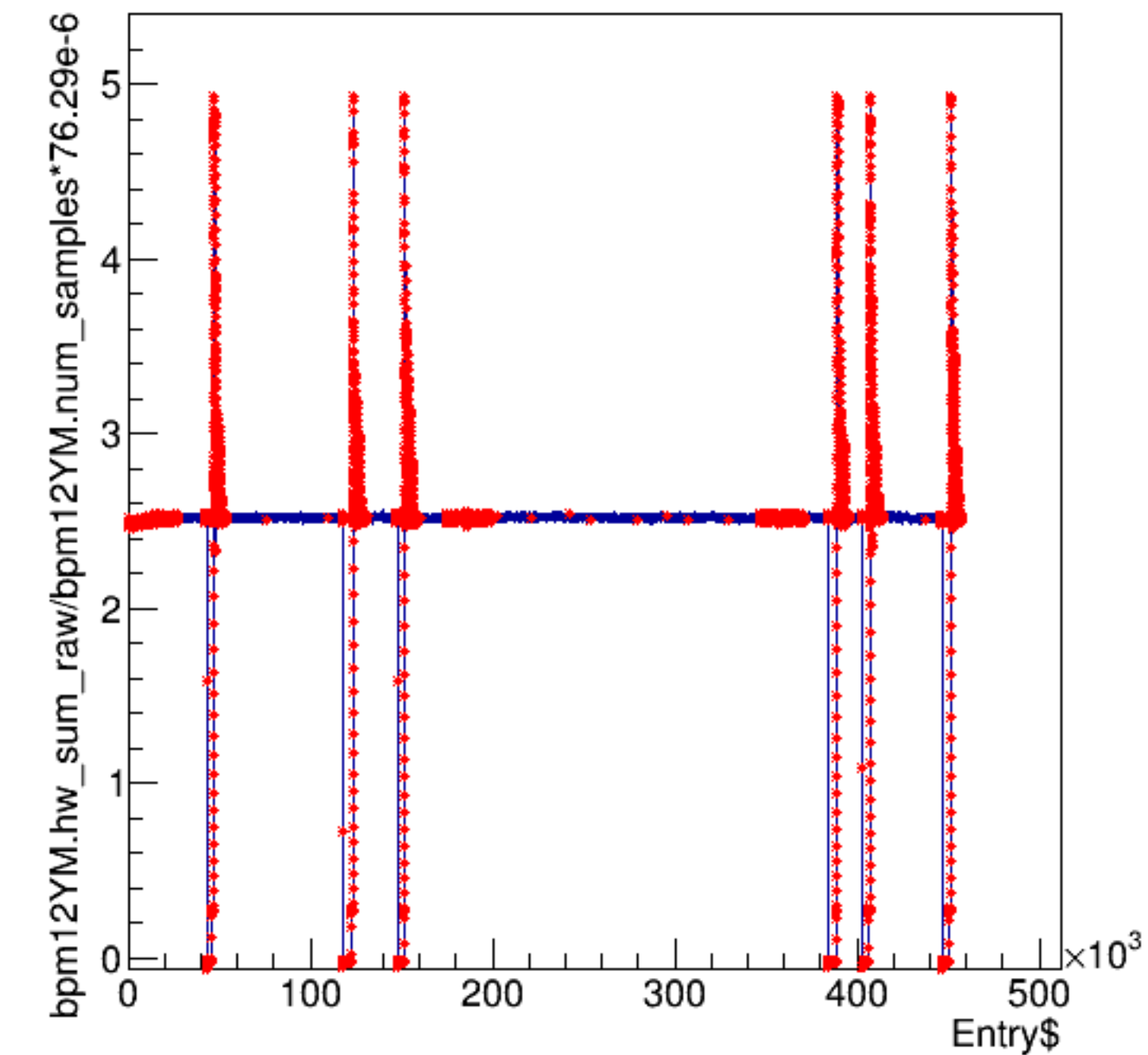
bpm12YM.hw_sum_raw/bpm12YM.num_samples*76.29e-6:Entry$
