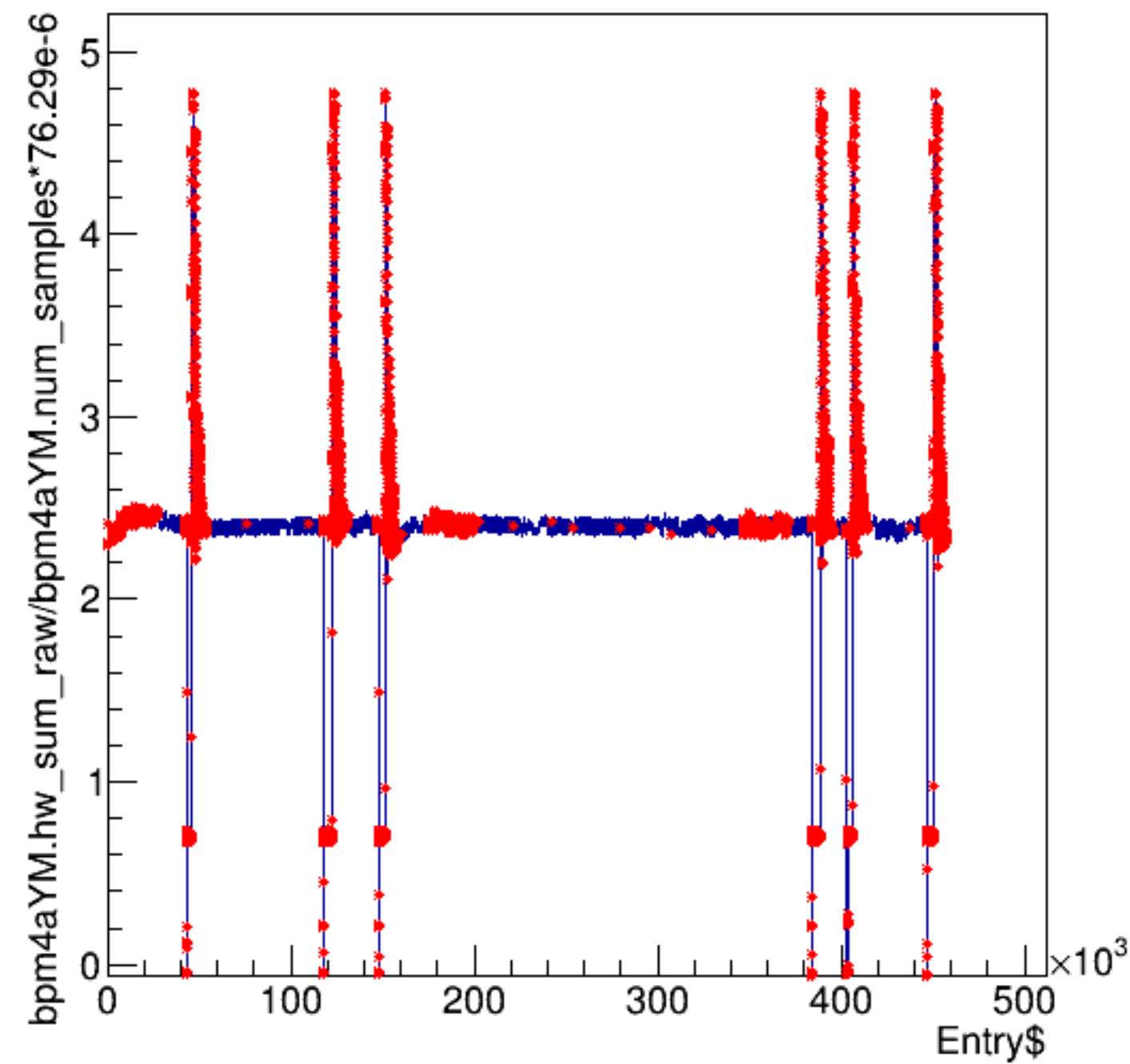
bpm4aYM.hw_sum_raw/bpm4aYM.num_samples*76.29e-6:Entry$
