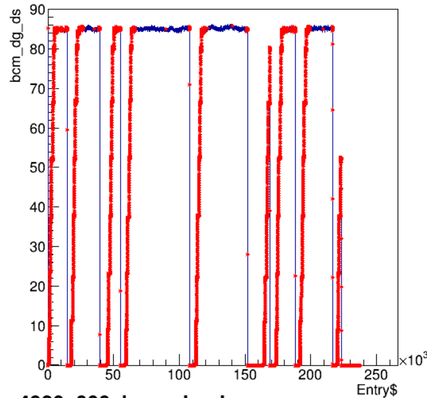
bcm_dg_ds:Entry$
