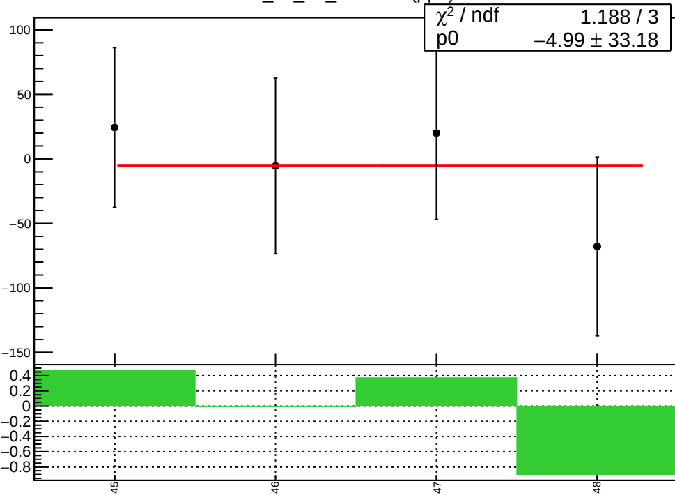
corr_us_dd_evMon1 (ppb)
