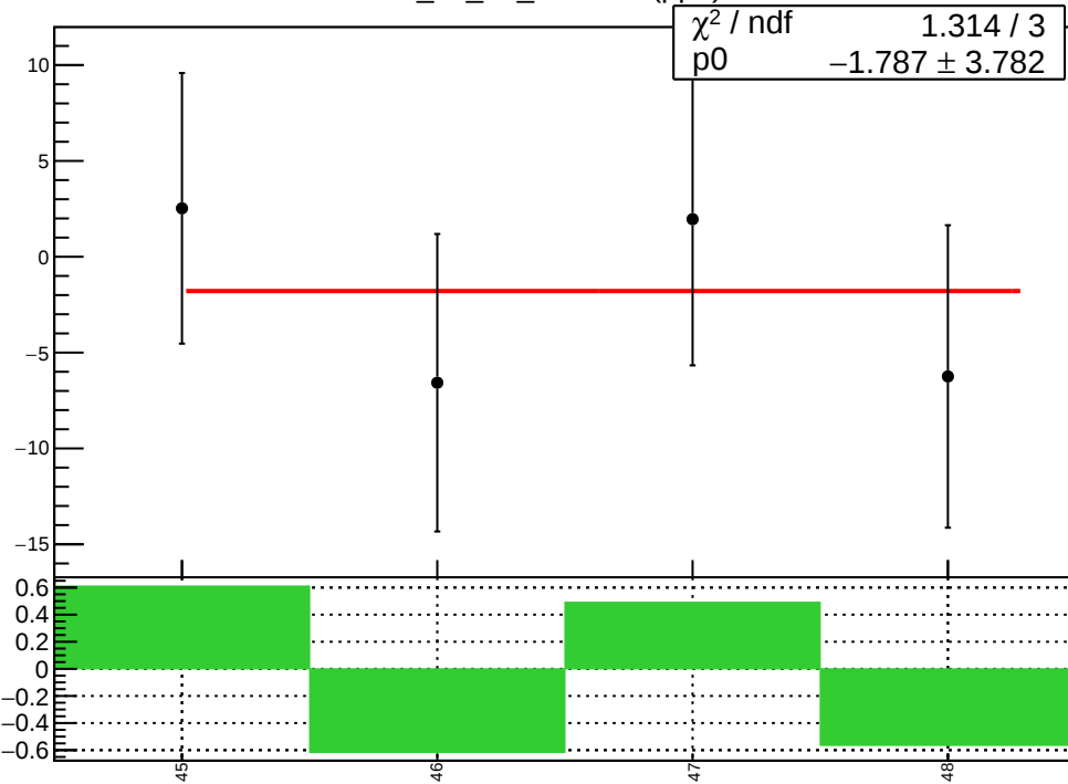
corr_us_dd_evMon8 (ppb)
