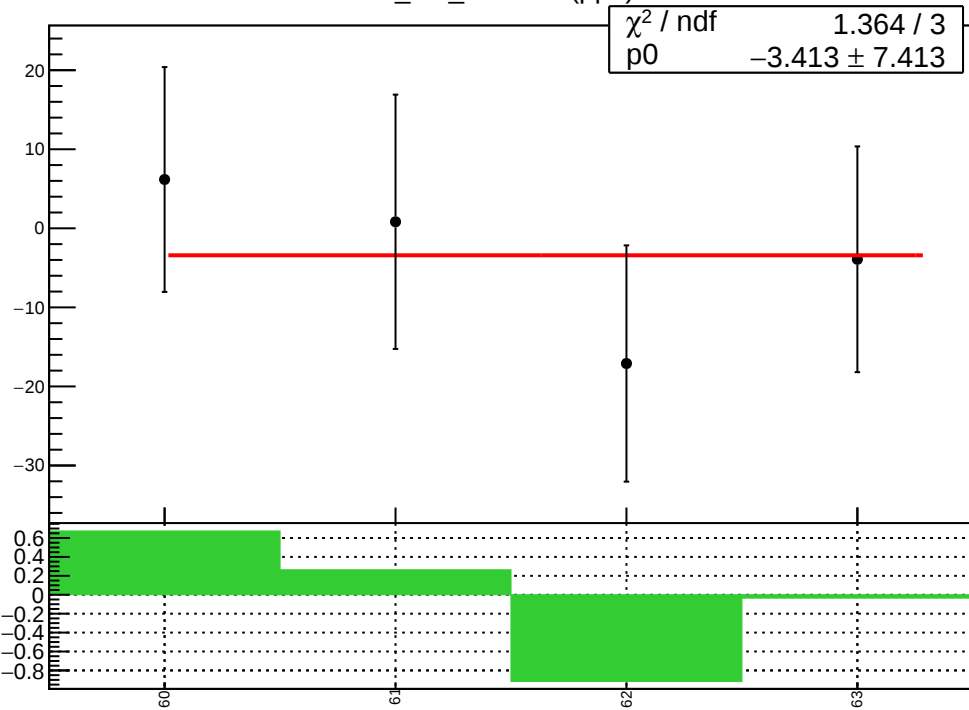
corr_usr_evMon7 (ppb)
