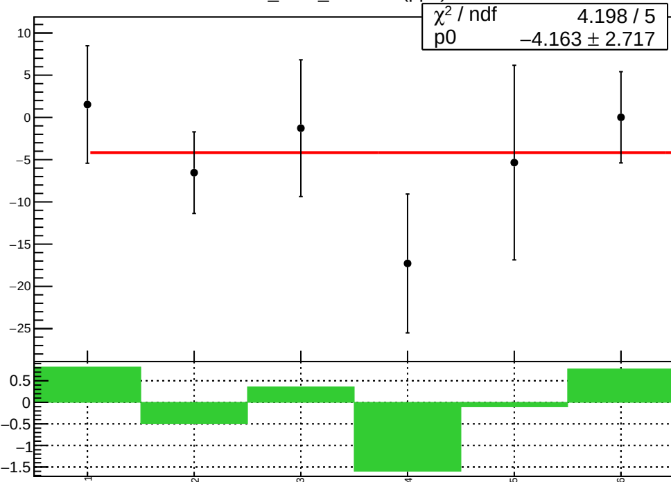
corr_Adet_evMon9 (ppb)
