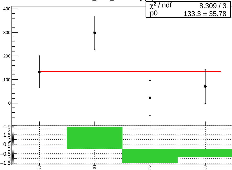
corr_Adet_evMon4 (ppb)
