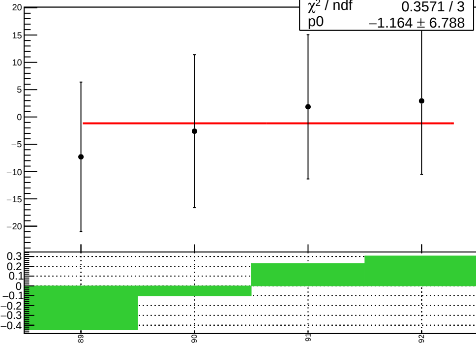
corr_Adet_evMon7 (ppb)
