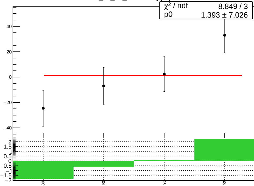
corr_us_dd_evMon6 (ppb)
