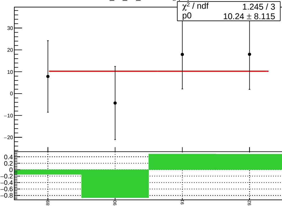
corr_us_dd_evMon3 (ppb)
