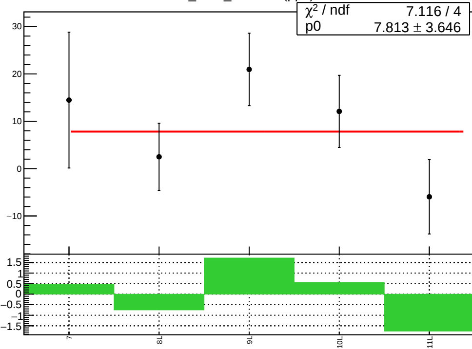
corr_Adet_evMon8 (ppb)
