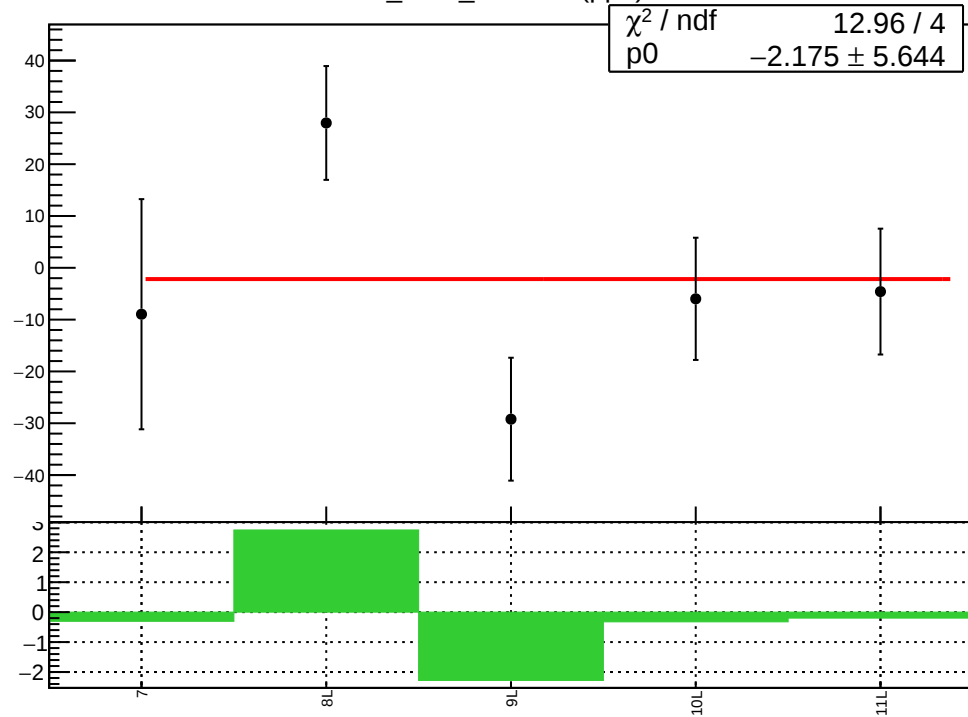
corr_Adet_evMon5 (ppb)
