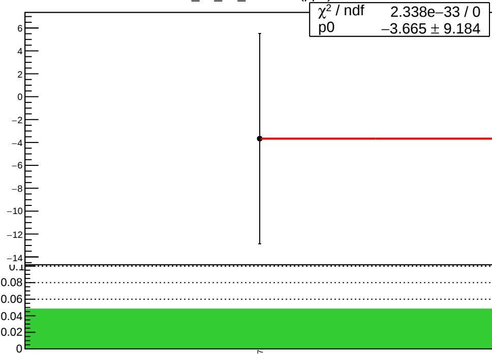
corr_us_dd_evMon9 (ppb)
