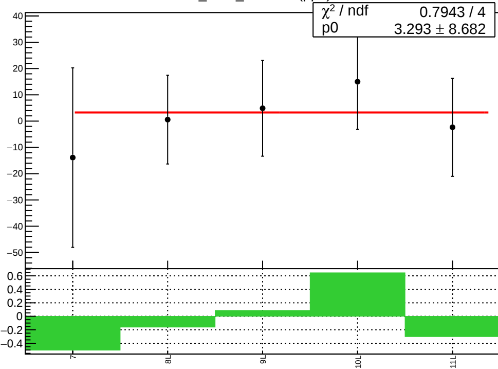
corr_Adet_evMon7 (ppb)
