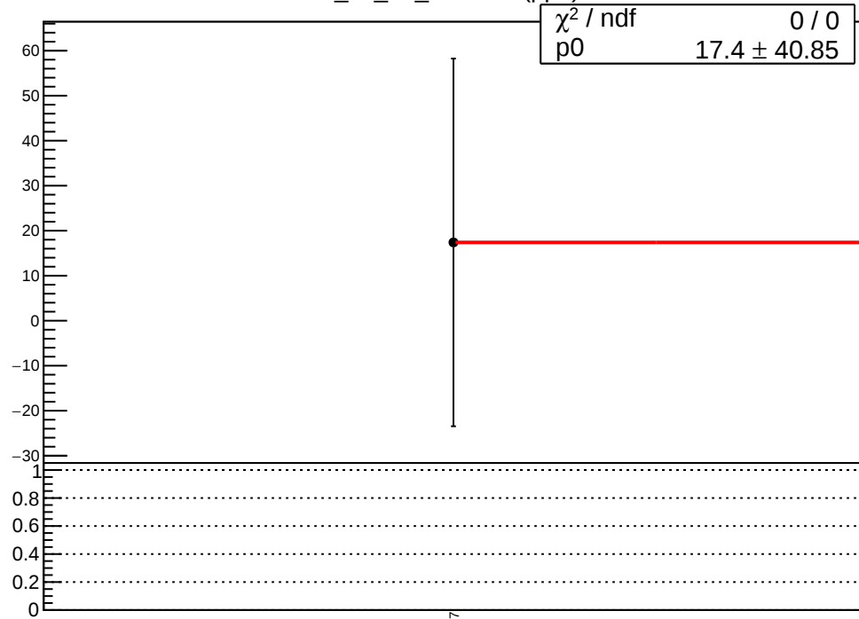
corr_us_dd_evMon3 (ppb)
