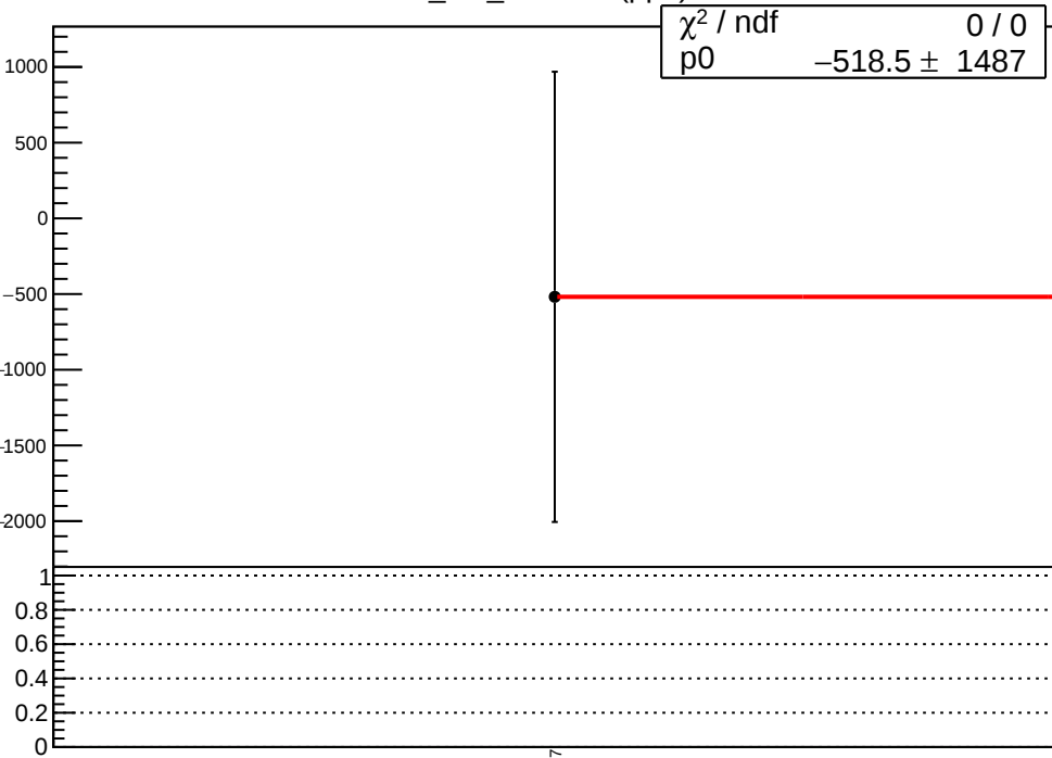
corr_usr_evMon0 (ppb)
