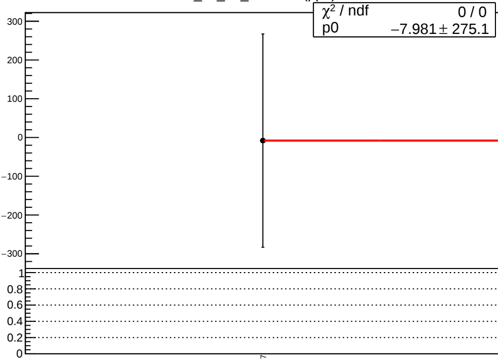
corr_us_dd_evMon1 (ppb)
