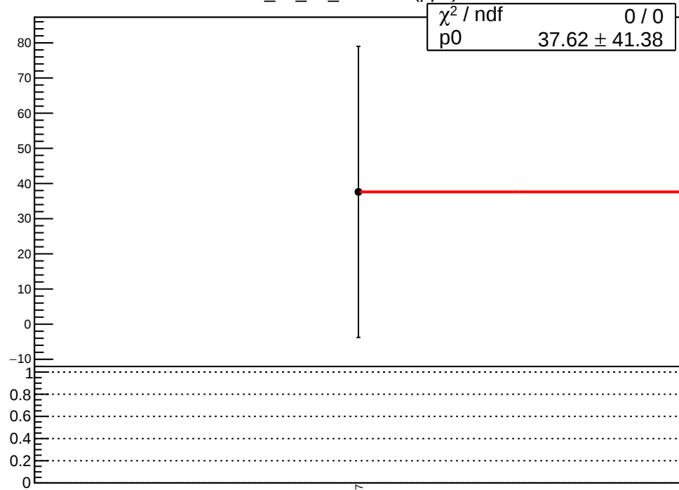
corr_us_dd_evMon4 (ppb)
