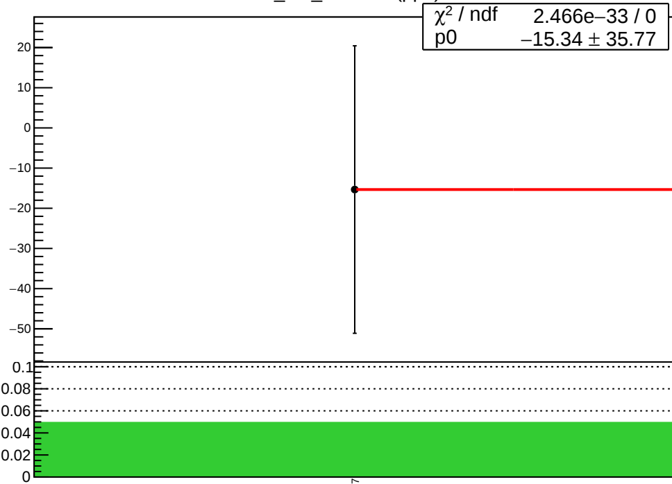
corr_usr_evMon7 (ppb)
