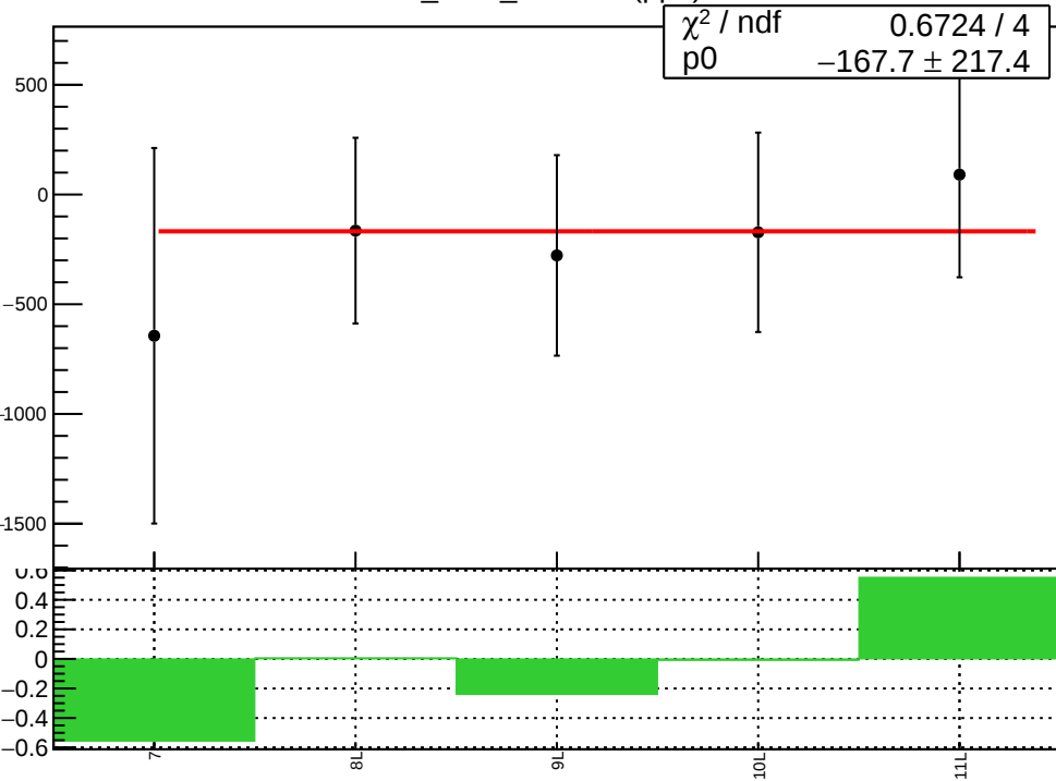
corr_Adet_evMon2 (ppb)
