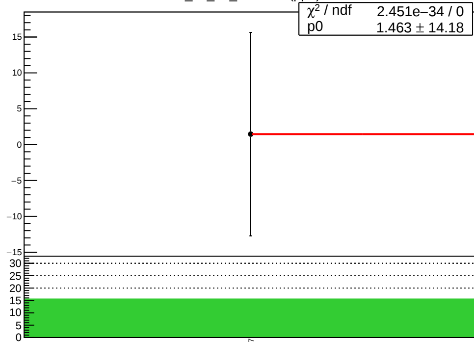
corr_us_dd_evMon7 (ppb)
