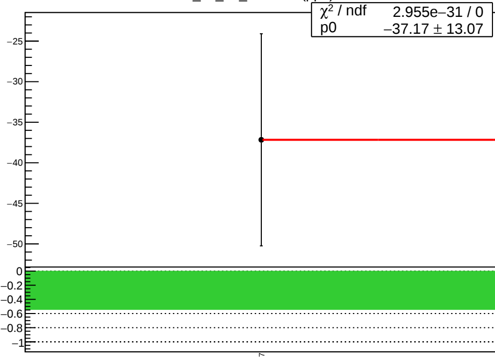
corr_us_dd_evMon5 (ppb)
