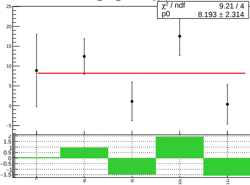
corr_Adet_evMon11 (ppb)
