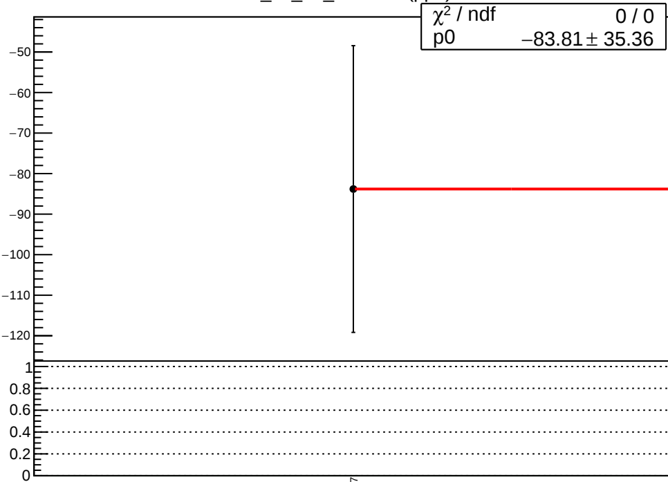
corr_us_dd_evMon6 (ppb)
