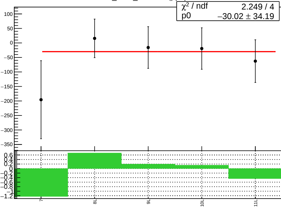
corr_Adet_evMon4 (ppb)
