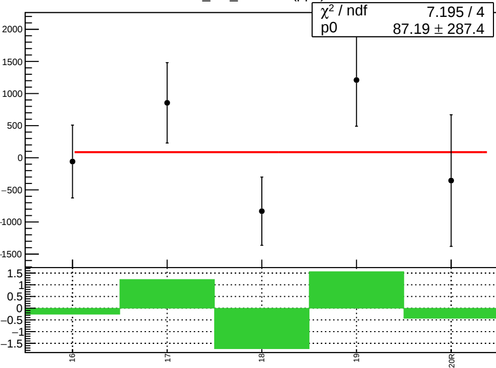
corr_usr_evMon0 (ppb)
