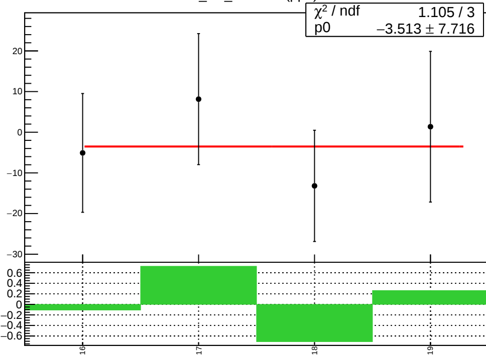
corr_usl_evMon7 (ppb)
