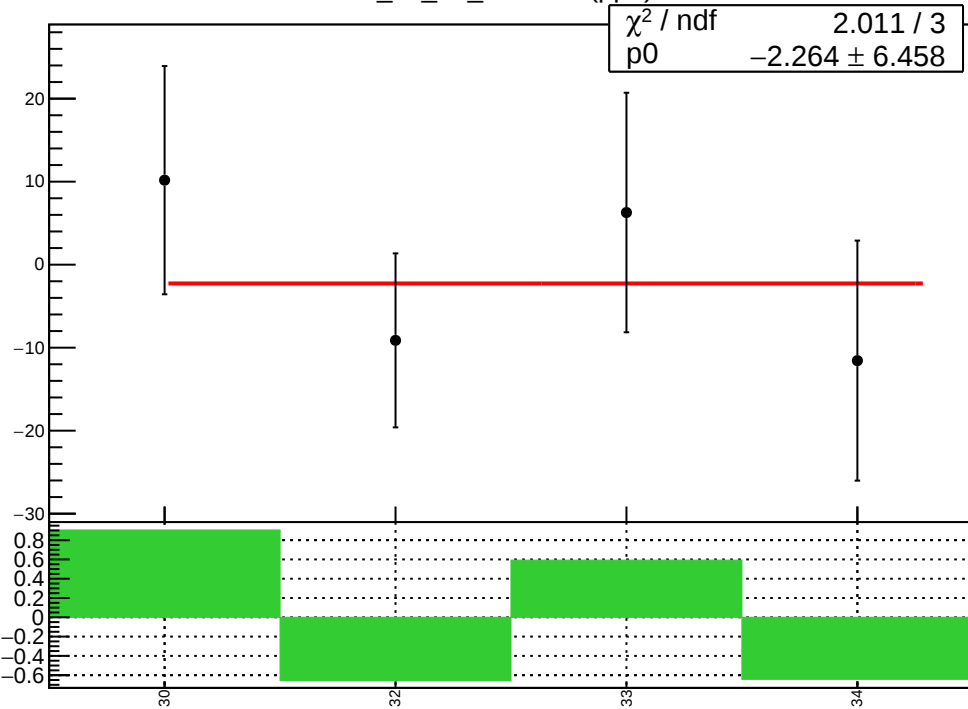
corr_us_dd_evMon6 (ppb)
