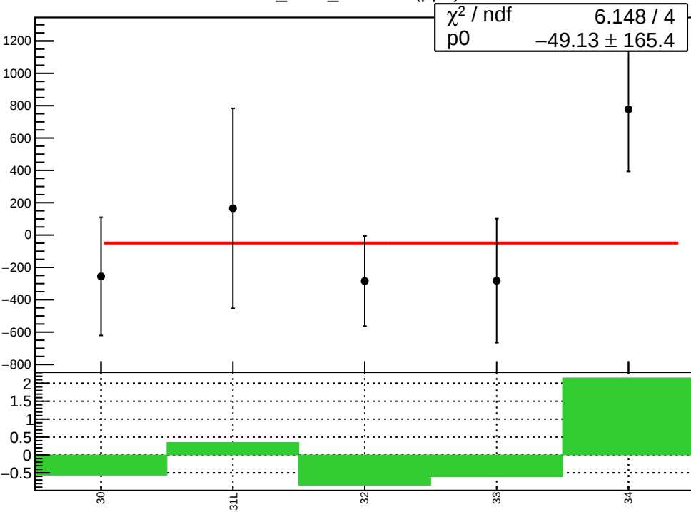
corr_Adet_evMon2 (ppb)
