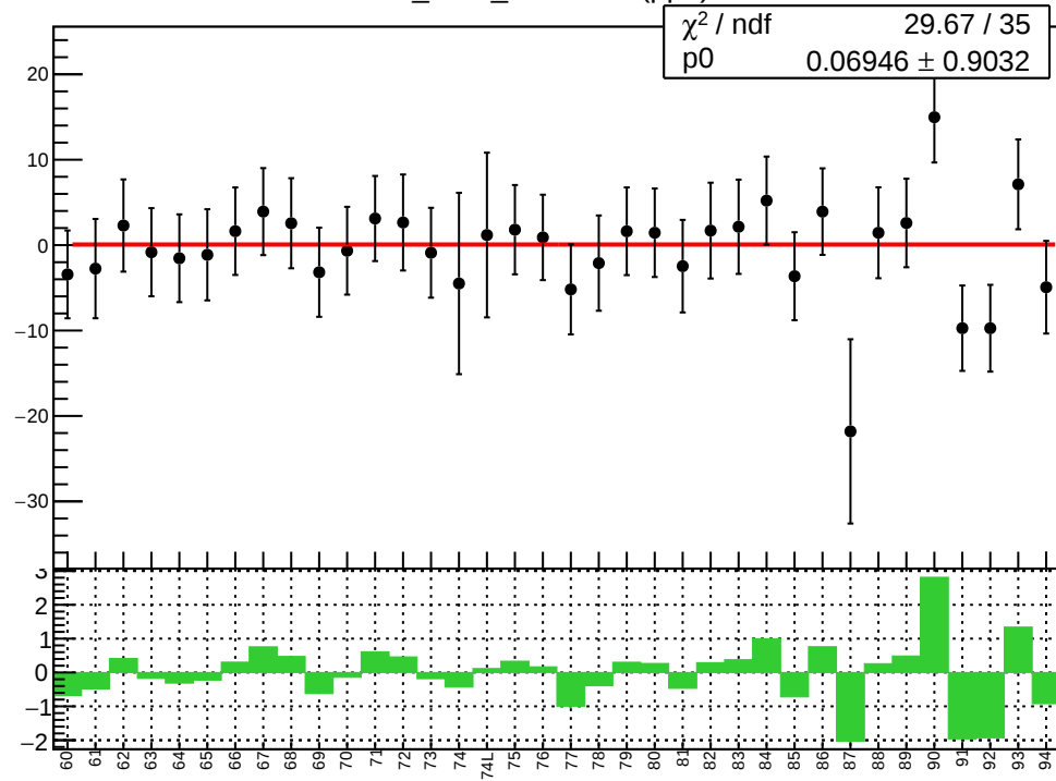
corr_Adet_evMon10 (ppb)
