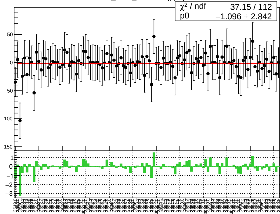
corr_Adet_evMon9 (ppb)
