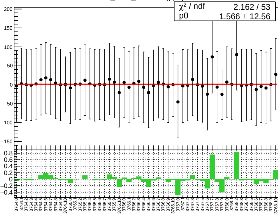
corr_Adet_evMon6 (ppb)
