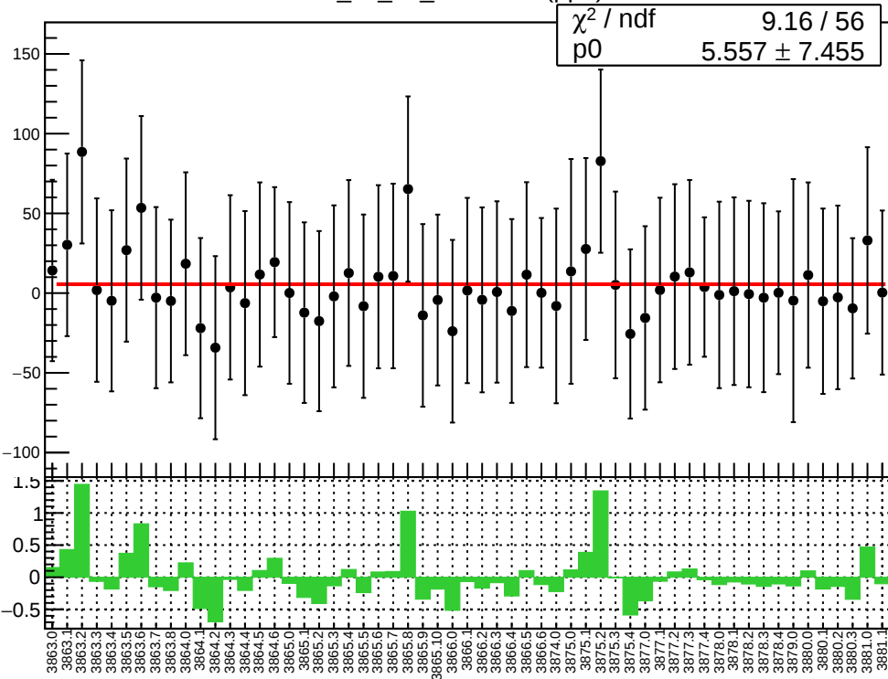
corr_us_dd_evMon10 (ppb)
