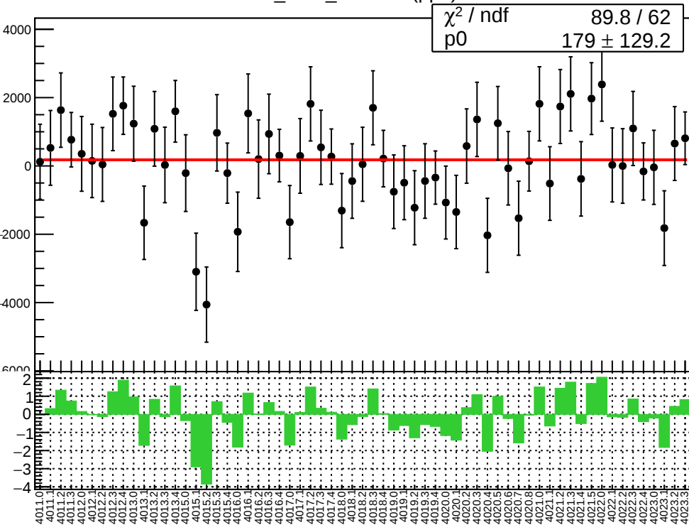
corr_Adet_evMon1 (ppb)
