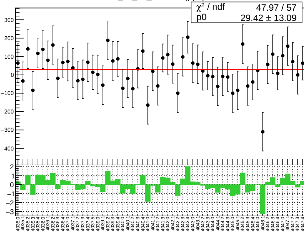
corr_us_dd_evMon6 (ppb)
