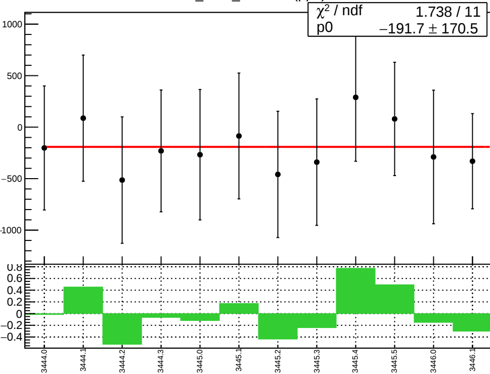
corr_Adet_evMon4 (ppb)
