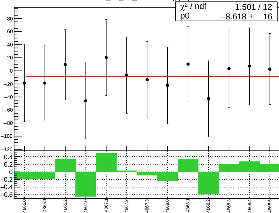
corr_us_dd_evMon10 (ppb)
