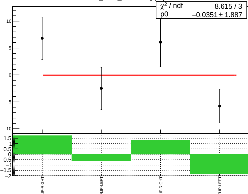
corr_Adet_evMon7 (ppb)
