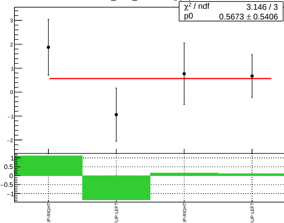
corr_Adet_evMon10 (ppb)
