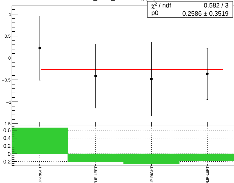
corr_Adet_evMon5 (ppb)
