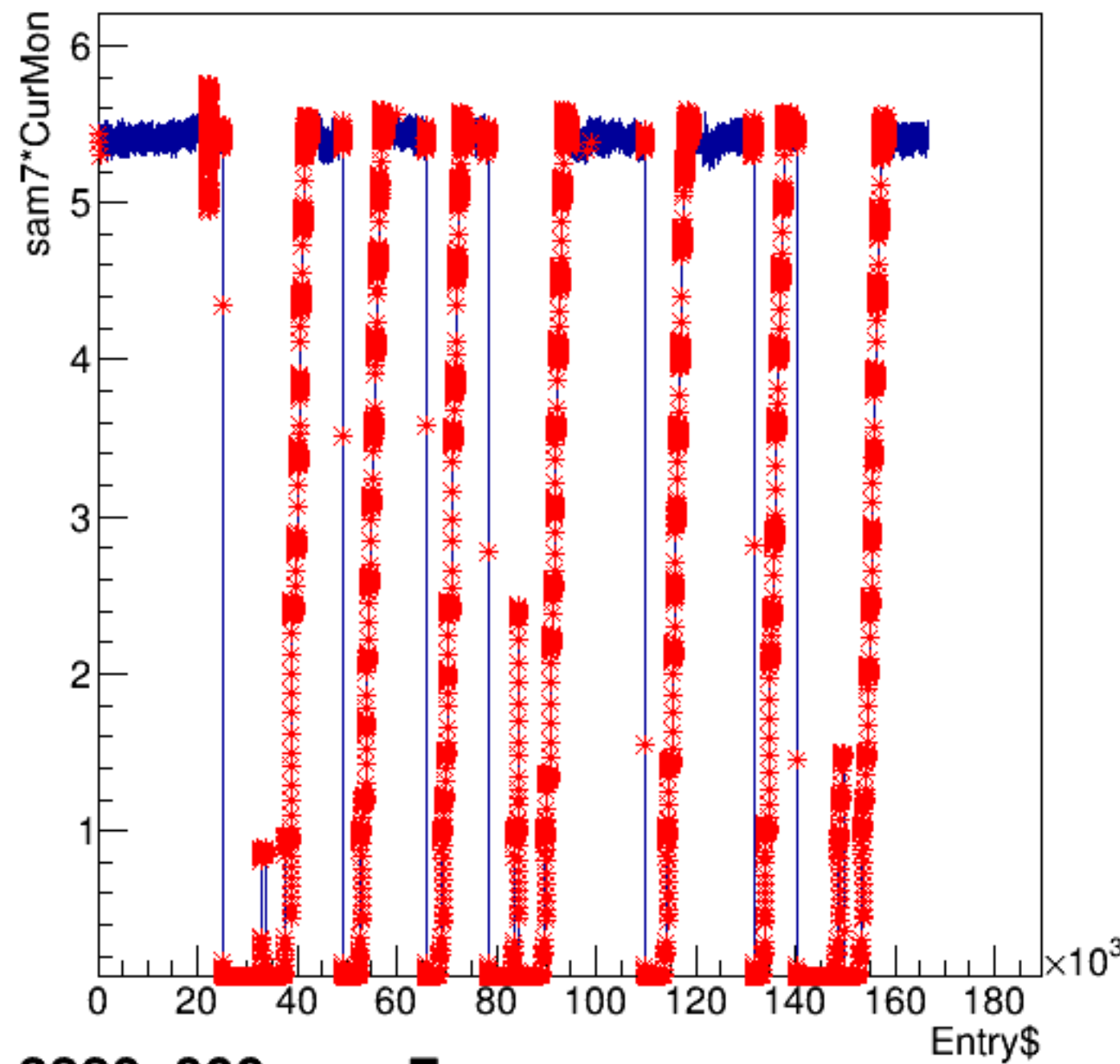
sam7*CurMon:Entry$
