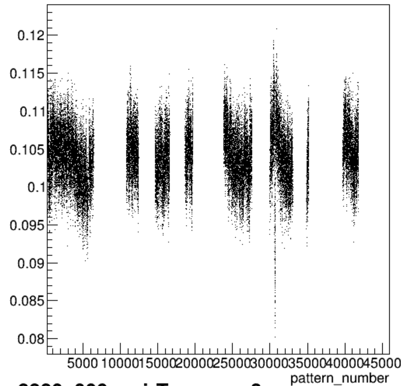
yield_sam3:pattern_number {ErrorFlag==0}
