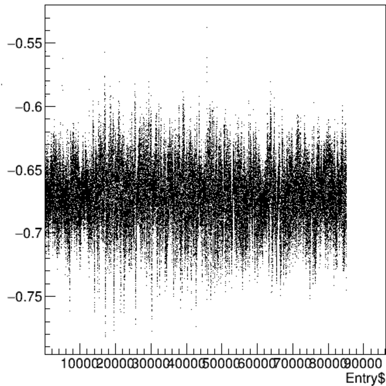
bpm0i02X/mm:Entry$ {ErrorFlag==0}
