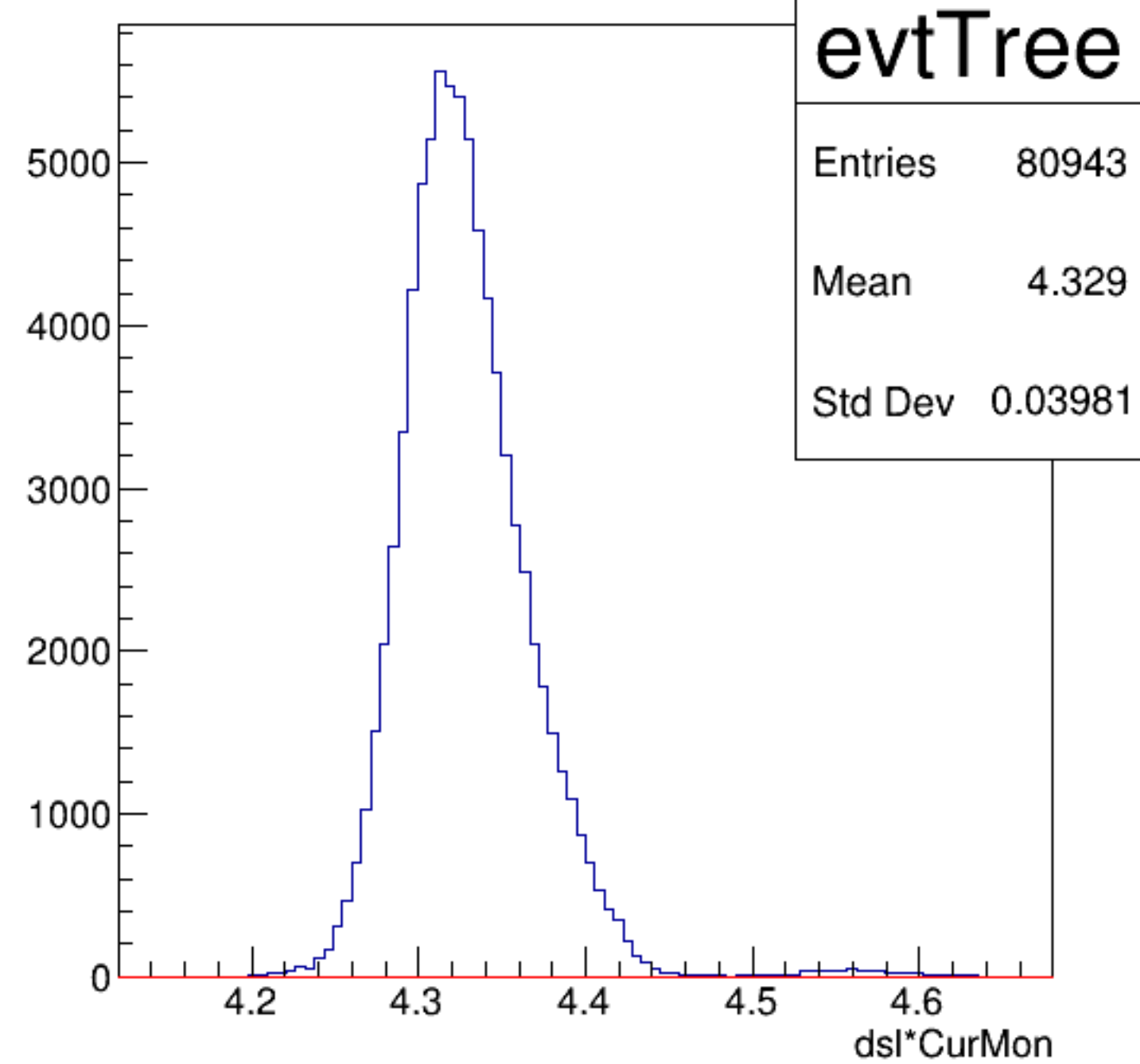
dsl*CurMon {ErrorFlag==0}
