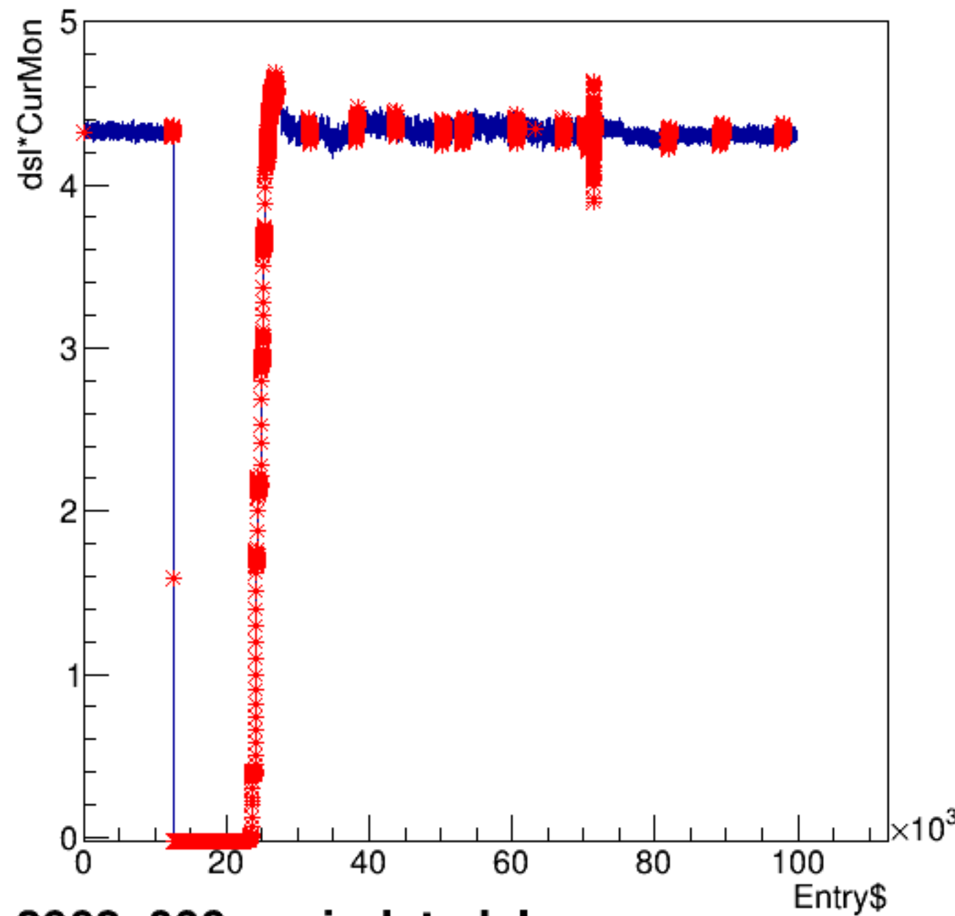
dsl*CurMon:Entry$
