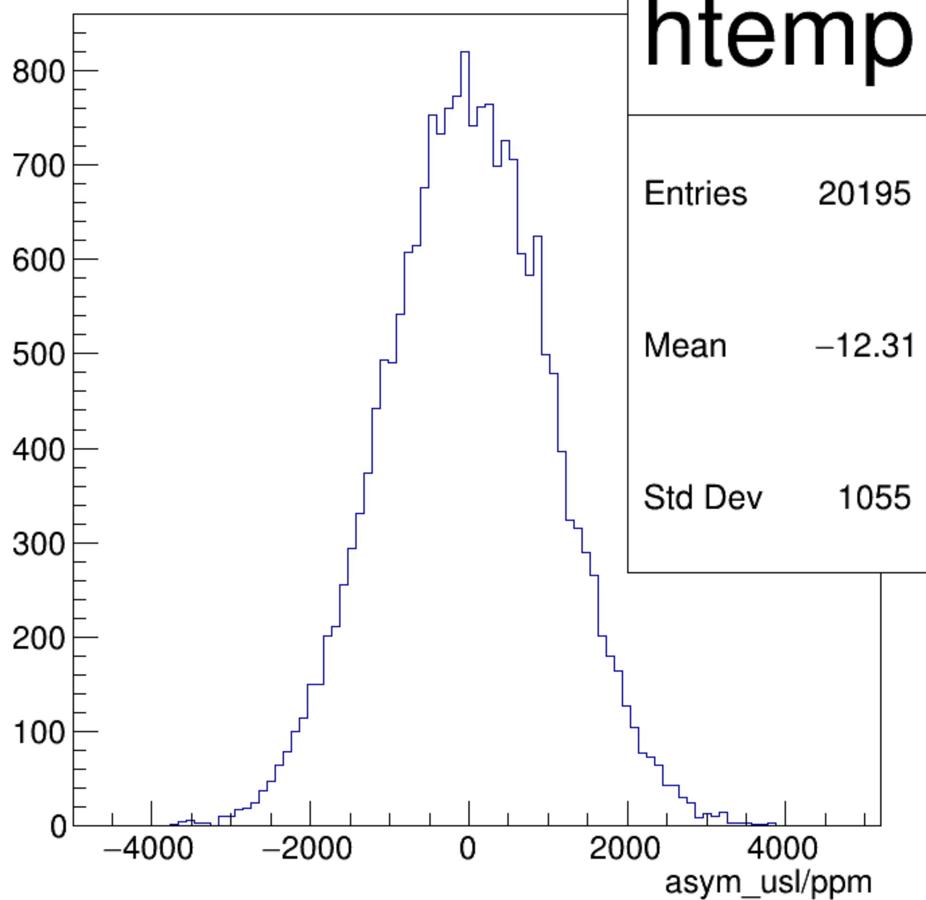
asym_usl/ppm {ErrorFlag==0}
