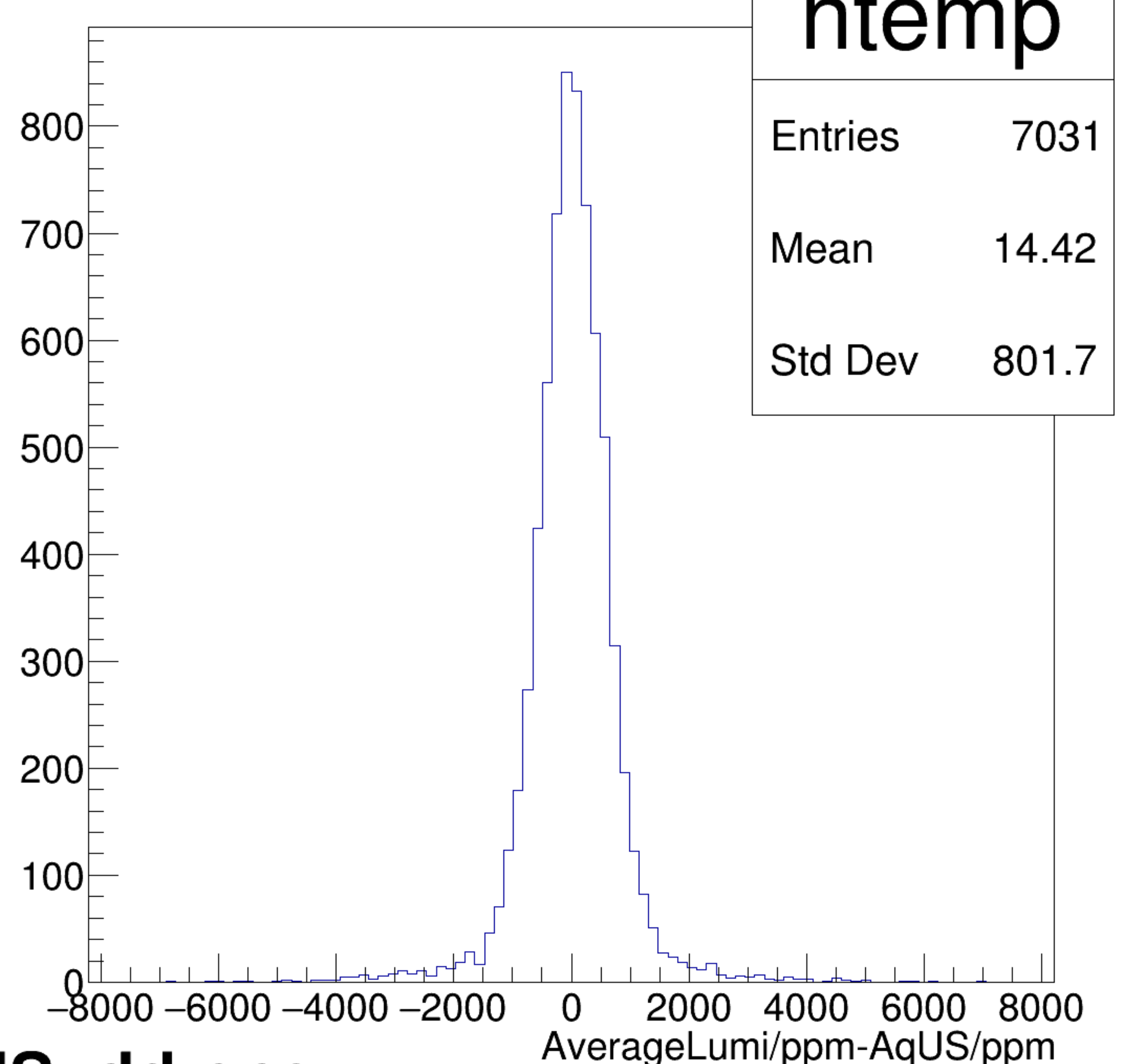
AverageLumi/ppm-AqUS/ppm {ErrorFlag==0}
