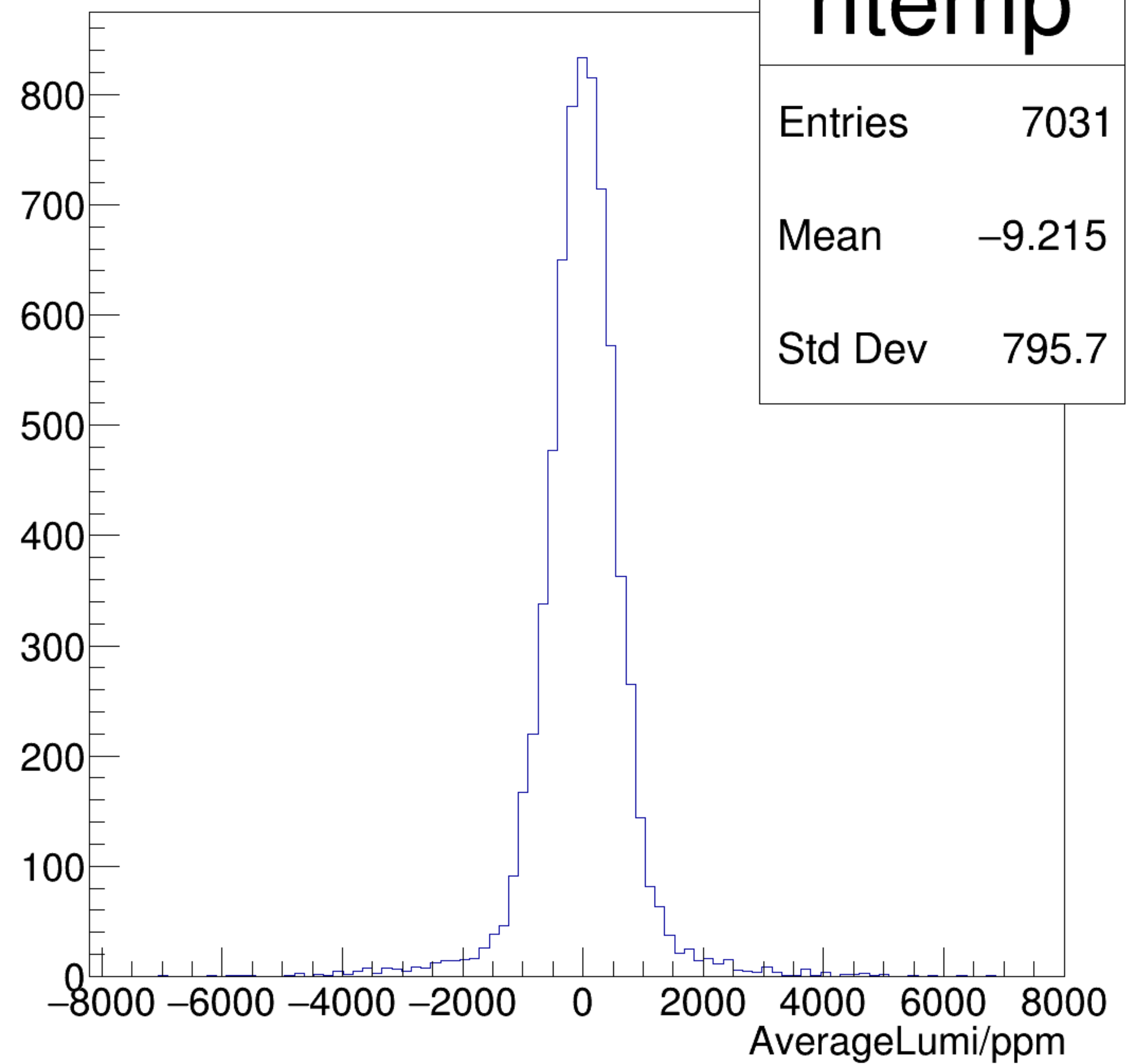
AverageLumi/ppm {ErrorFlag==0}
