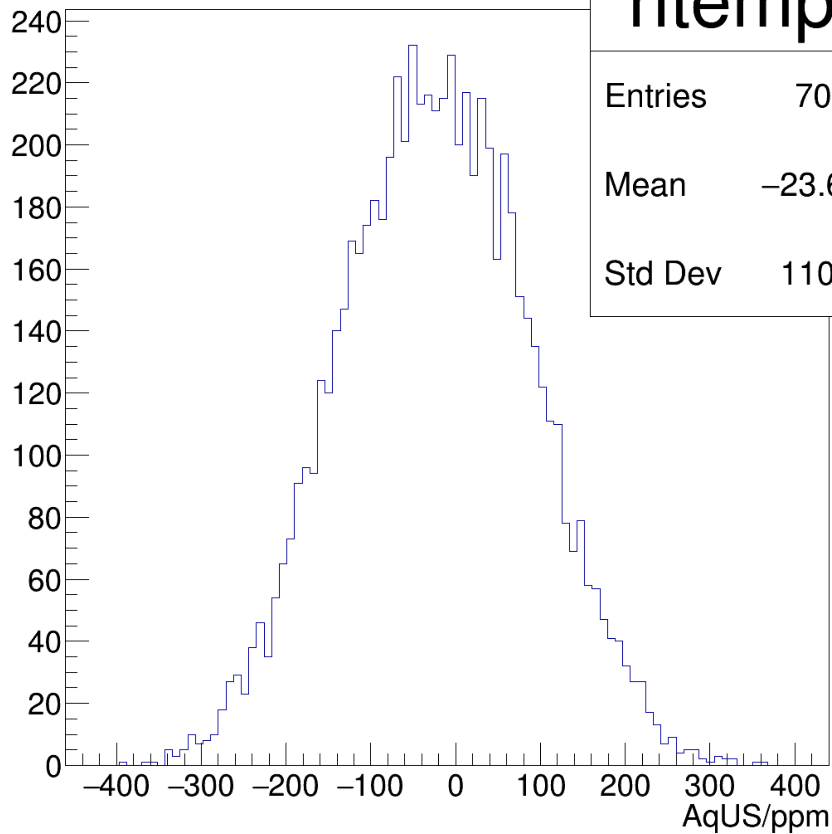
AqUS/ppm {ErrorFlag==0}
