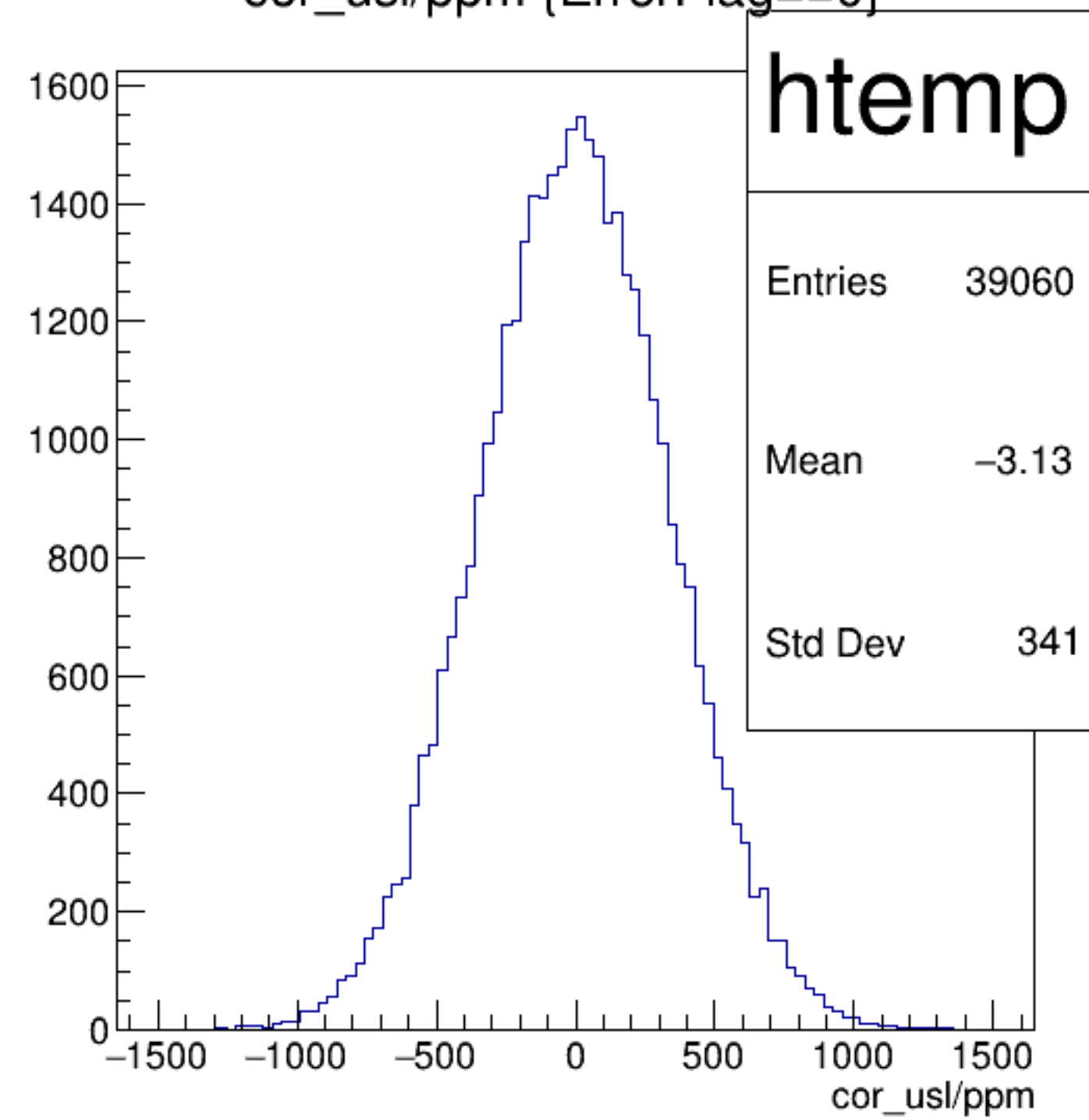
cor_usl/ppm {ErrorFlag==0}
