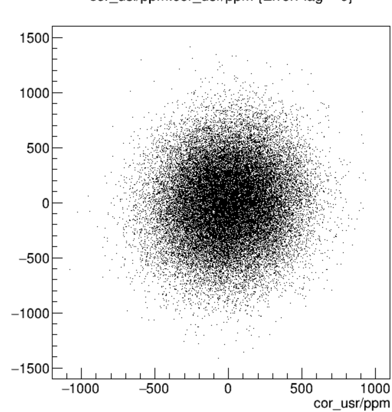
cor_usl/ppm:cor_usr/ppm {ErrorFlag==0}
