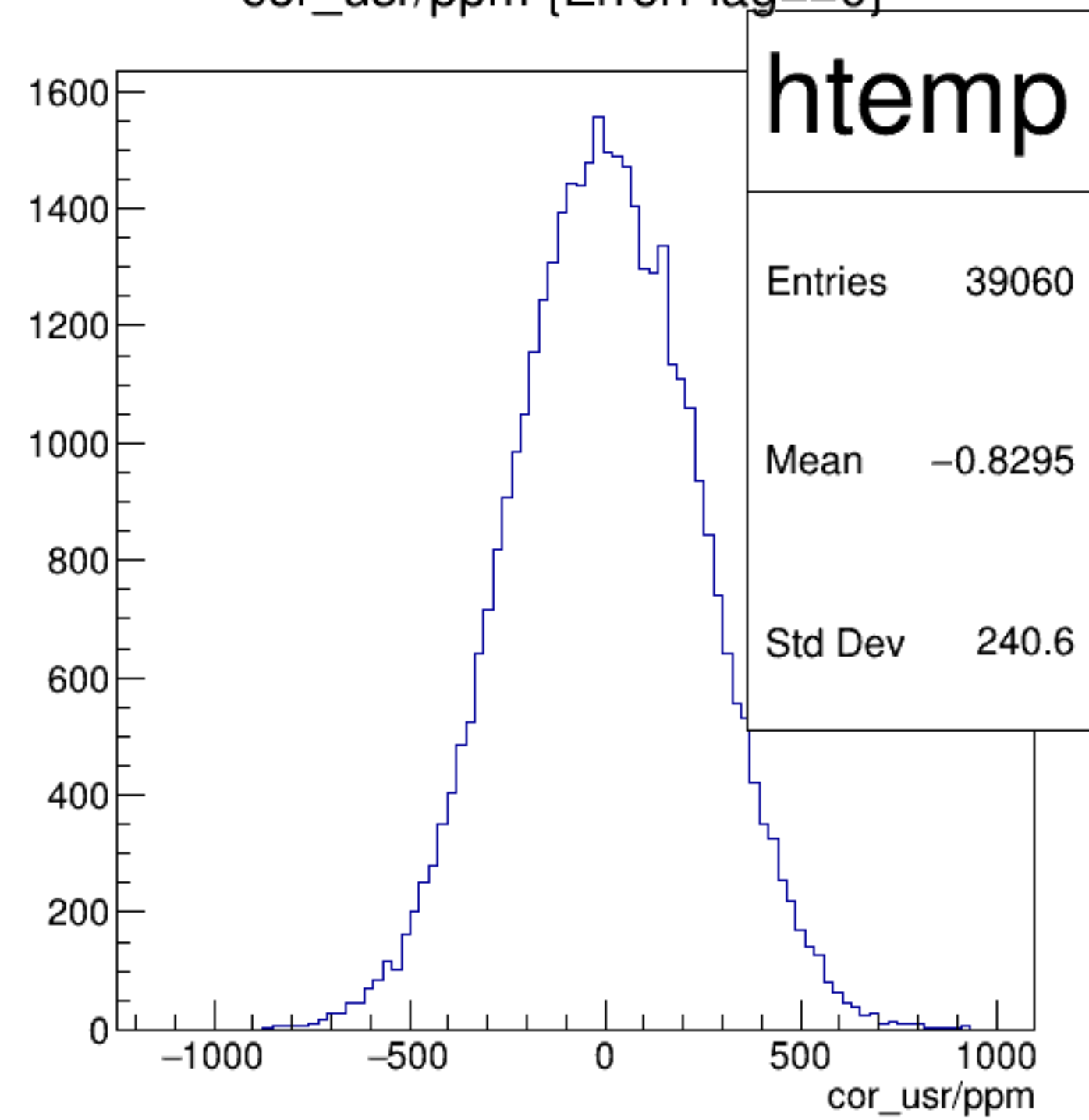
cor_usr/ppm {ErrorFlag==0}
