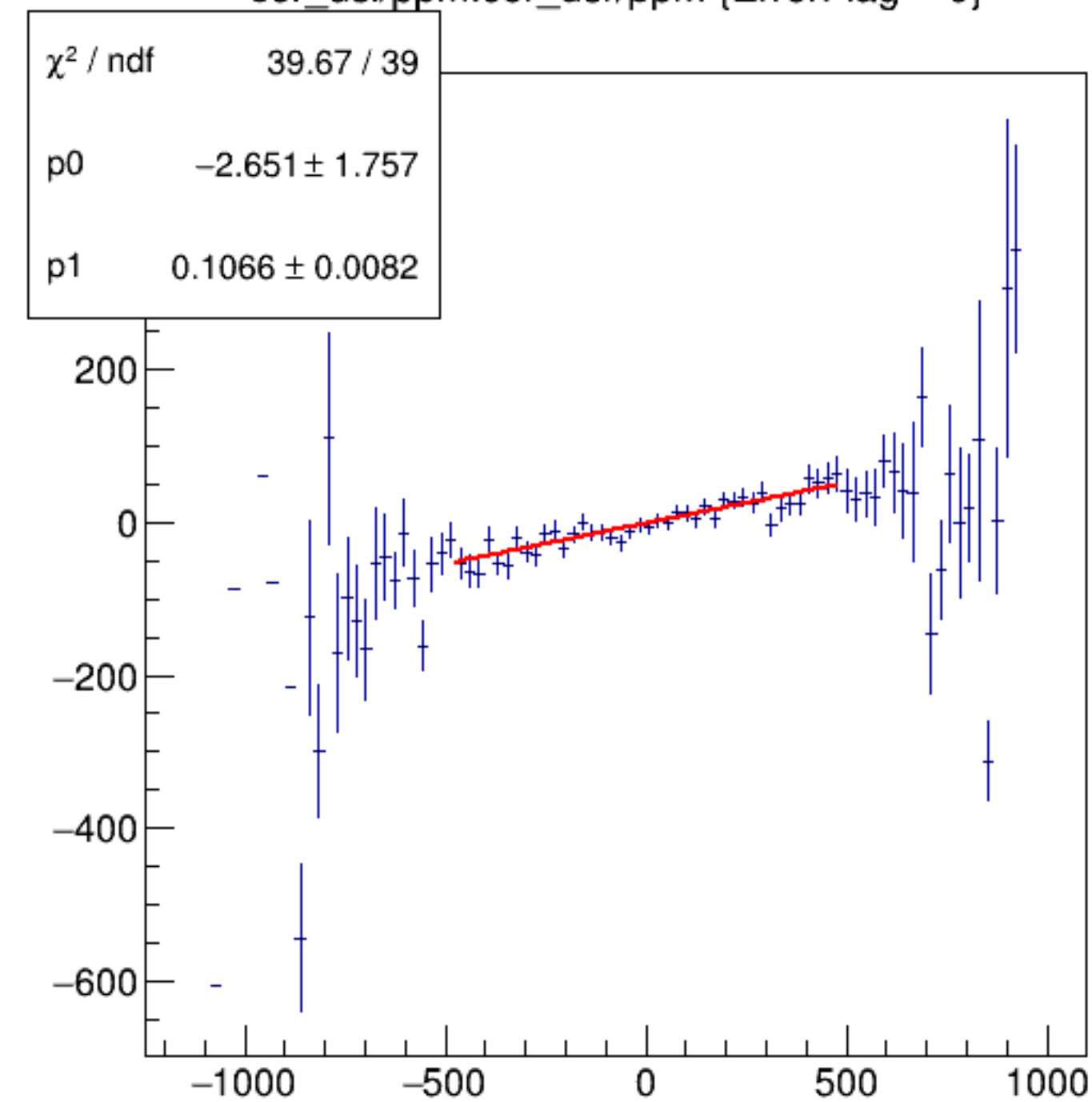
cor_usl/ppm:cor_usr/ppm {ErrorFlag==0}
