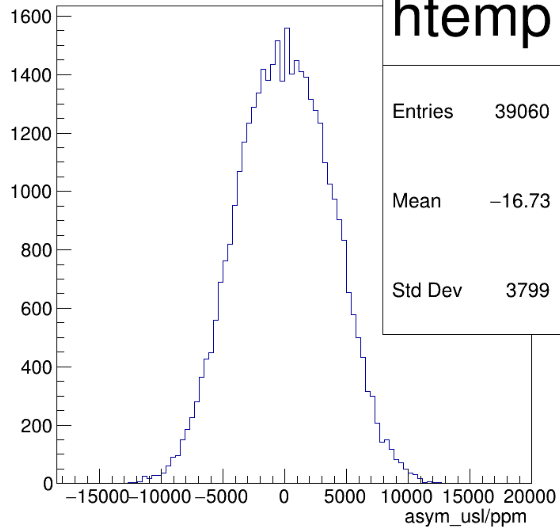
asym_usl/ppm {ErrorFlag==0}
