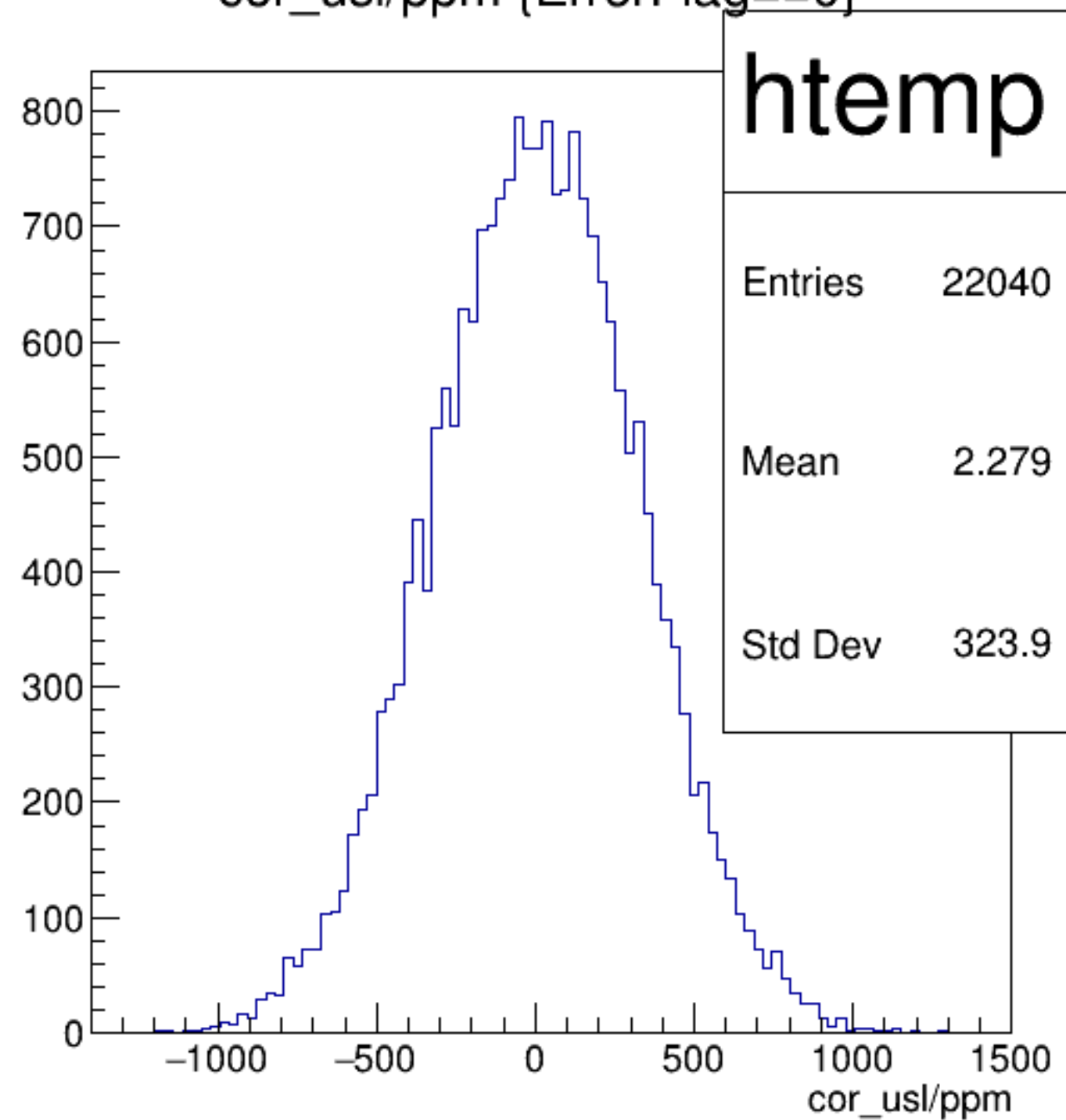
cor_usl/ppm {ErrorFlag==0}
