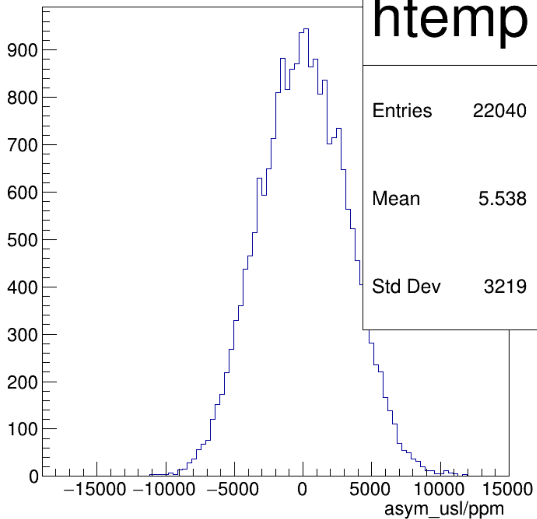
asym_usl/ppm {ErrorFlag==0}
