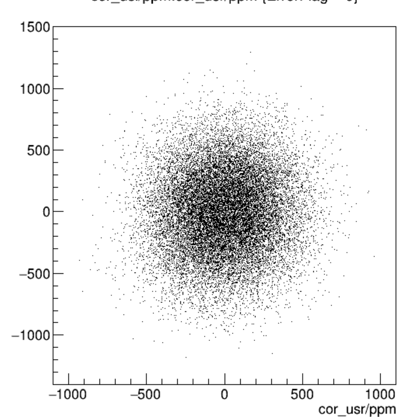
cor_usl/ppm:cor_usr/ppm {ErrorFlag==0}
