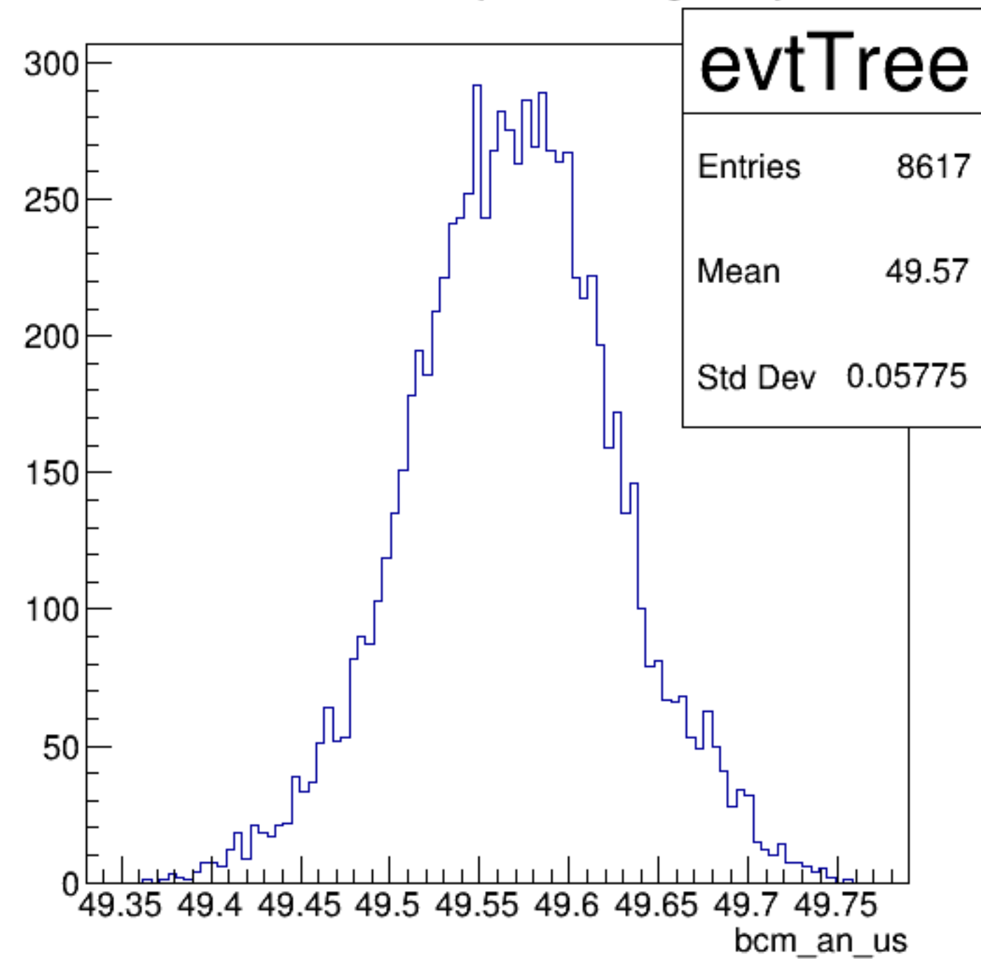
bcm_an_us {ErrorFlag==0}
