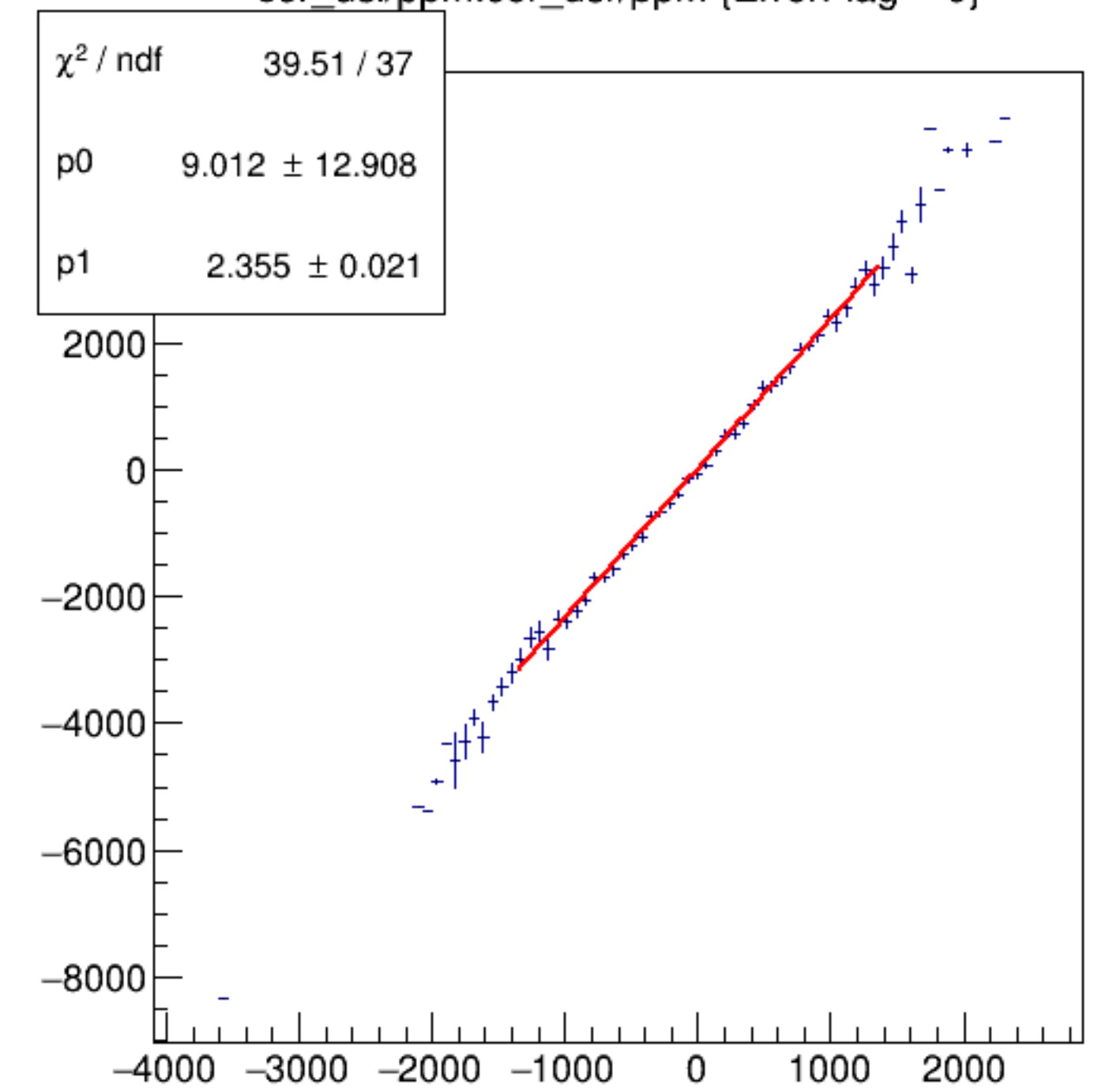
cor_usr/ppm:cor_usr/ppm {ErrorFlag==0}
