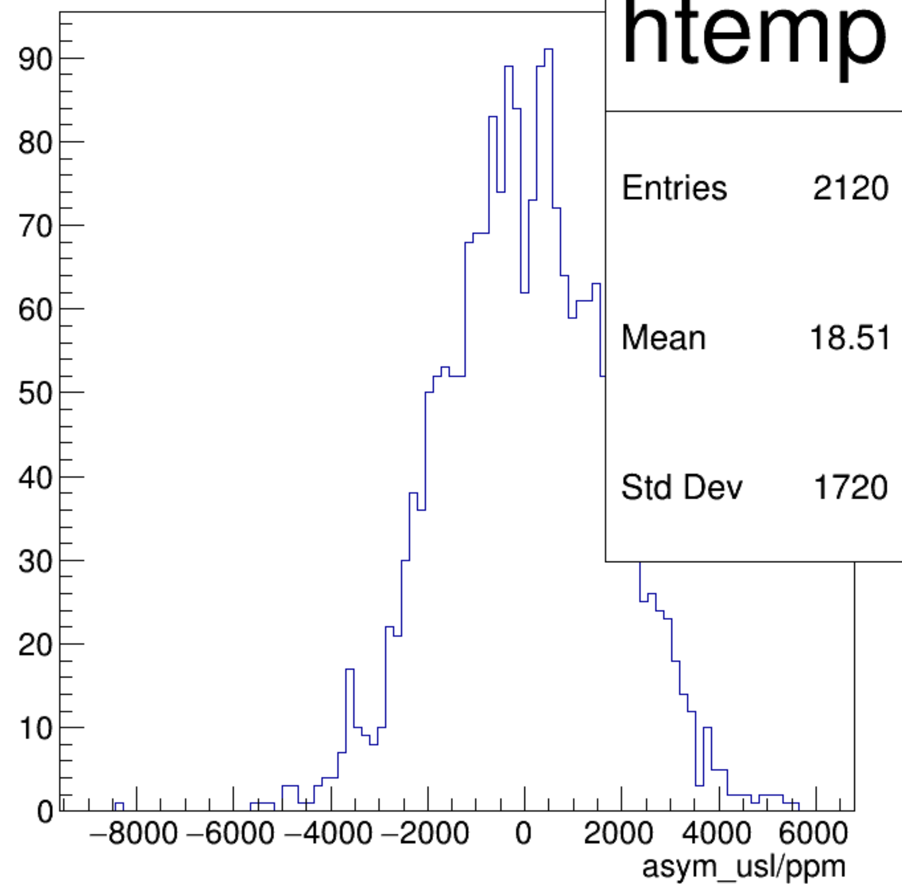
asym_usl/ppm {ErrorFlag==0}
