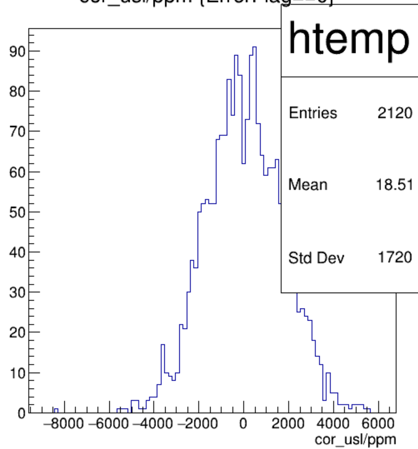
cor_usr/ppm {ErrorFlag==0}
