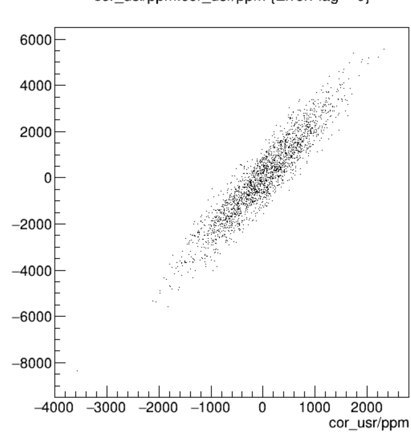
cor_usr/ppm:cor_usr/ppm {ErrorFlag==0}
