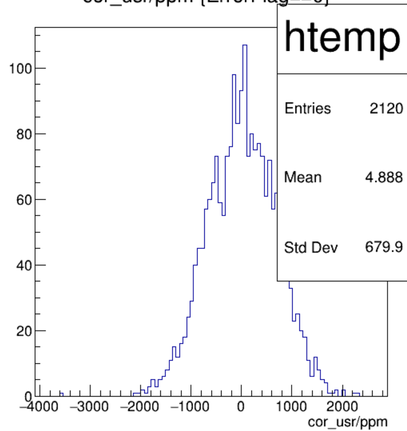
cor_usr/ppm {ErrorFlag==0}
