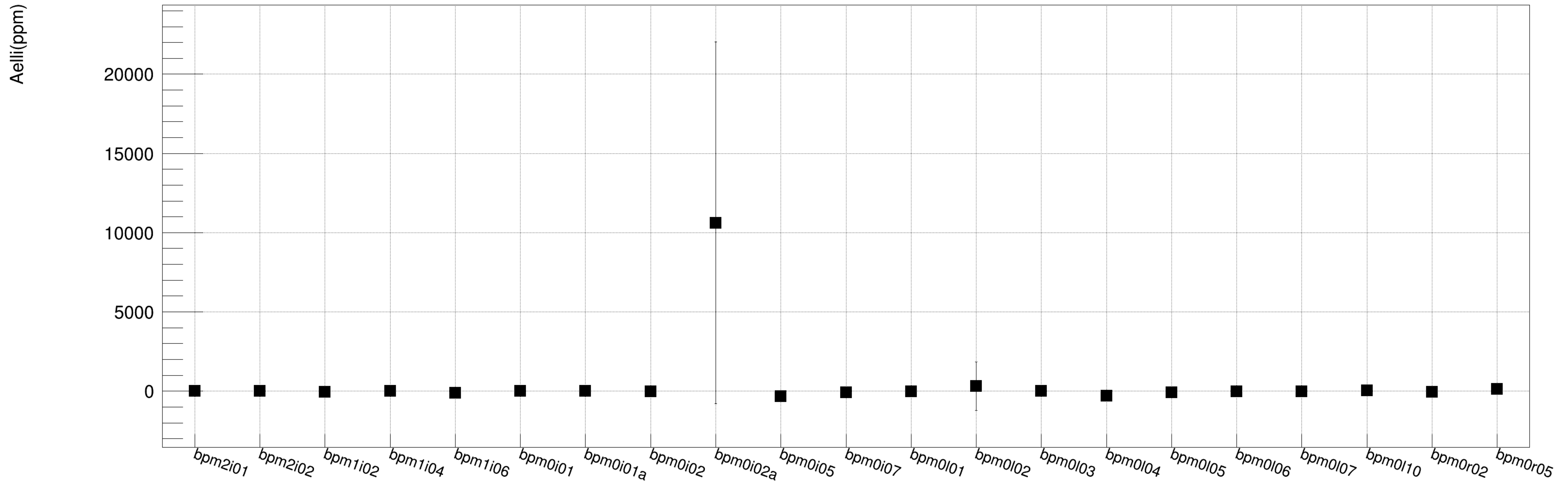
IHWP=1, ErrorFlag==0
