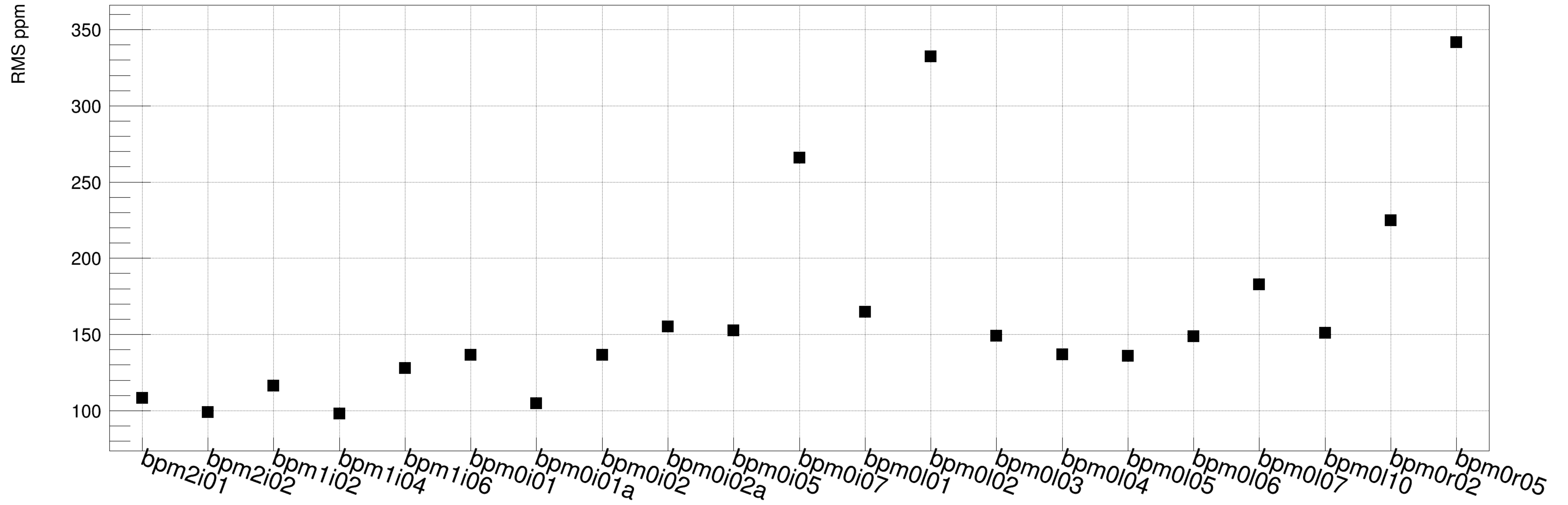
IHWP=1, ErrorFlag==0
