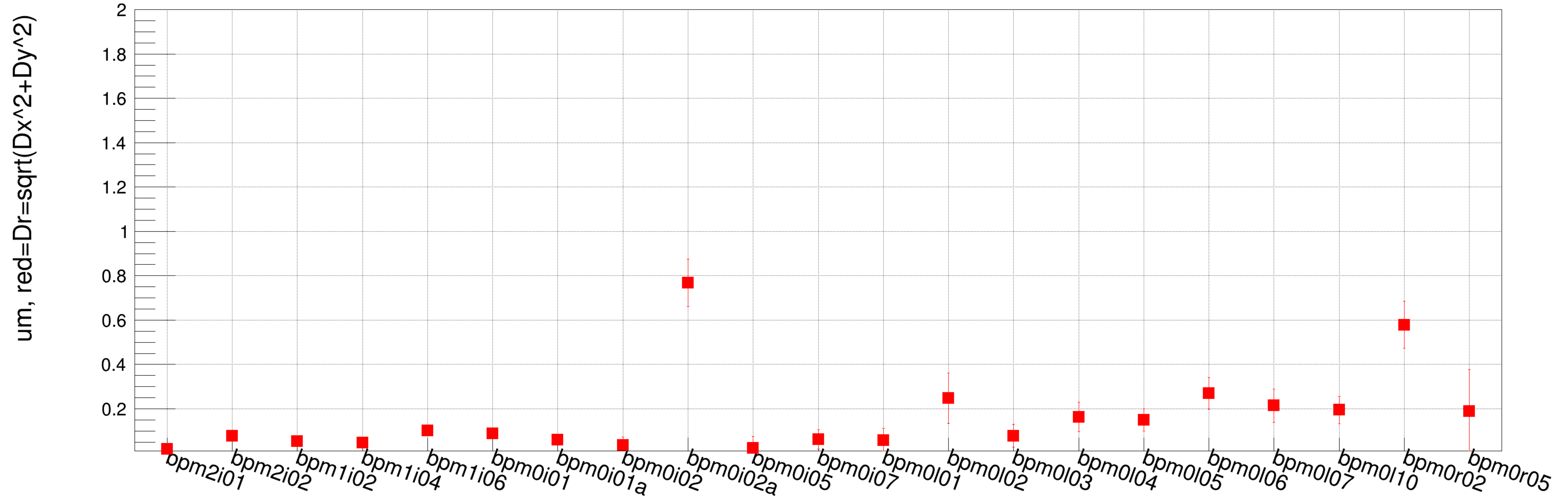
IHWP=1, ErrorFlag==0
