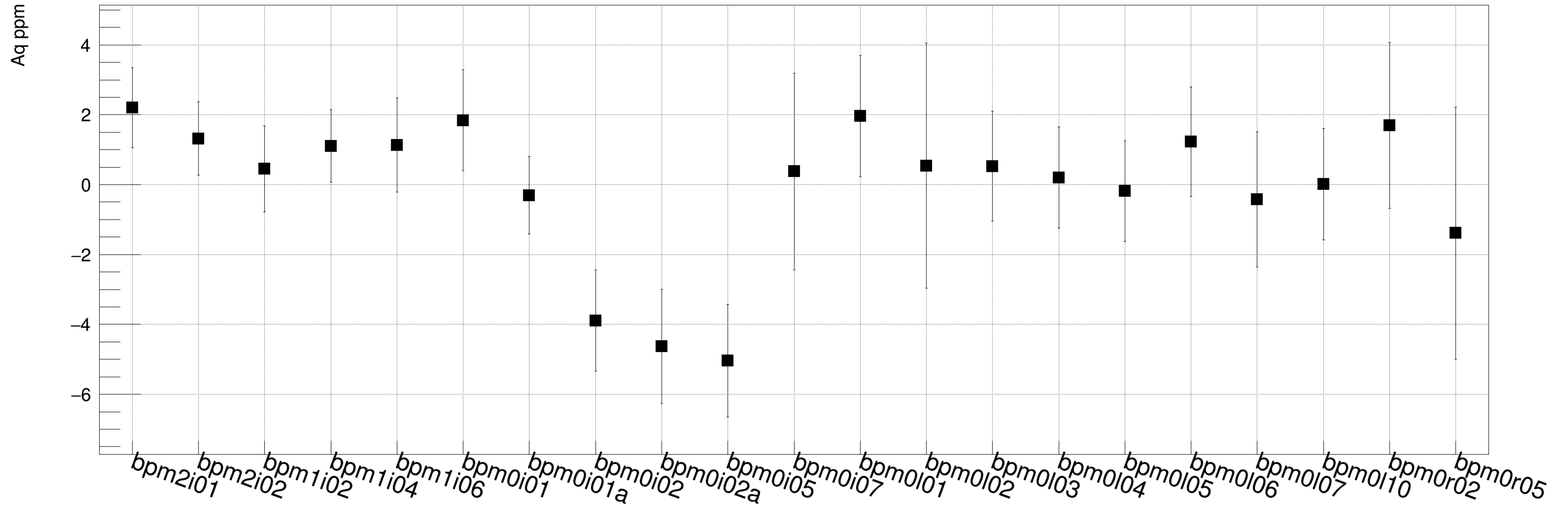
IHWP=1, ErrorFlag==0
