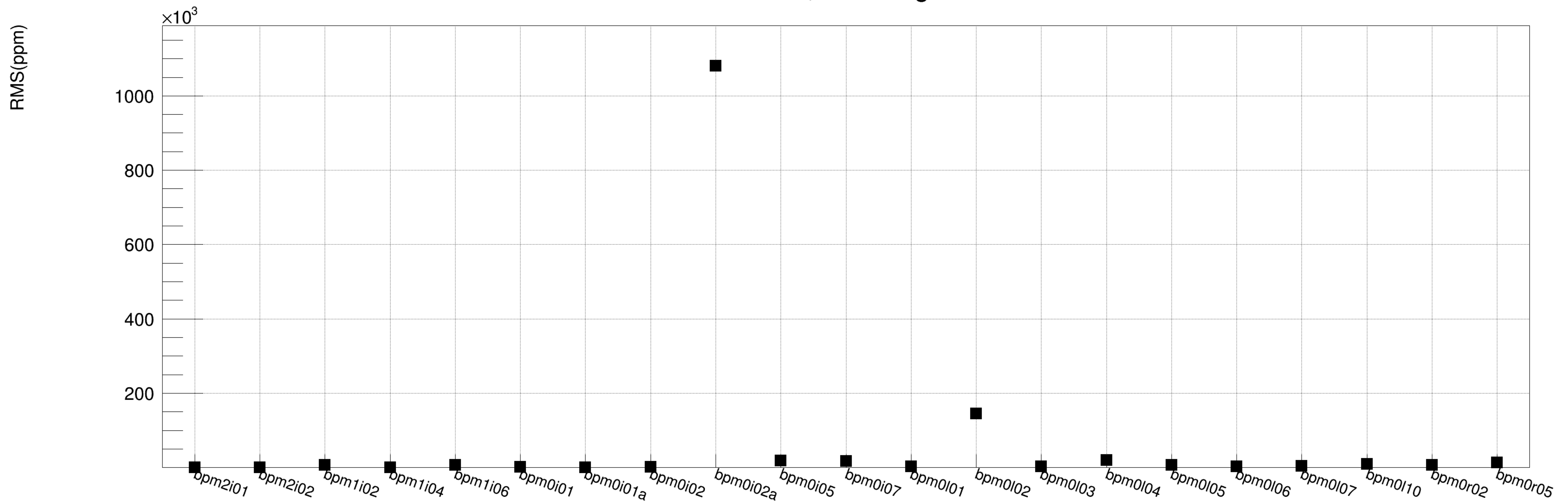
IHWP=1, ErrorFlag==0
