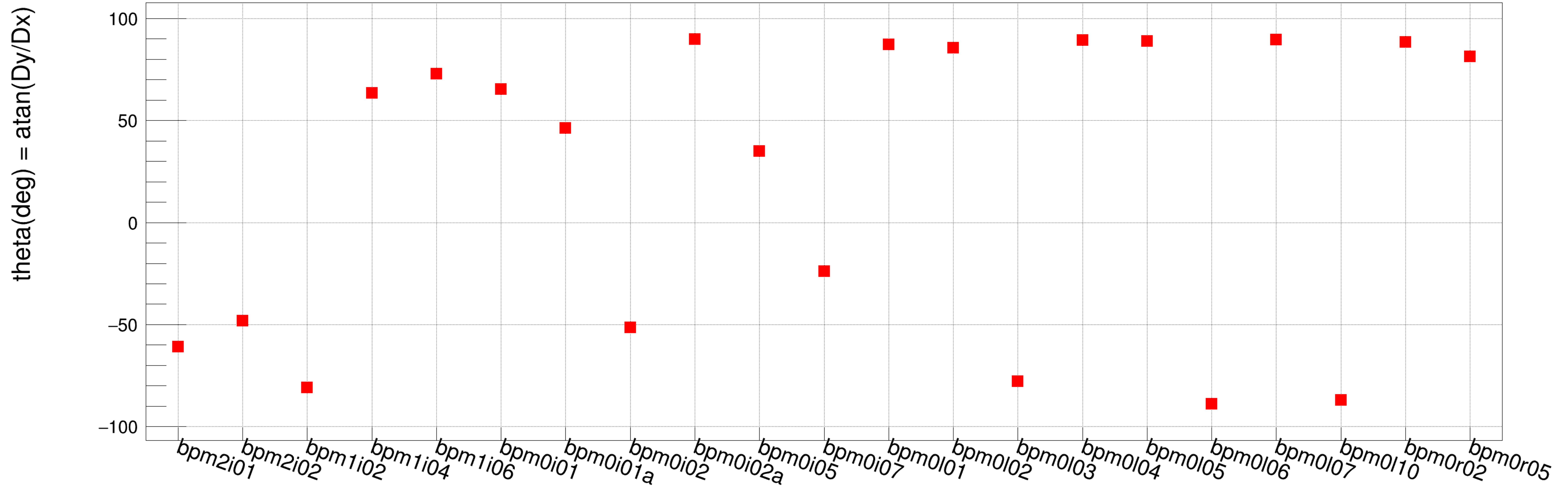
IHWP=1, ErrorFlag==0
