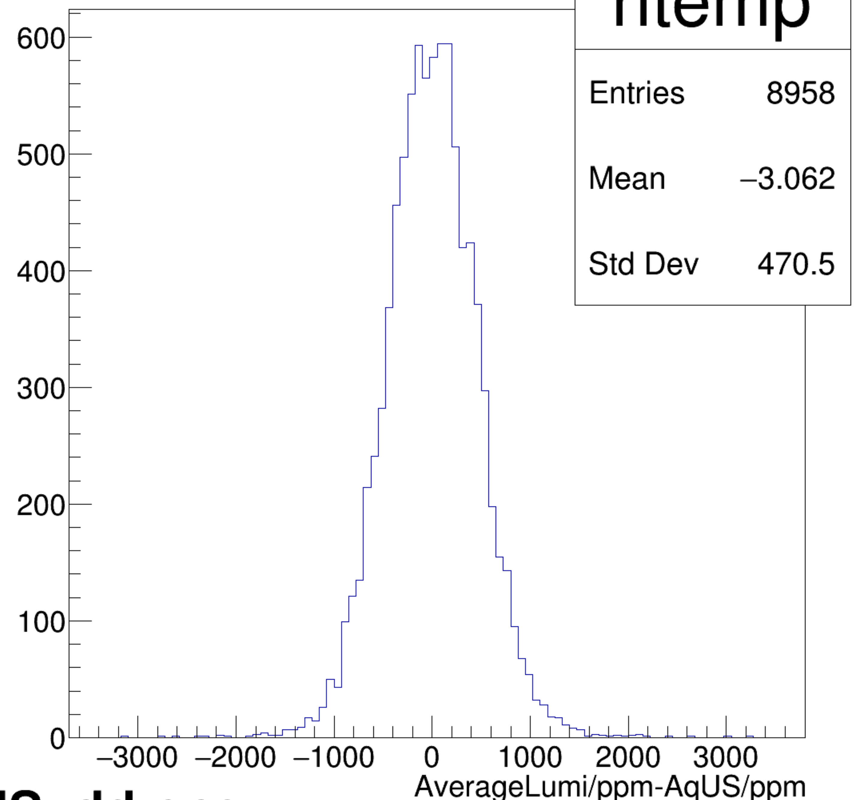
AverageLumi/ppm-AqUS/ppm {ErrorFlag==0}
