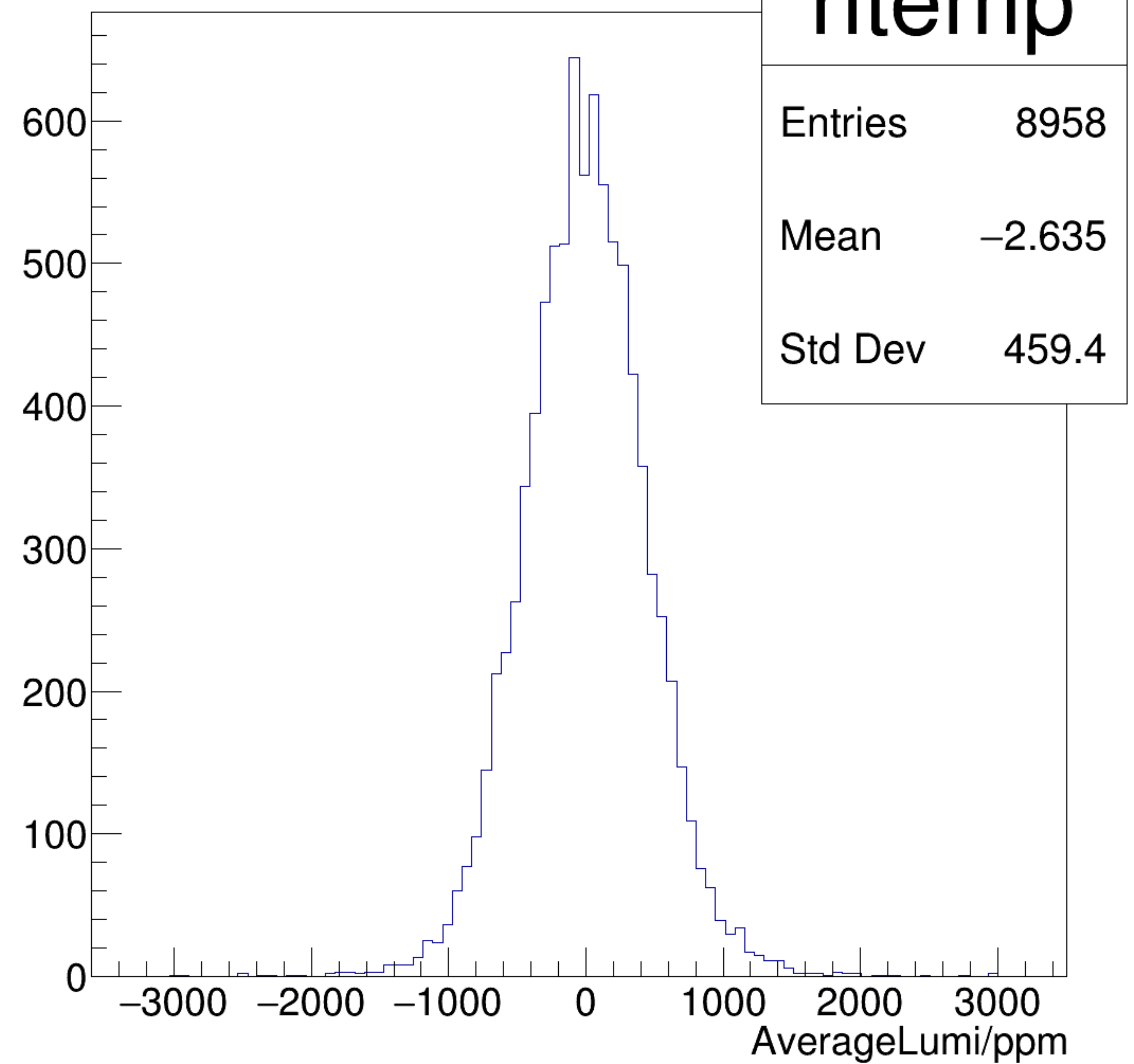
AverageLumi/ppm {ErrorFlag==0}
