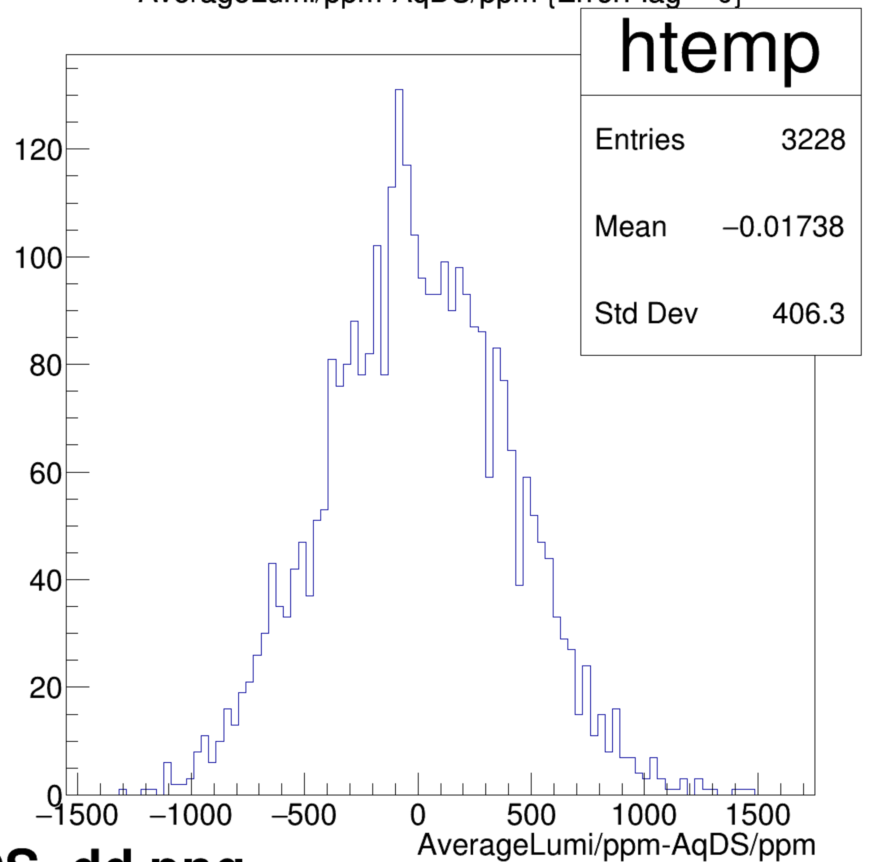
AverageLumi/ppm-AqDS/ppm {ErrorFlag==0}
