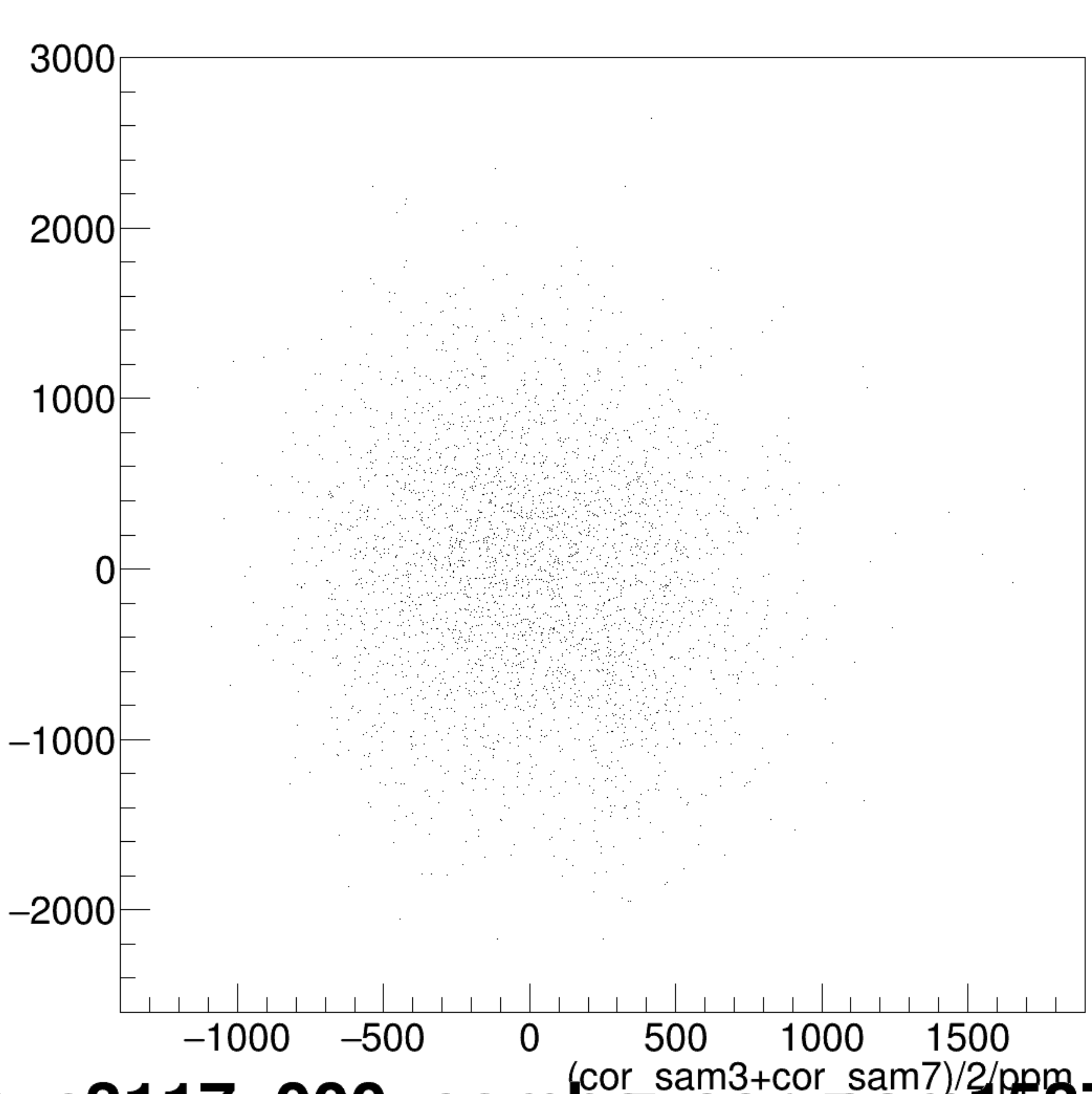
(cor_sam1+cor_sam5)/2/ppm:(cor_sam3+cor_sam7)/2/ppm {ErrorFlag==0}
