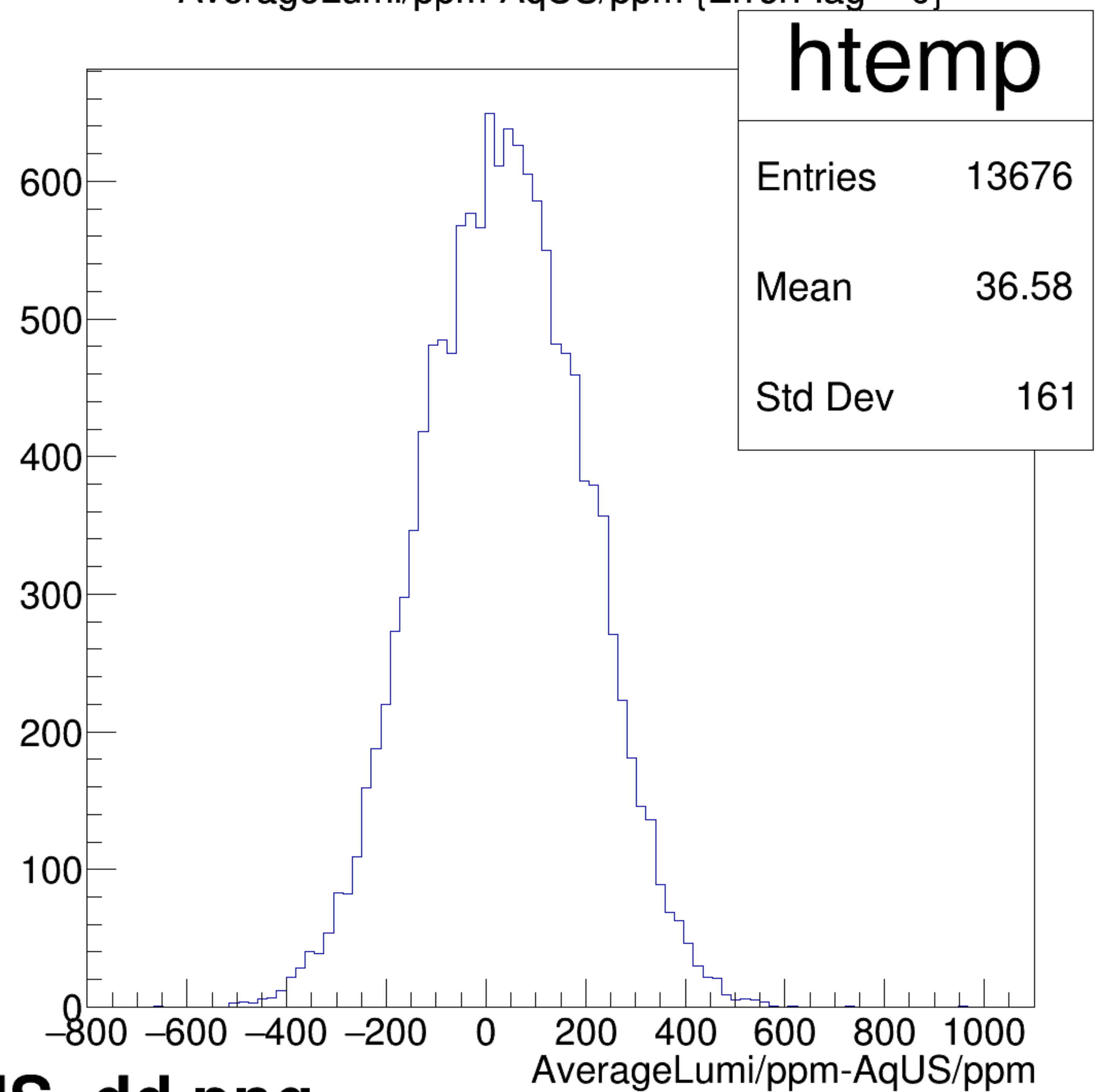
AverageLumi/ppm-AqUS/ppm {ErrorFlag==0}
