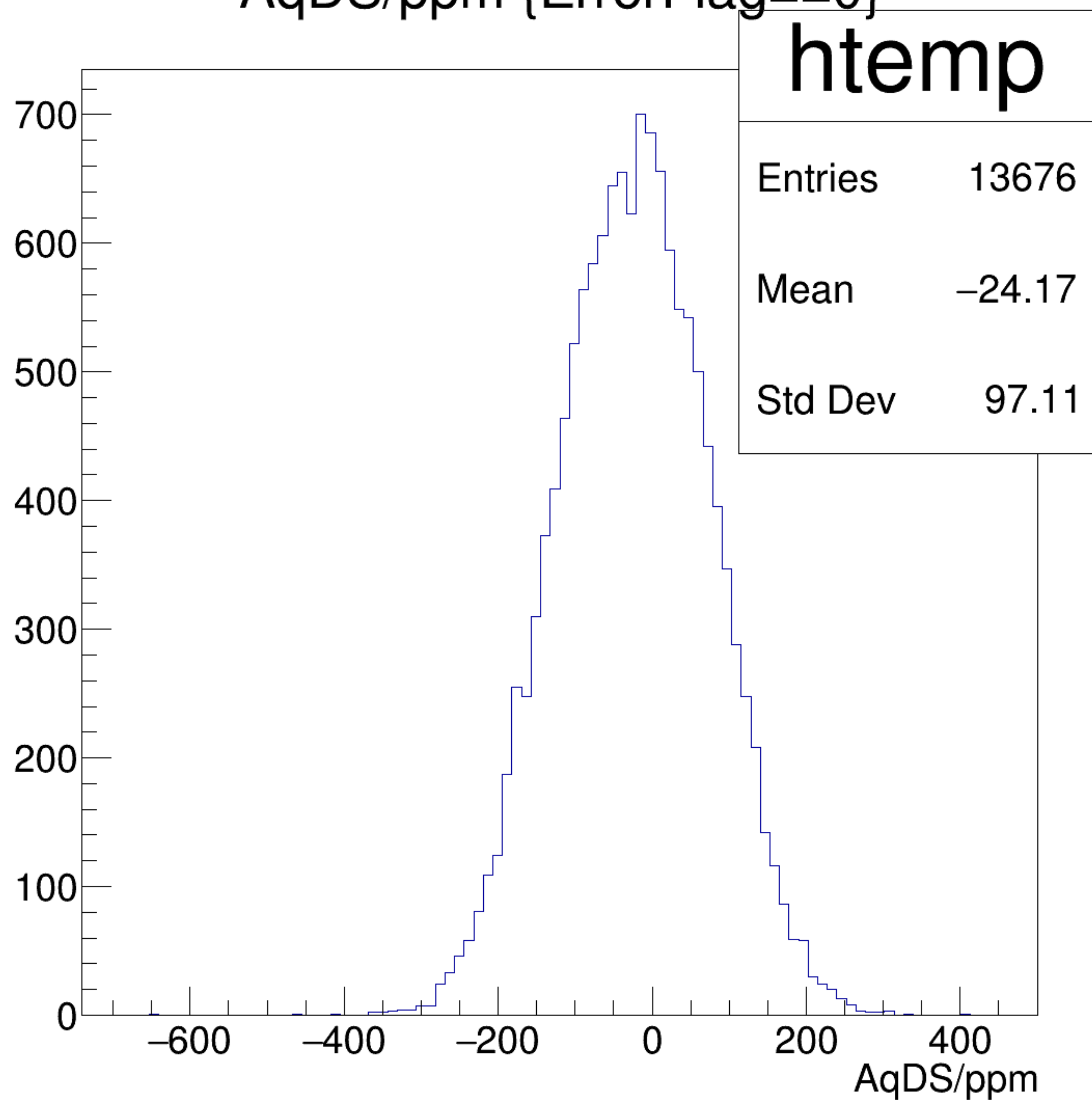
AqDS/ppm {ErrorFlag==0}
