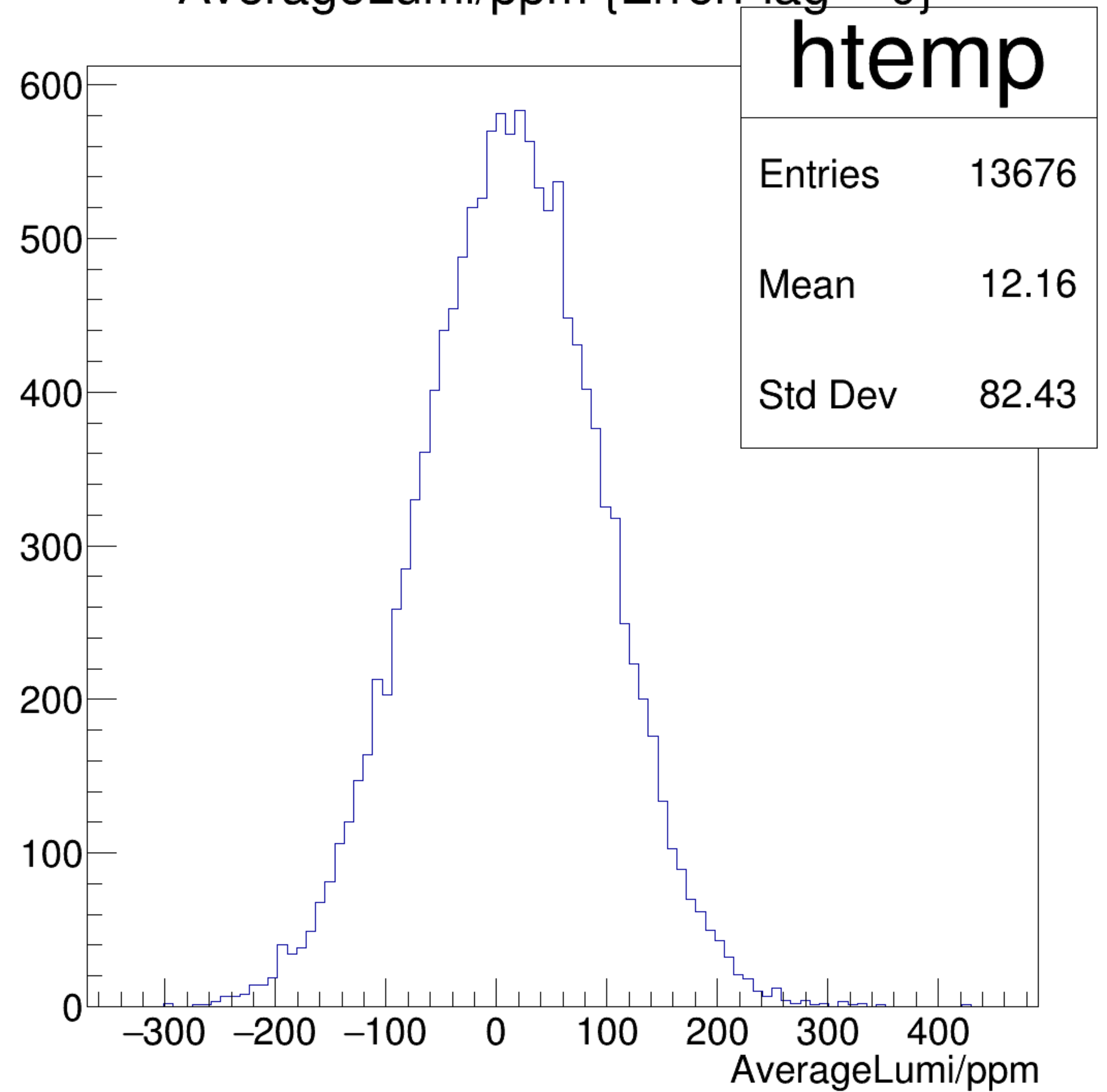
AverageLumi/ppm {ErrorFlag==0}
