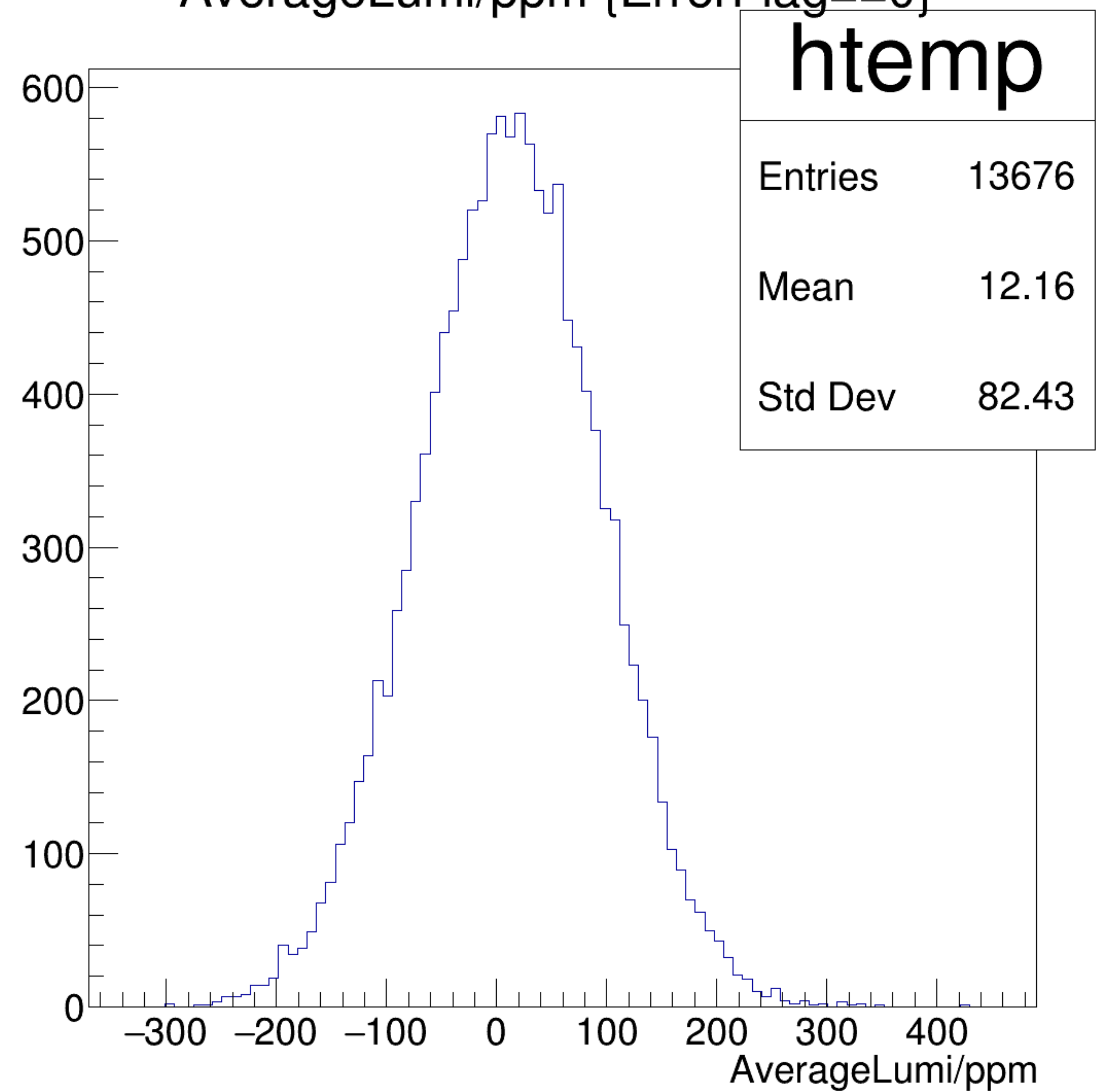
AverageLumi/ppm {ErrorFlag==0}
