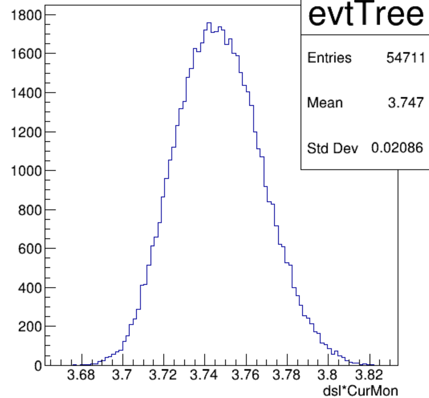
dsl*CurMon {ErrorFlag==0}
