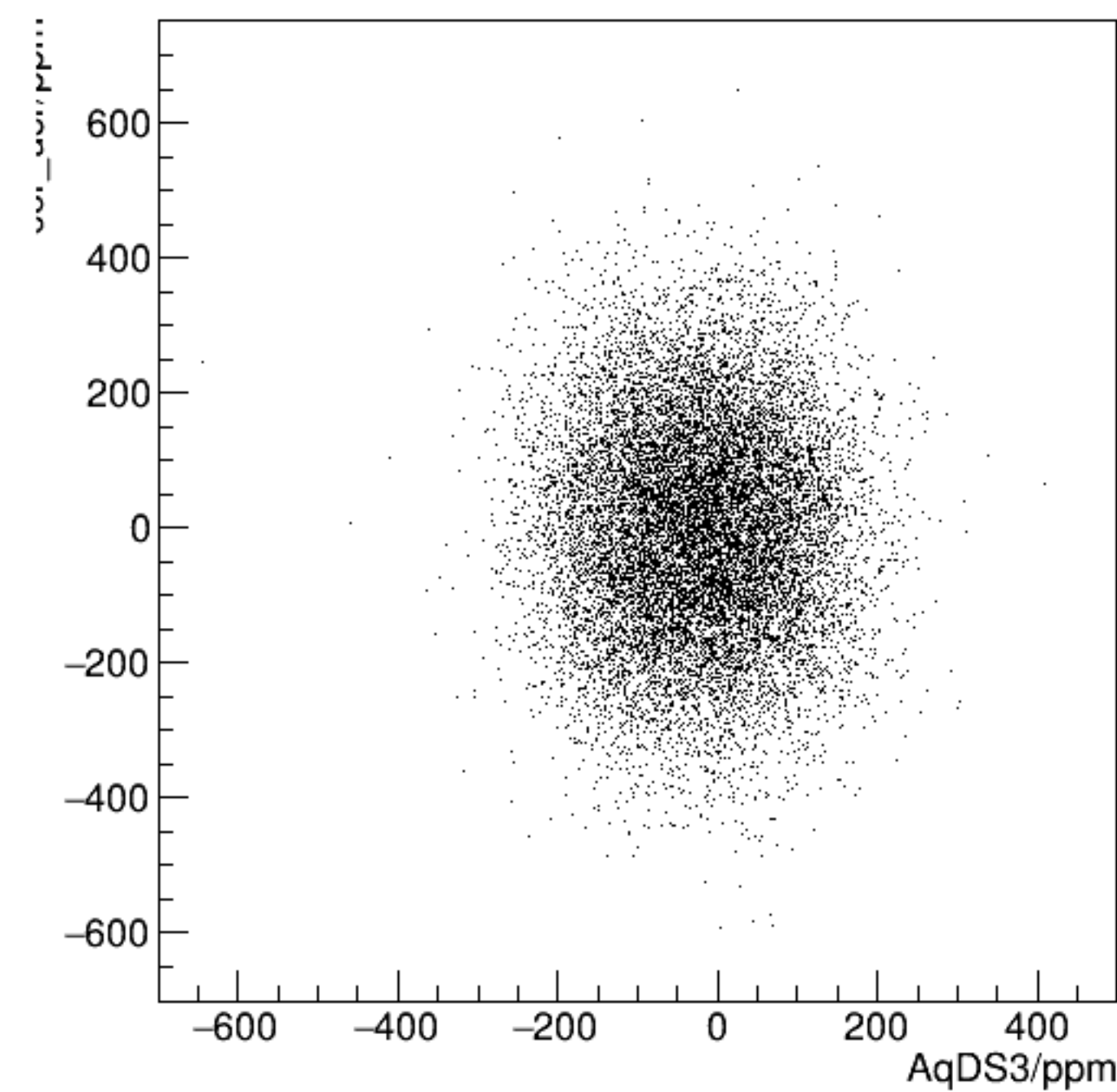
cor_usr/ppm:AqDS3/ppm {ErrorFlag==0}
