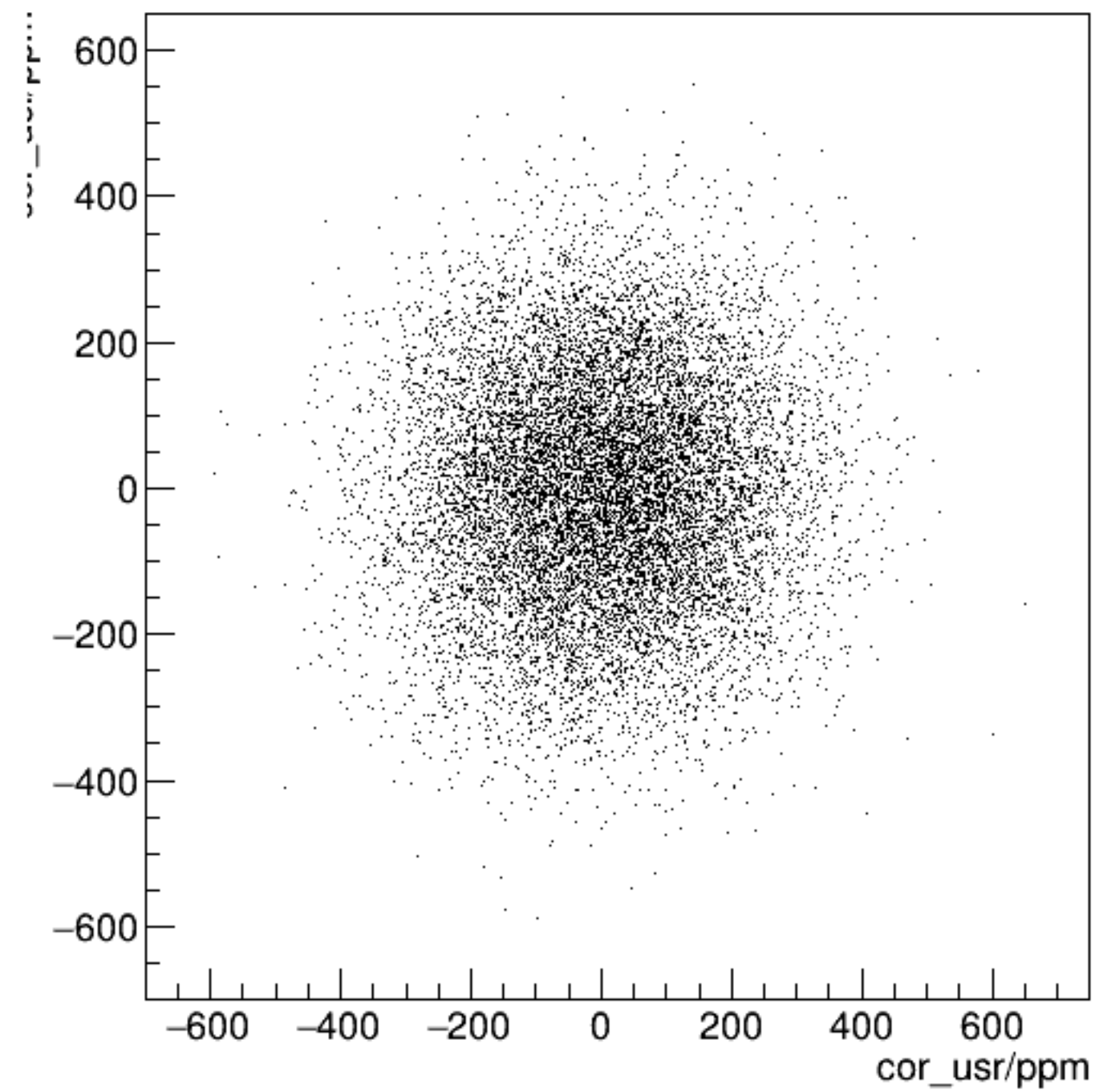
cor_usl/ppm:cor_usr/ppm {ErrorFlag==0}
