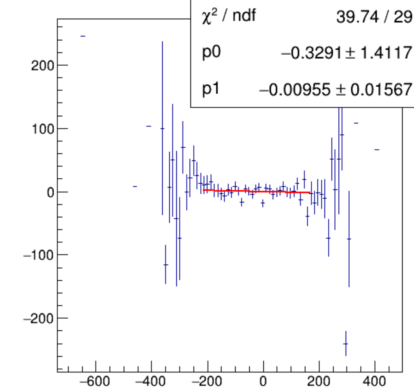
cor_usr/ppm:AqDS3/ppm {ErrorFlag==0}
