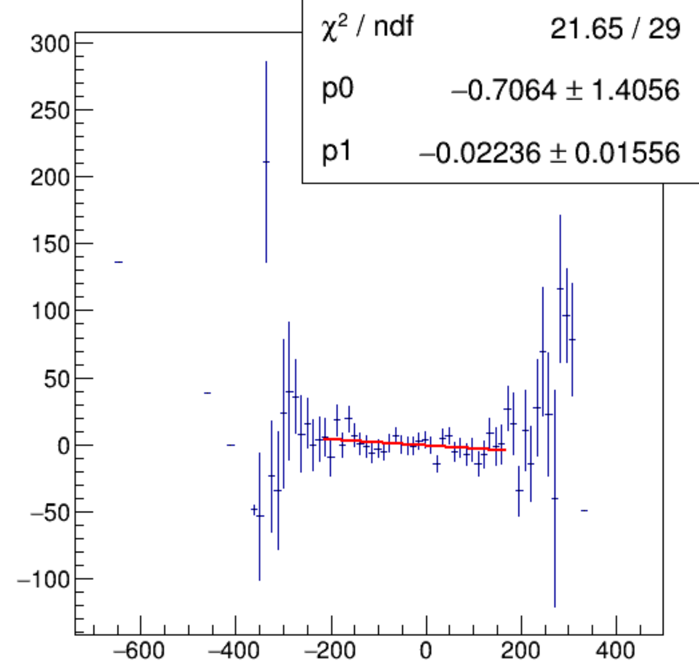
cor_usr/ppm:AqDS3/ppm {ErrorFlag==0}
