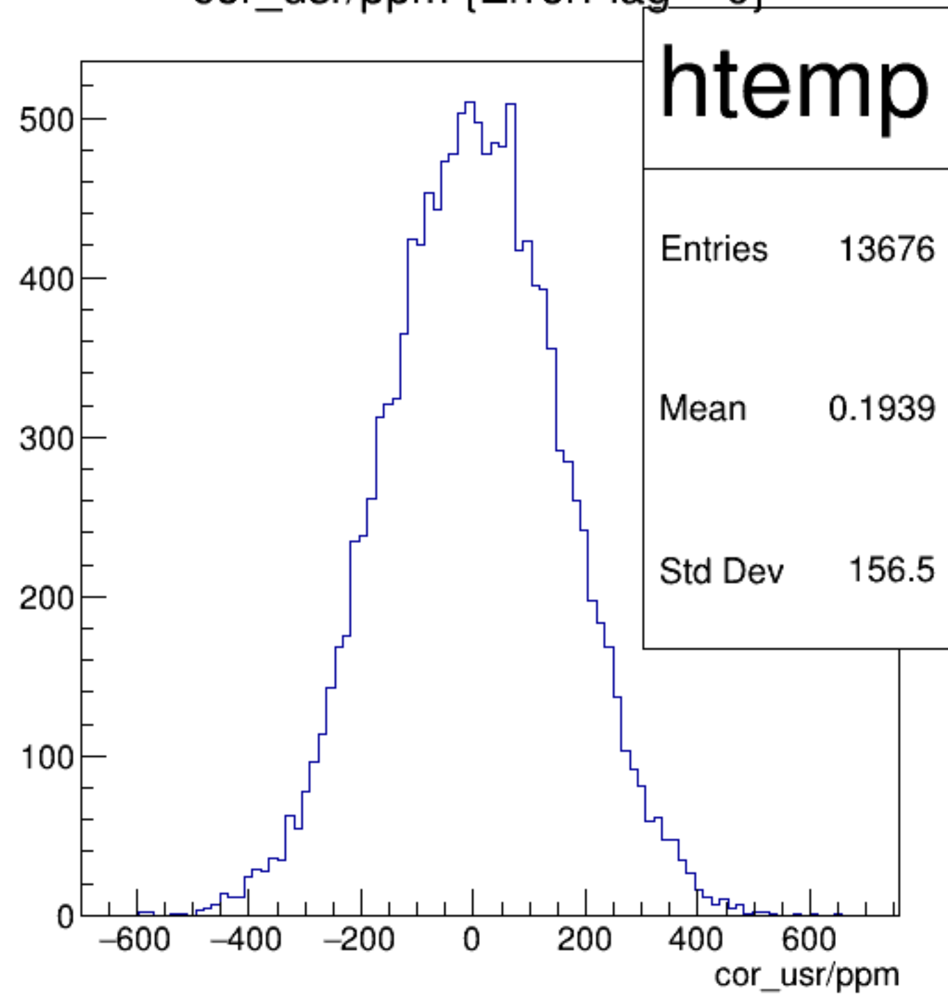
cor_usr/ppm {ErrorFlag==0}
