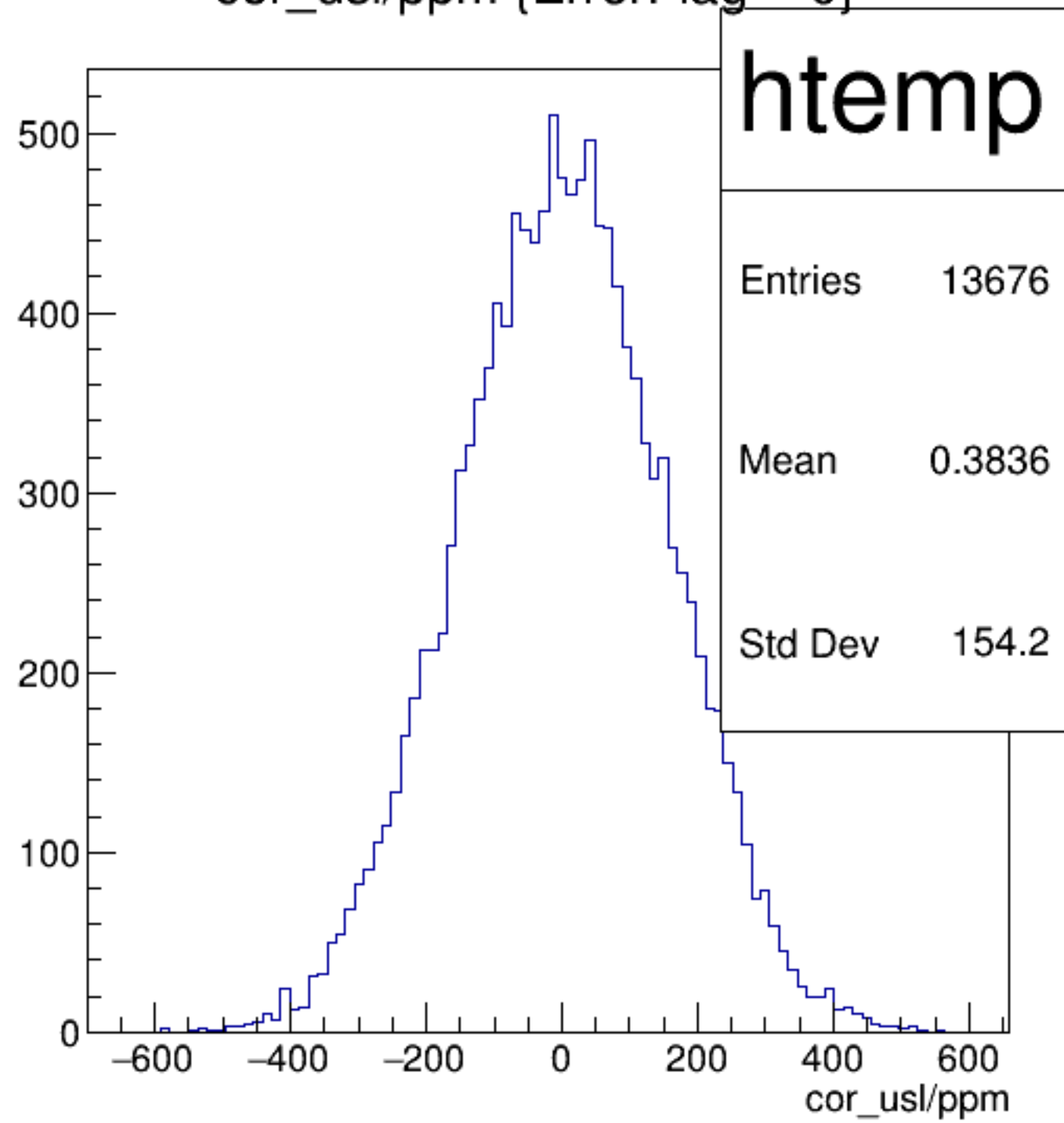
cor_usl/ppm {ErrorFlag==0}
