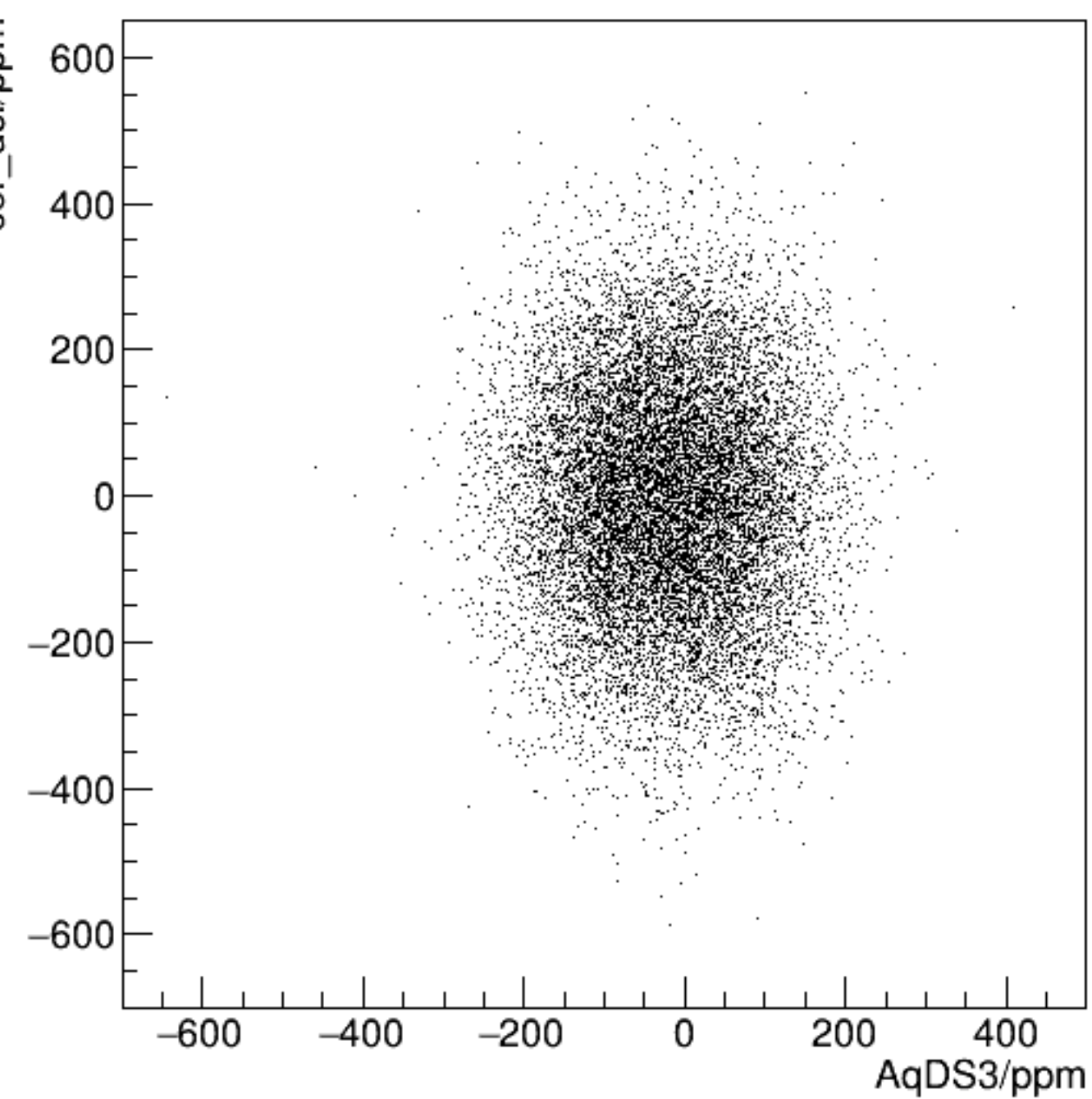
cor_usr/ppm:AqDS3/ppm {ErrorFlag==0}
